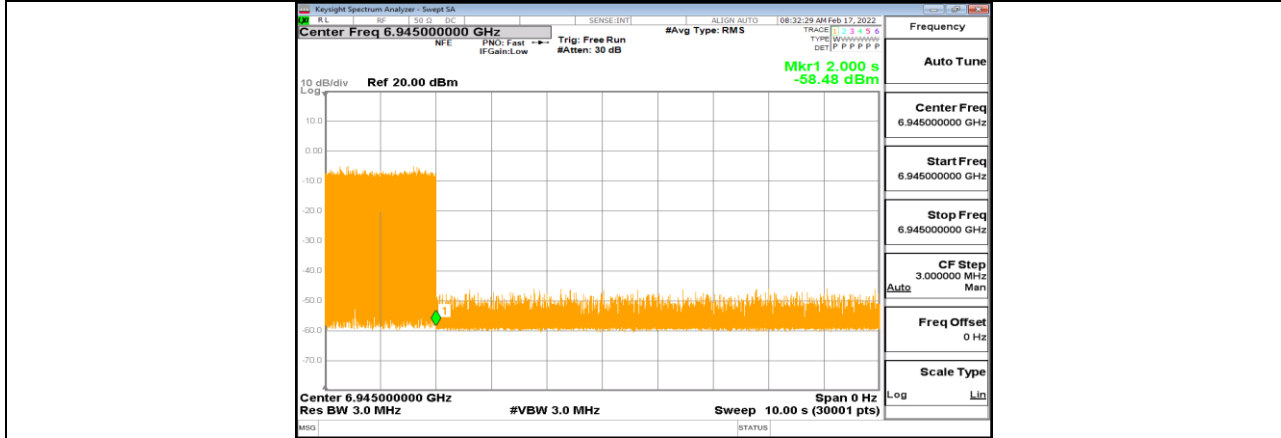
11AX80MIMO_Ant1_6945_Center_6945_9
