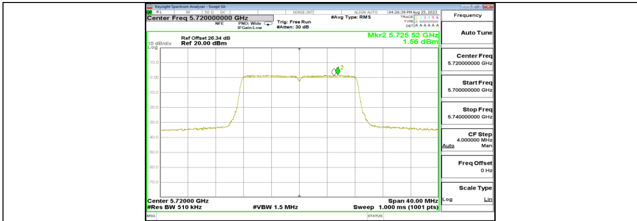
11A_Ant1_5720_UNI1-3
