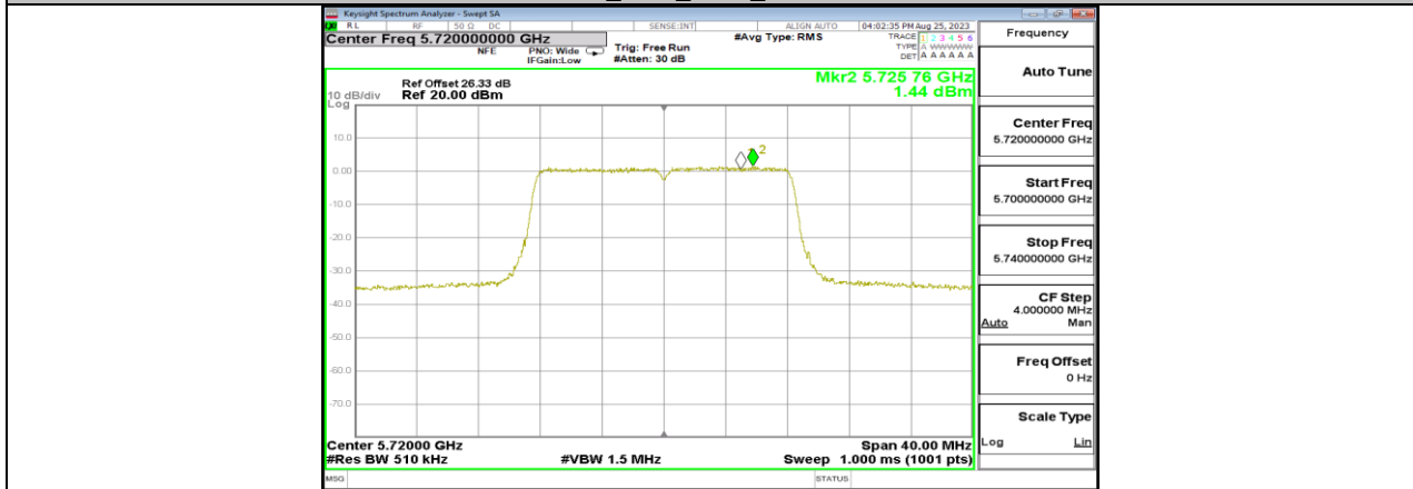
11A_Ant0_5720_UNII-3
