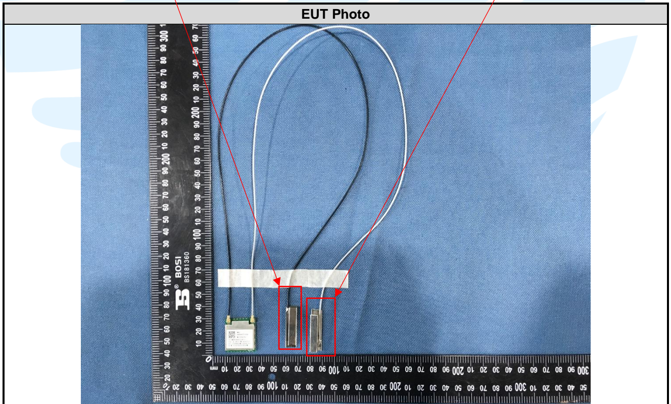
Antenna 0 (BT&WI-FI)
