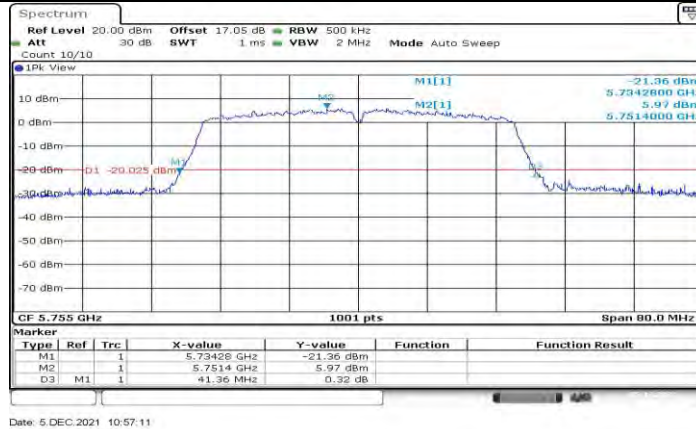
11N40MIMO Ant1 5755
