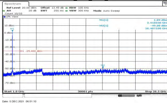
11N20MIMO_Ant1_2412_1000~26500
