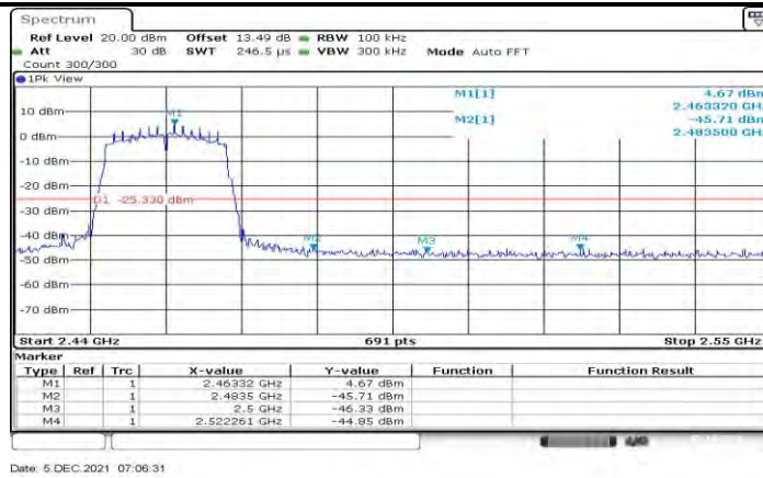
11N20MIMO_Ant1_High_2462
