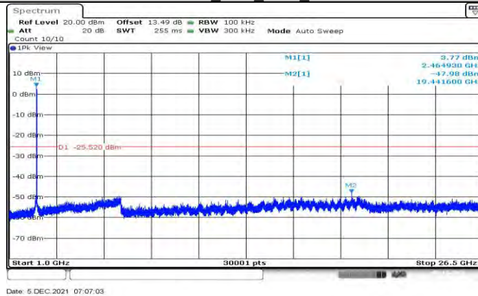
11N20MIMO Ant1 2462 1000~26500
