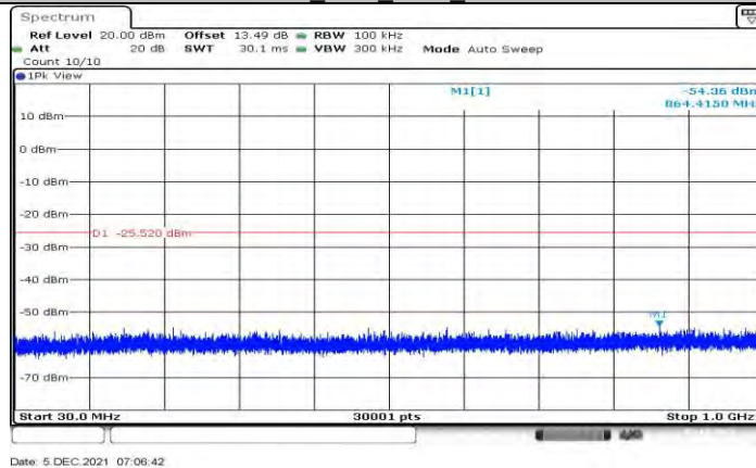
11N20MIMO Ant1 2462 30~1000
