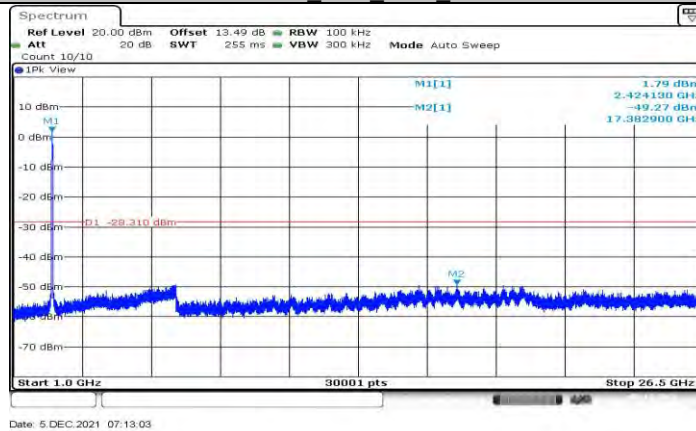
11N40MIMO_Ant1_2422_1000~26500
