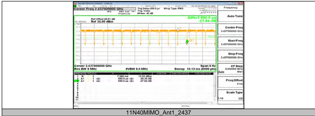
11N40MIMO_Ant1_2437
