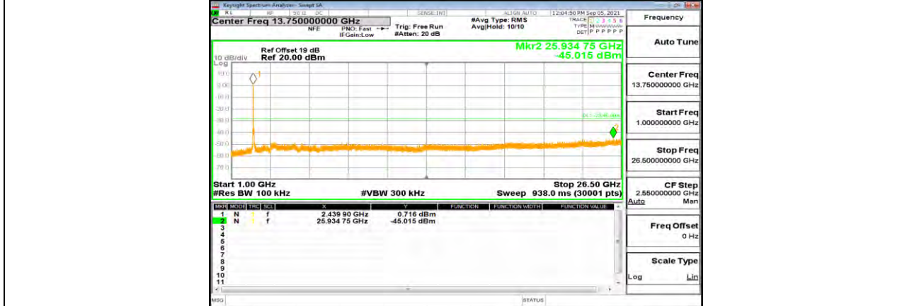
11N40MIMO Ant2 2452 1000~26500
