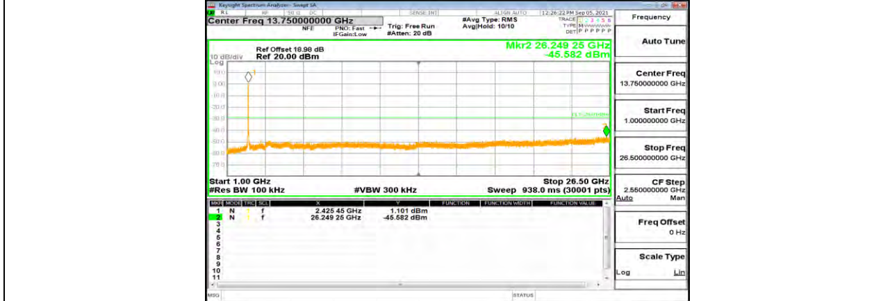
11N40MIMO Ant1 2422 1000~26500
