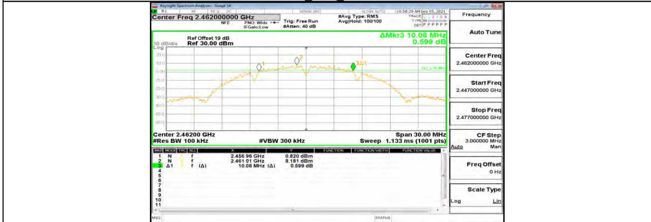
11B Ant2 2462
