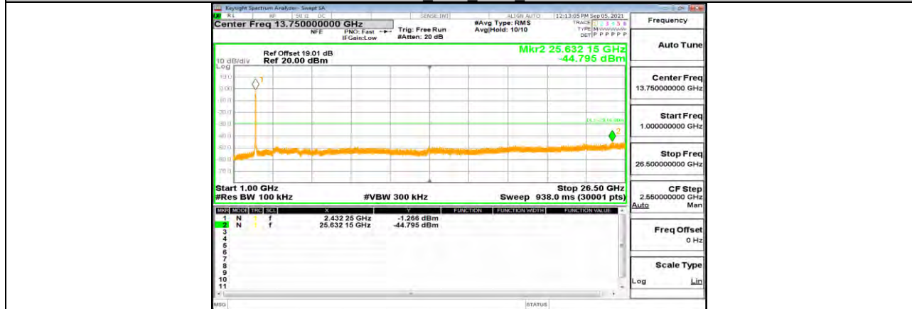
11N40MIMO Ant1 2437 1000~26500
