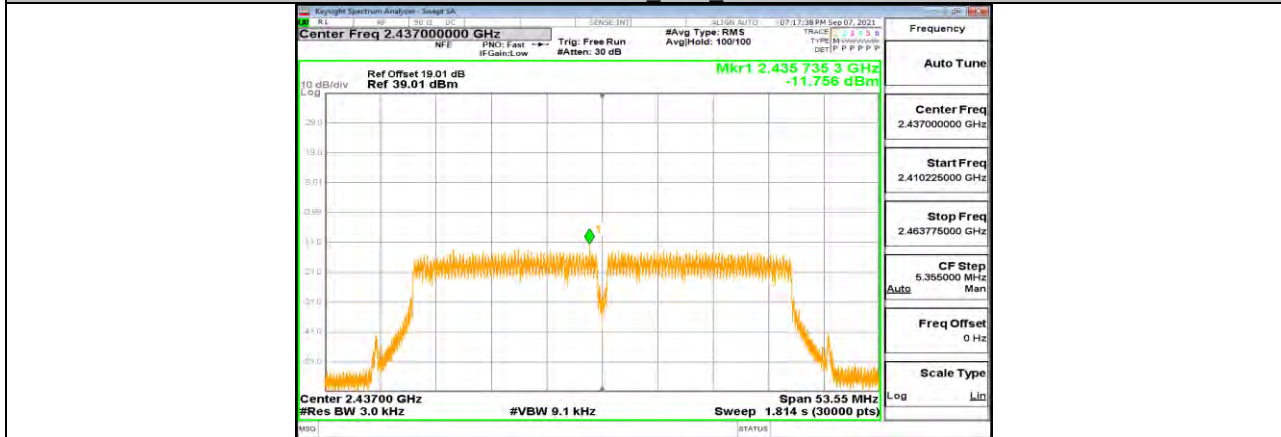
11N40MIMO Ant1 2437
