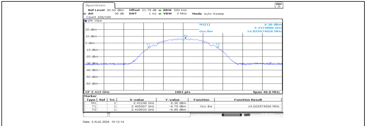
11B_Ant1_2412
