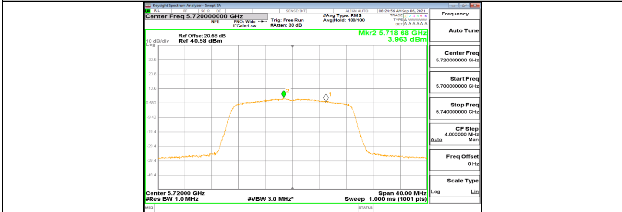
11N20MIMO_Ant2_5720_UHII-2C
