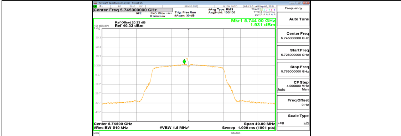
11A_Ant2_5745
