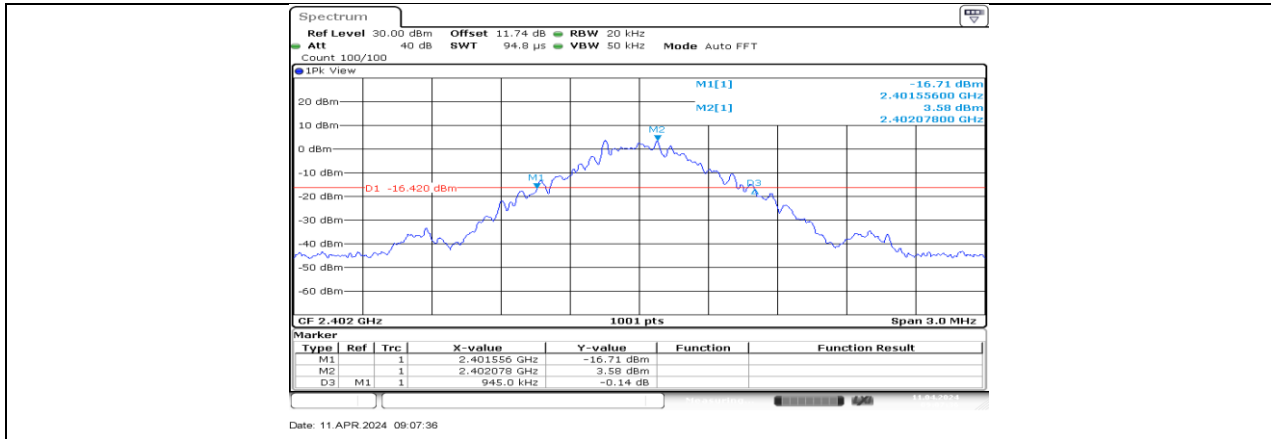
DH5_Ant3_2402
