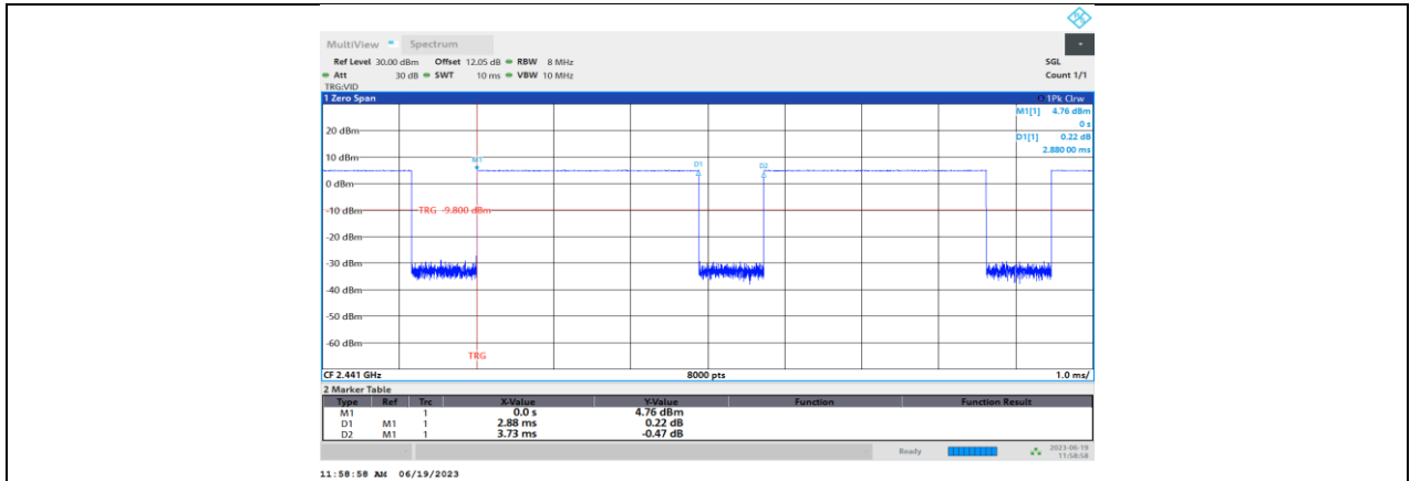
DH5_Ant1_2441
