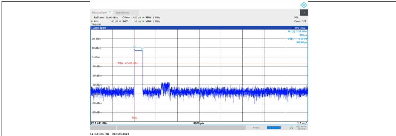
DH1_Ant1_Hop
