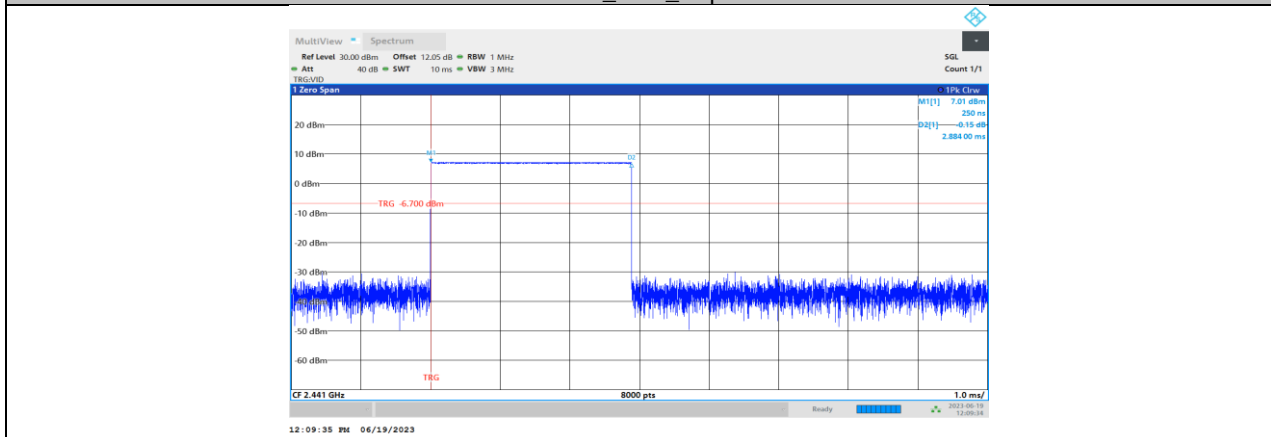
DH5_Ant1_Hop
