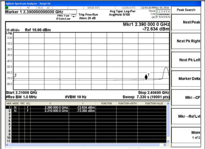
GFSK -Low channel(Average)
