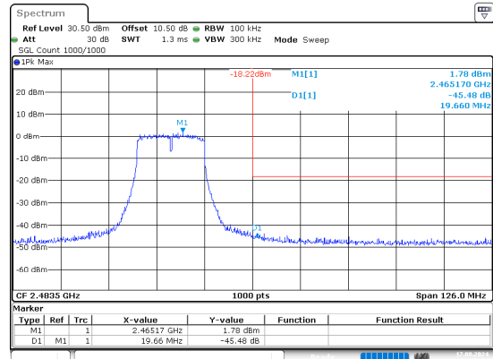
n20_2462MHz_Chain 1
