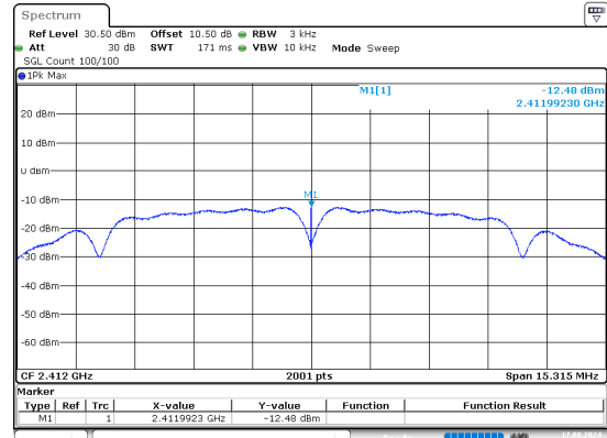
b_2412MHz_Chain 1
