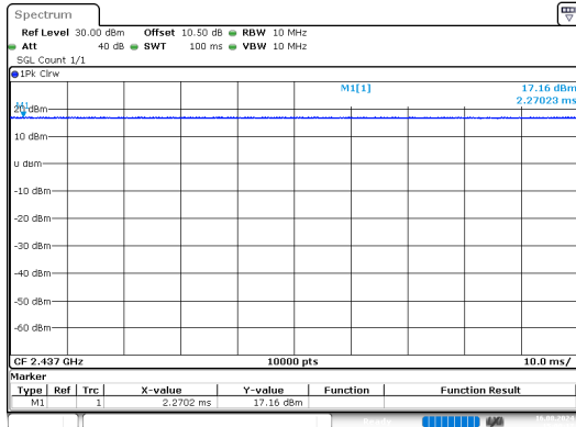
b_2437MHz
