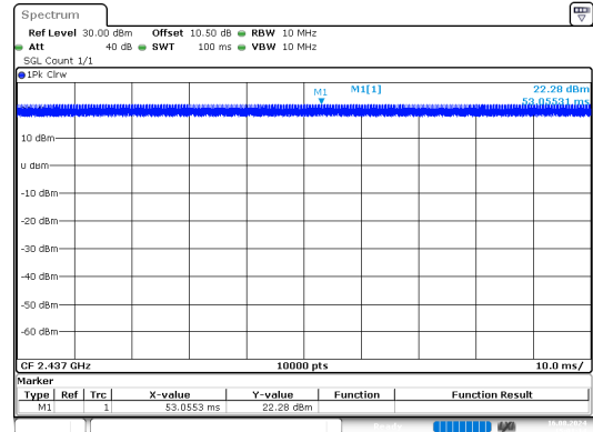
g_2437MHz
