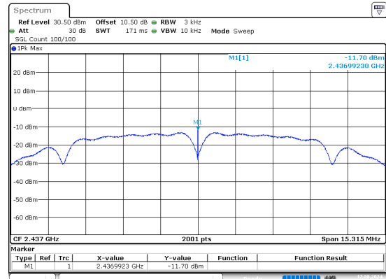
b_2437MHz_Chain 1
