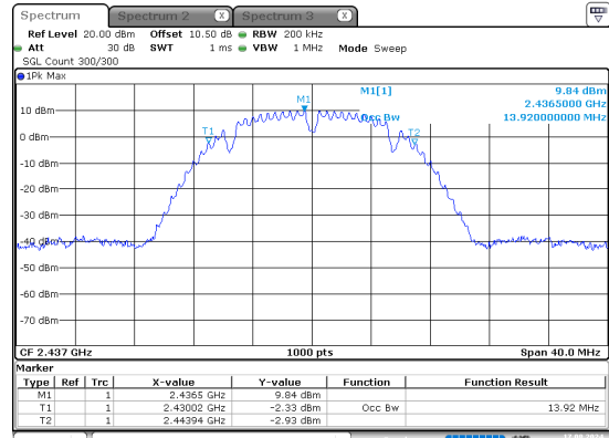
b_2437MHz
