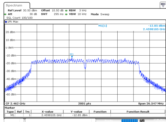
n20_2462MHz_Chain 1
