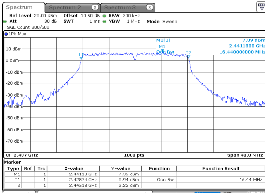
g_2437MHz
