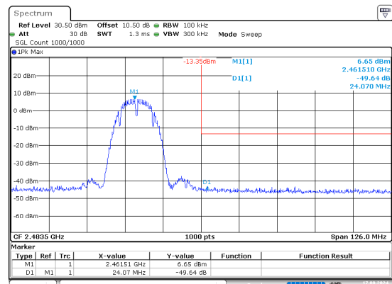
b_2462MHz_Chain 1
