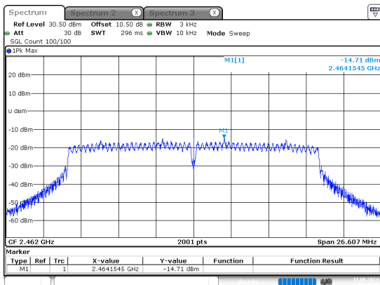
n20_2462MHz_Chain 0
