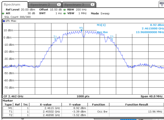
b_2462MHz
