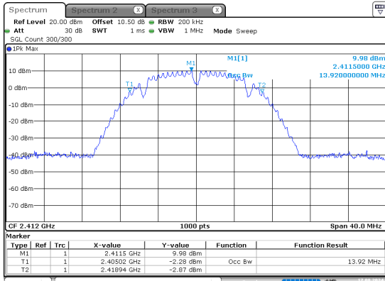
b_2412MHz
