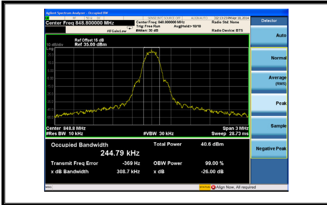
(Plot I1: GSM 850MHz Channel = 251)
