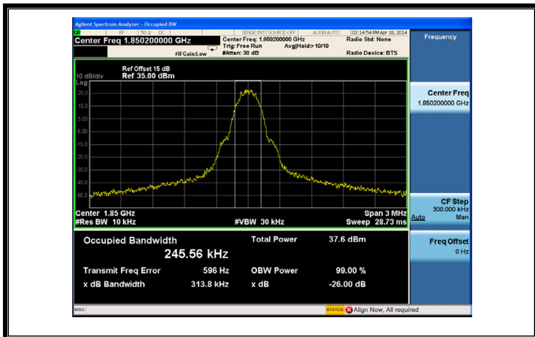
(Plot J1: GSM 1900MHz Channel = 512)
