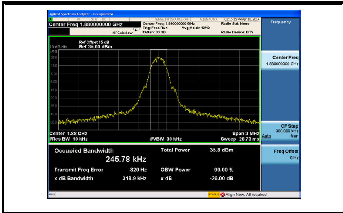
(Plot K1: GSM 1900MHz Channel = 661)
