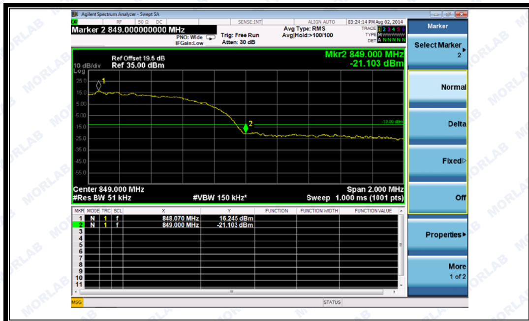
(Plot J: WCDMA 850 Channel = 4233)
