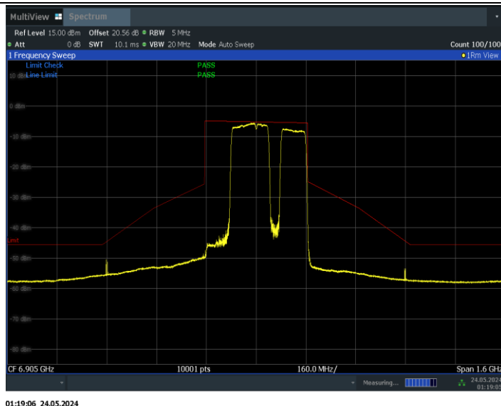
11BE320MIMO_Ant0_6905_2*996+484_Non-OFDMA_11
