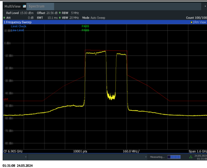
11BE320MIMO_Ant0_6905_3*996_Non-OFDMA_4
