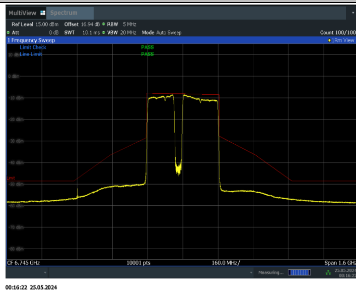
11BE320MIMO_Ant0_6745_3*996+484_Non-OFDMA_4
