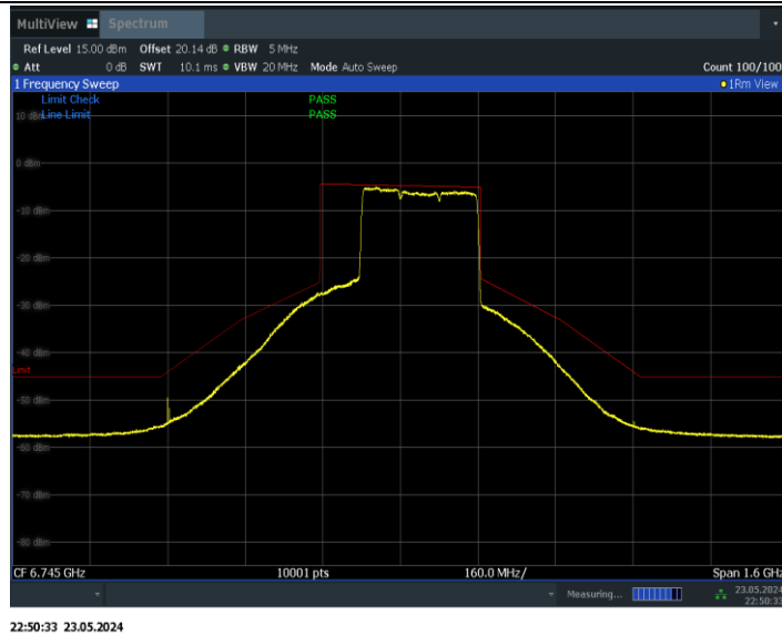
11BE320MIMO_Ant0_6745_3*996_Non-OFDMA_2
