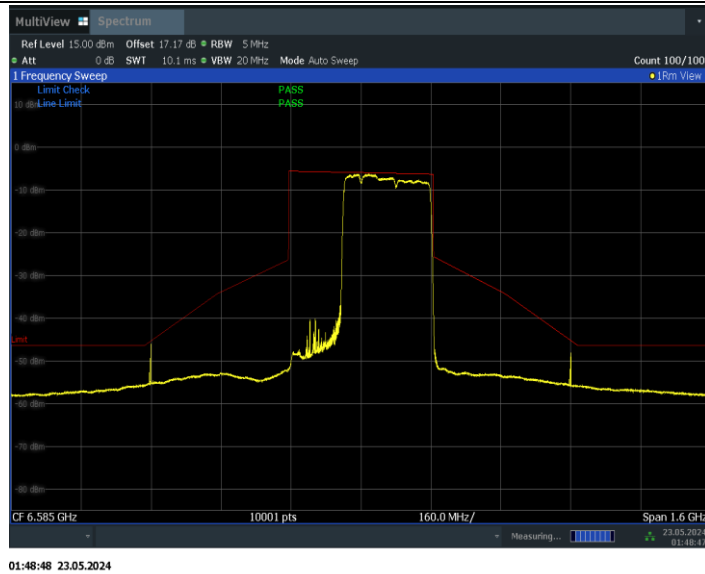
11BE320MIMO_Ant1_6585_2*996+484_Non-OFDMA_8
