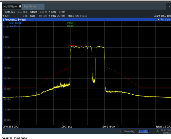
11BE320MIMO_Ant0_6585_3*996+484_Non-OFDMA_7
