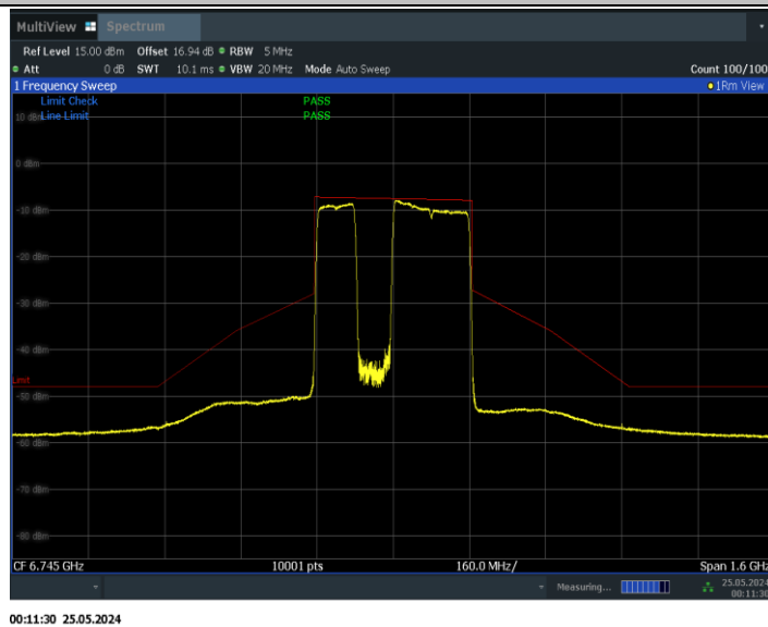
11BE320MIMO_Ant0_6745_3*996_Non-OFDMA_3
