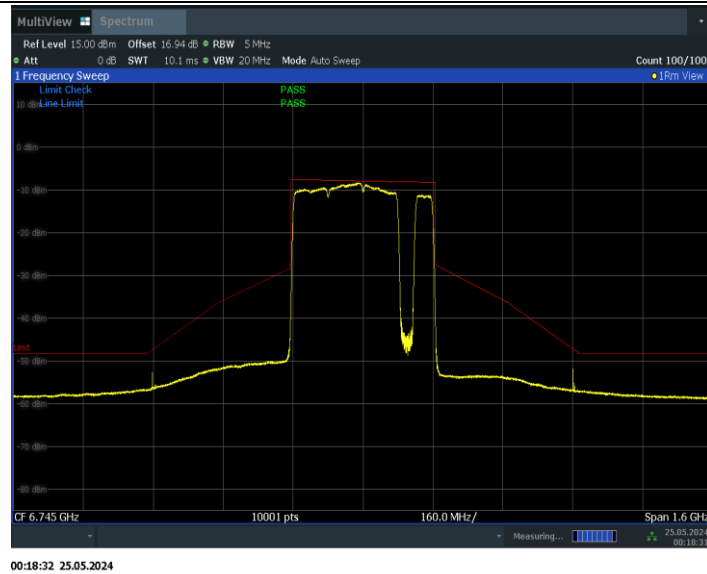
11BE320MIMO_Ant0_6745_3*996+484_Non-OFDMA_8
