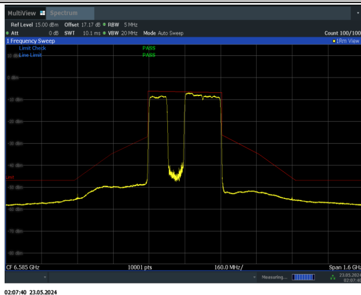
11BE320MIMO_Ant1_6585_3*996_Non-OFDMA_2
