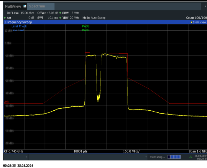
11BE320MIMO_Ant1_6745_3*996+484_Non-OFDMA_4
