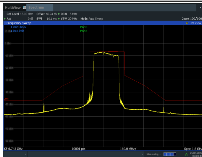
11BE320MIMO_Ant0_6745_2*996+484_Non-OFDMA_12
