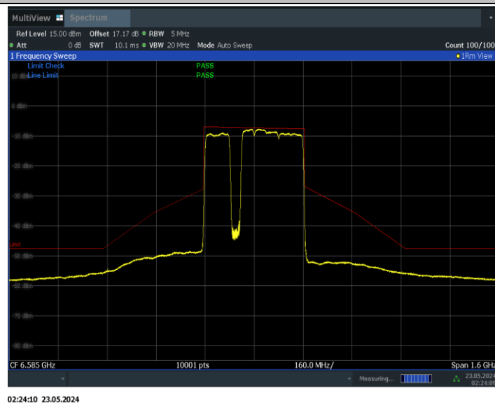
11BE320MIMO_Ant1_6585_3*996+484_Non-OFDMA_3
