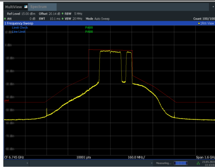
11BE320MIMO_Ant0_6745_2*996+484_Non-OFDMA_11
