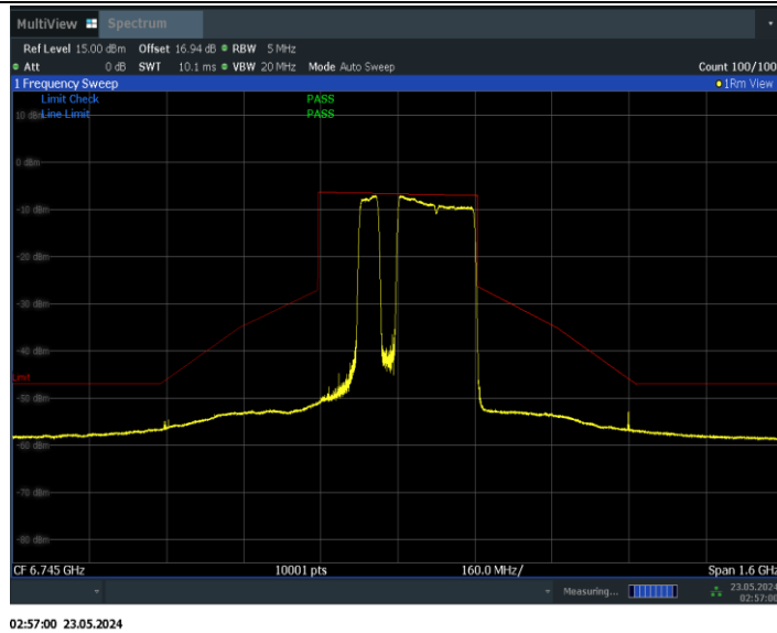
11BE320MIMO_Ant0_6745_2*996+484_Non-OFDMA_9
