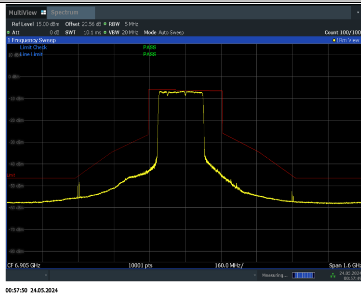
11BE320MIMO_Ant0_6905_2*996+484_Non-OFDMA_2
