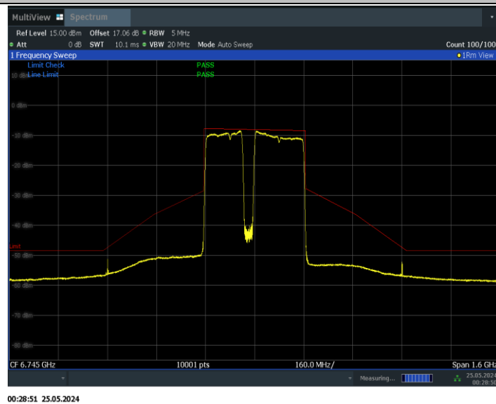
11BE320MIMO_Ant1_6745_3*996+484_Non-OFDMA_5
