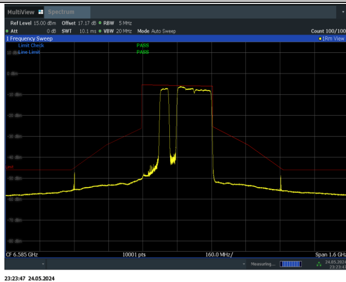
11BE320MIMO_Ant1_6585_2*996+484_Non-OFDMA_9
