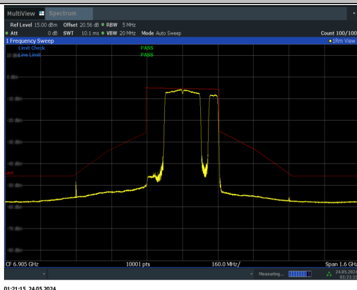
11BE320MIMO_Ant0_6905_2*996+484_Non-OFDMA_12
