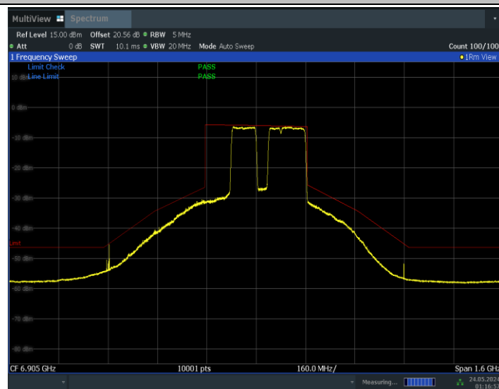
11BE320MIMO_Ant0_6905_2*996+484_Non-OFDMA_9
