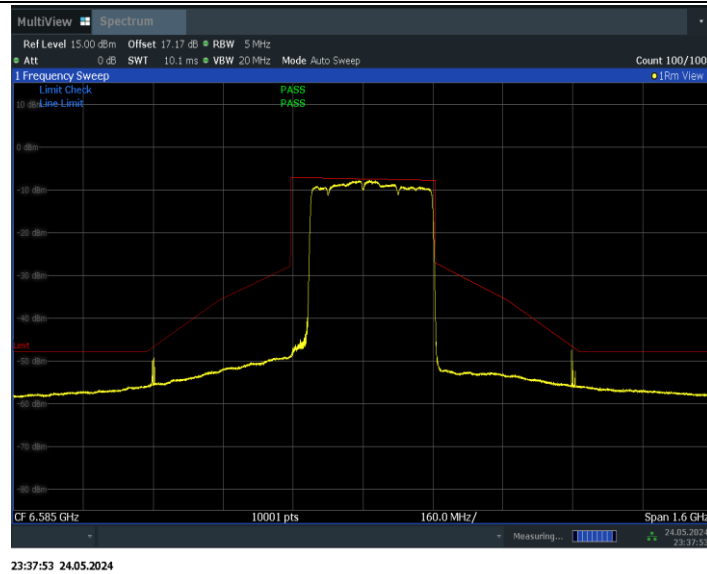
11BE320MIMO_Ant1_6585_3*996+484_Non-OFDMA_2
