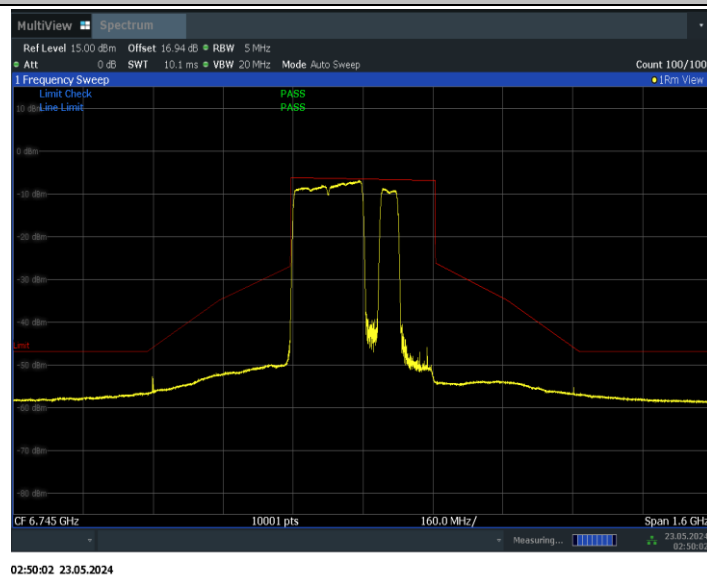
11BE320MIMO_Ant0_6745_2*996+484_Non-OFDMA_5
