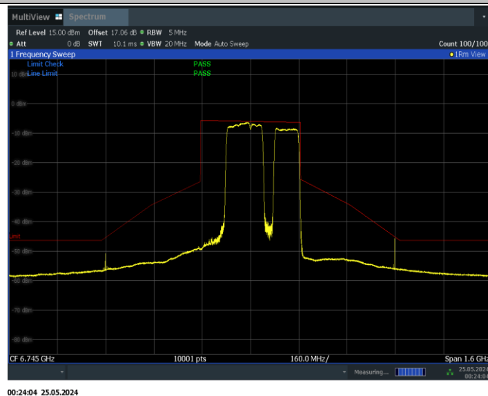
11BE320MIMO_Ant1_6745_2*996+484_Non-OFDMA_11
