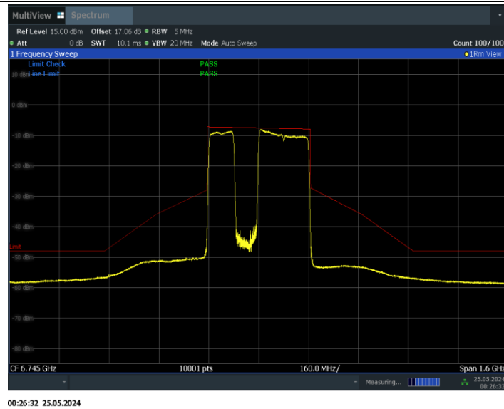
11BE320MIMO_Ant1_6745_3*996_Non-OFDMA_3
