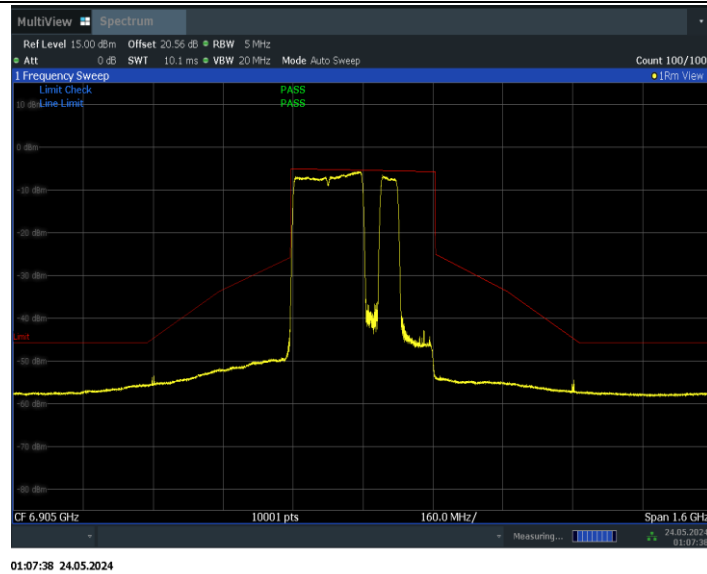
11BE320MIMO_Ant0_6905_2*996+484_Non-OFDMA_6
