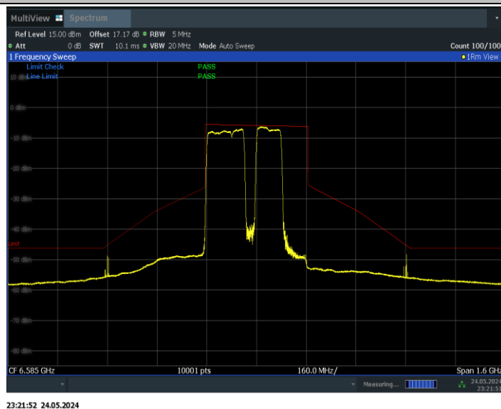
11BE320MIMO_Ant1_6585_2*996+484_Non-OFDMA_4
