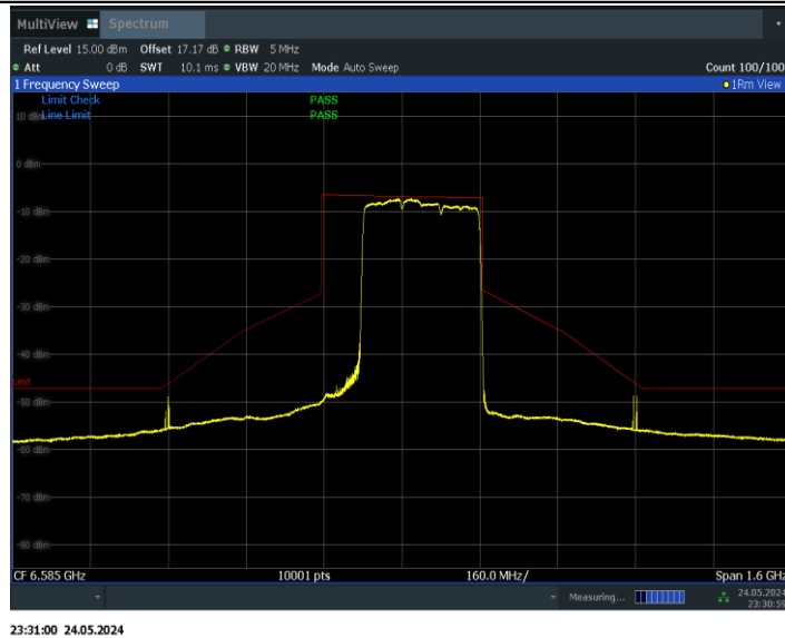
11BE320MIMO_Ant1_6585_3*996_Non-OFDMA_2
