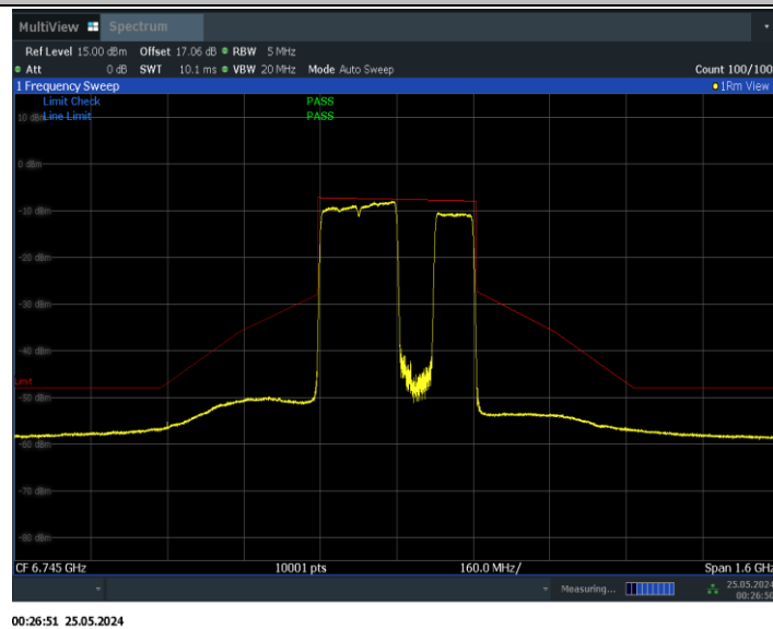
11BE320MIMO_Ant1_6745_3*996_Non-OFDMA_4
