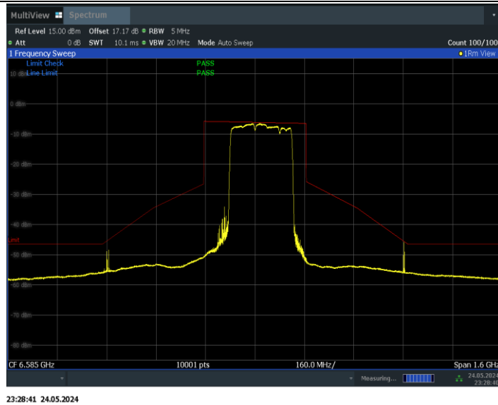
11BE320MIMO_Ant1_6585_3*996_Non-OFDMA_1
