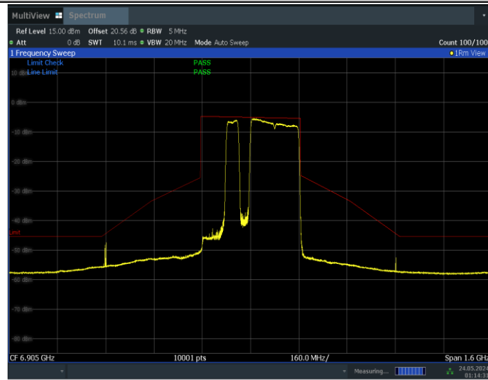
11BE320MIMO_Ant0_6905_2*996+484_Non-OFDMA_8
