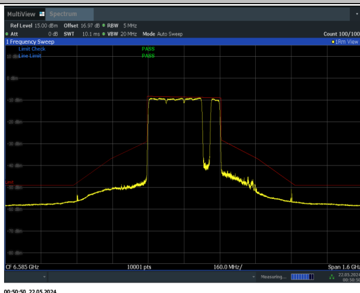
11BE320MIMO_Ant0_6585_3*996+484_Non-OFDMA_7
