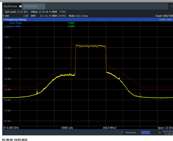
11BE320MIMO_Ant0_6905_3*996+484_Non-OFDMA_1
