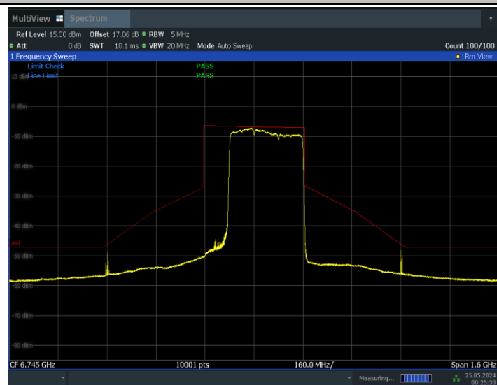
11BE320MIMO_Ant1_6745_3*996_Non-OFDMA_1
