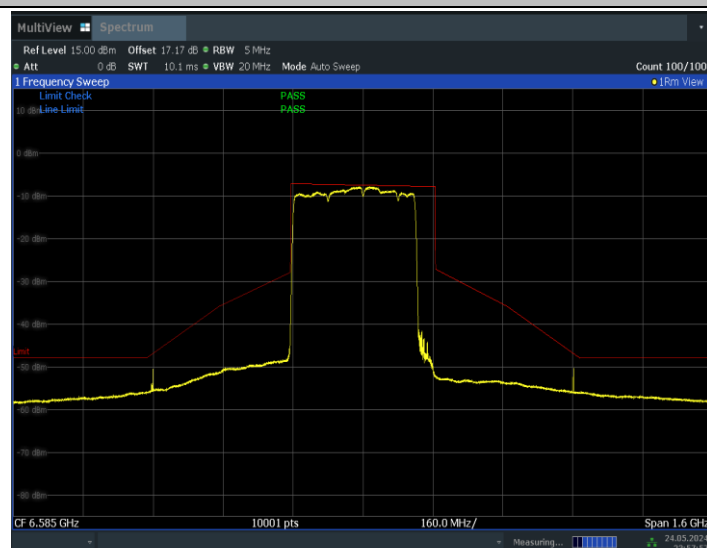
11BE320MIMO_Ant1_6585_3*996+484_Non-OFDMA_8
