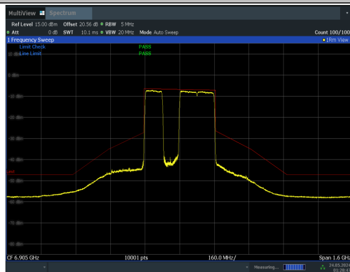
11BE320MIMO_Ant0_6905_3*996_Non-OFDMA_2
