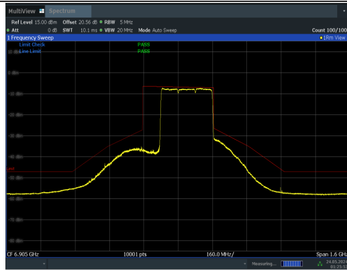
11BE320MIMO_Ant0_6905_3*996_Non-OFDMA_1
