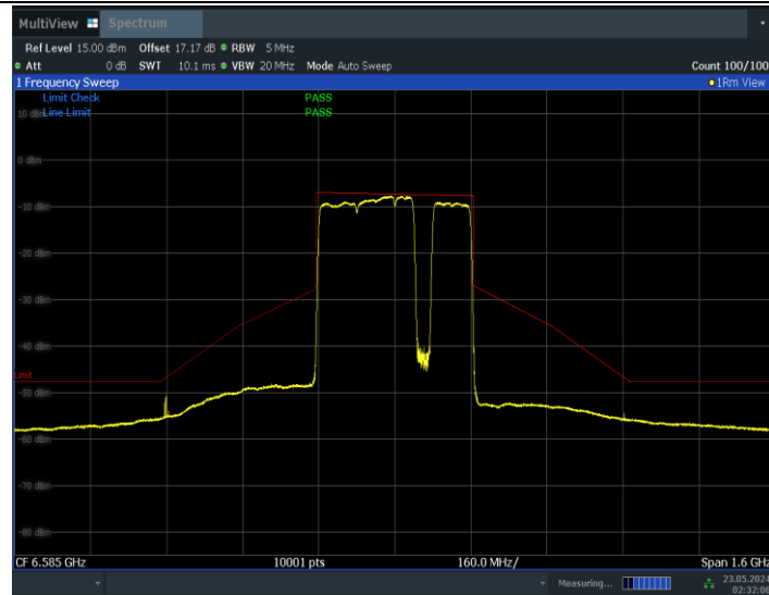
11BE320MIMO_Ant1_6585_3*996+484_Non-OFDMA_7
