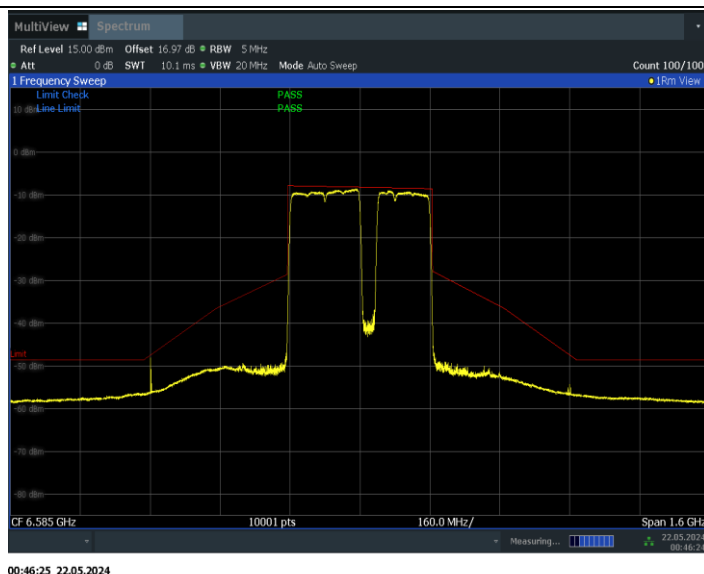
11BE320MIMO_Ant0_6585_3*996+484_Non-OFDMA_6
