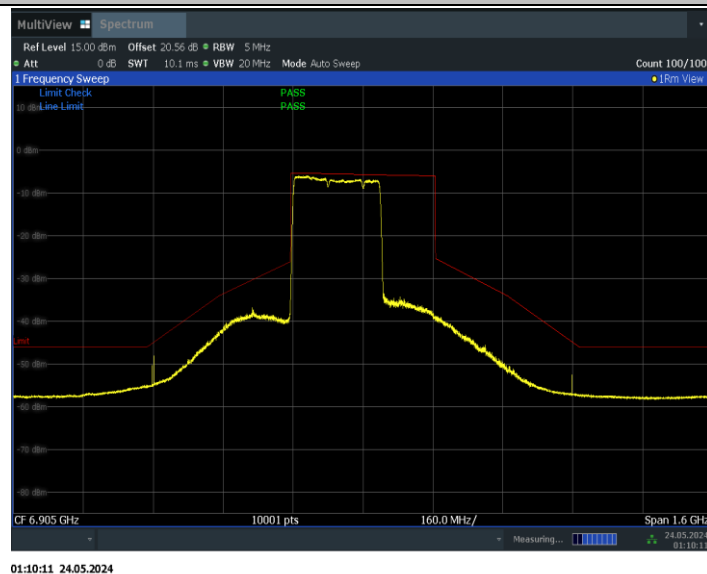
11BE320MIMO_Ant0_6905_2*996+484_Non-OFDMA_7
