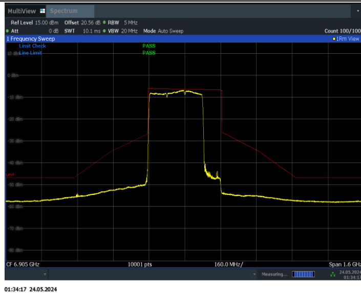
11BE320MIMO_Ant0_6905_3*996+484_Non-OFDMA_1
