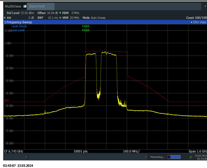
11BE320MIMO_Ant0_6745_2*996+484_Non-OFDMA_4
