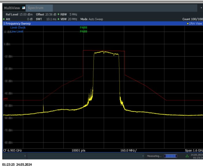
11BE320MIMO_Ant0_6905_2*996+484_Non-OFDMA_12
