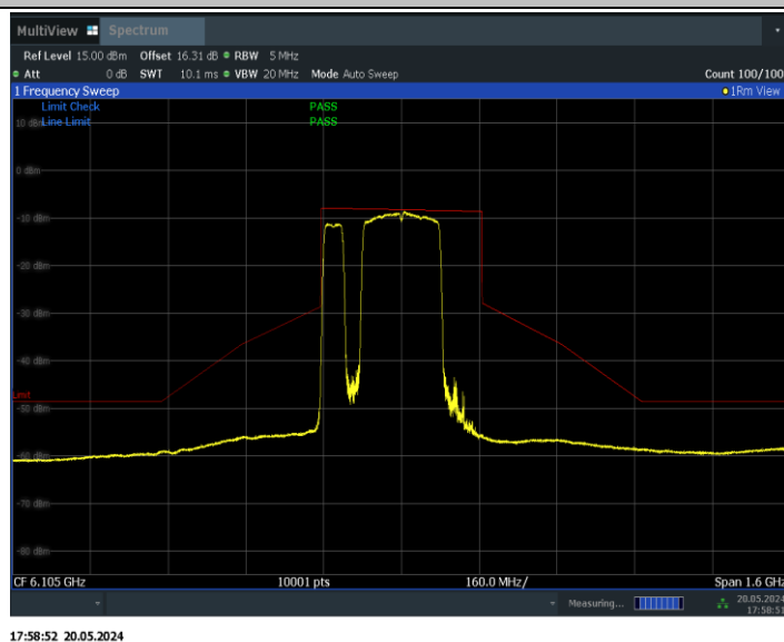
11BE320MIMO_Ant0_6105_2*996+484_Non-OFDMA_2
