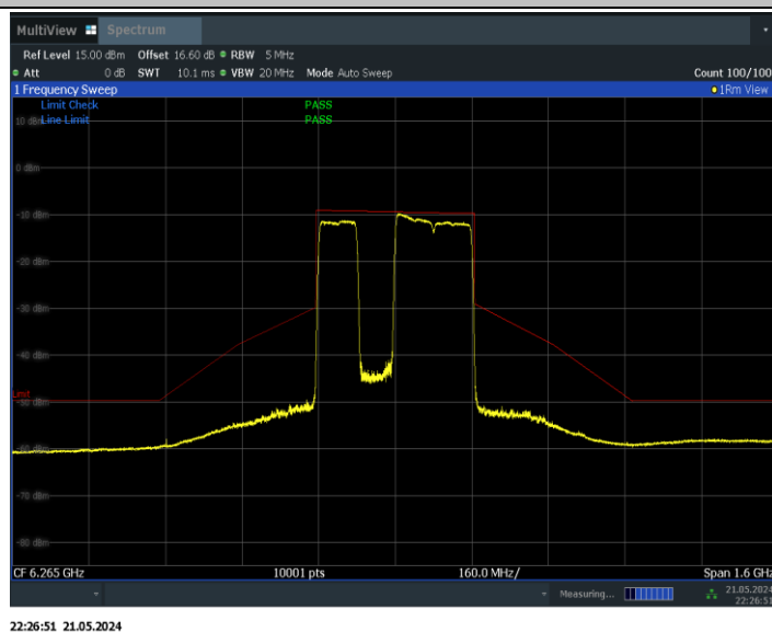
11BE320MIMO_Ant0_6265_3*996_Non-OFDMA_2
