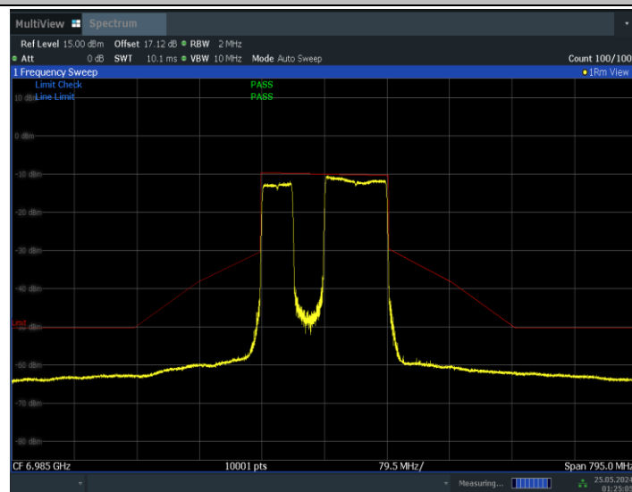
11BE160MIMO_Ant0_6985_996+484_Non-OFDMA_3
