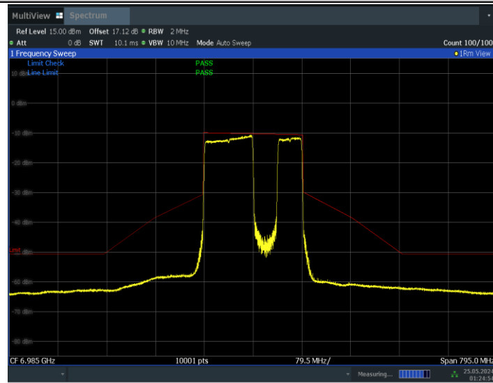
11BE160MIMO_Ant0_6985_996+484_Non-OFDMA_2
