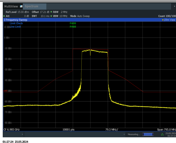
11BE160MIMO_Ant1_6985_996+484_Non-OFDMA_4
