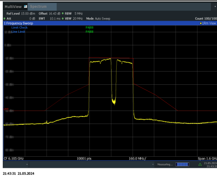
11BE320MIMO_Ant1_6105_3*996+484_Non-OFDMA_6
