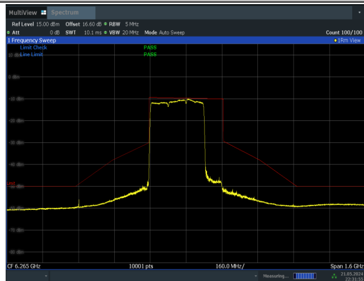
11BE320MIMO_Ant0_6265_3*996_Non-OFDMA_4
