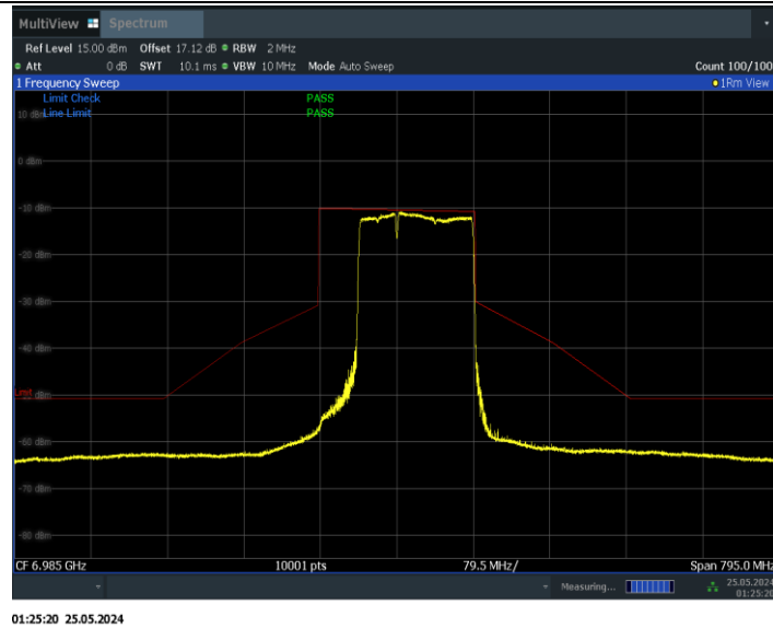
11BE160MIMO_Ant0_6985_996+484+242_Non-OFDMA_1
