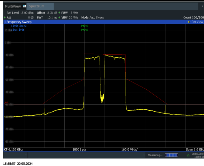
11BE320MIMO_Ant0_6105_3*996+484_Non-OFDMA_5
