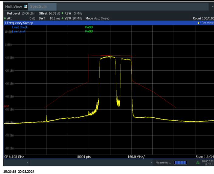
11BE320MIMO_Ant0_6105_2*996+484_Non-OFDMA_11
