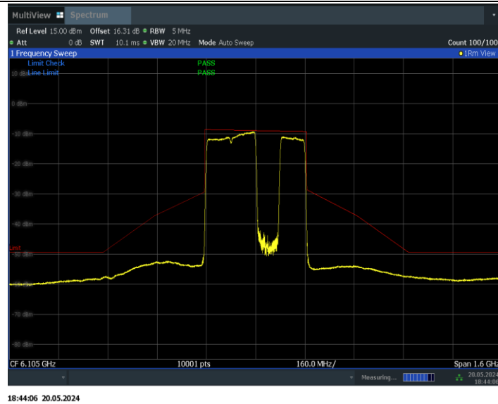
11BE320MIMO_Ant0_6105_3*996_Non-OFDMA_4
