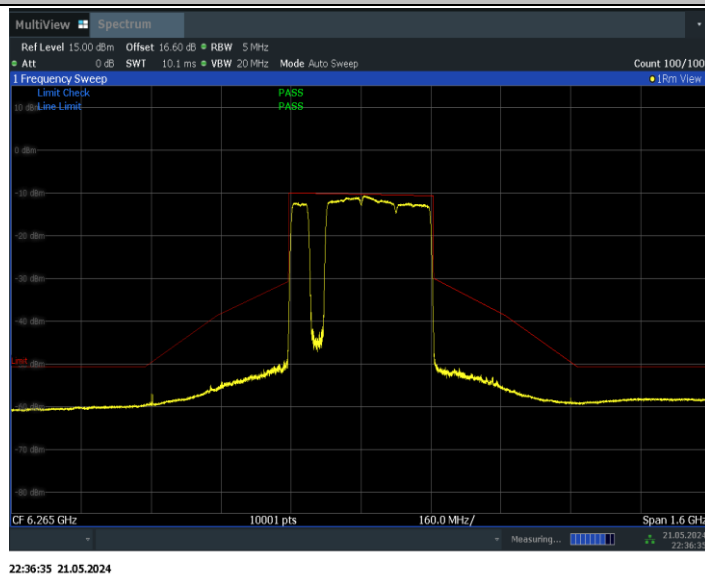
11BE320MIMO_Ant0_6265_3*996+484_Non-OFDMA_3
