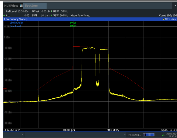
11BE320MIMO_Ant0_6265_2*996+484_Non-OFDMA_10
