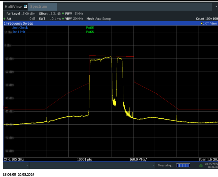
11BE320MIMO_Ant0_6105_2*996+484_Non-OFDMA_6
