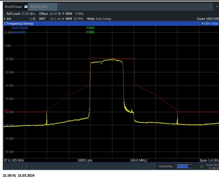
11BE320MIMO_Ant1_6105_3*996+484_Non-OFDMA_1
