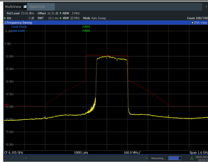
11BE320MIMO_Ant0_6105_3*996_Non-OFDMA_1
