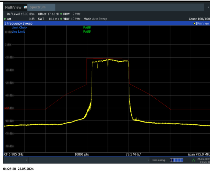
11BE160MIMO_Ant0_6985_996+484+242_Non-OFDMA_2
