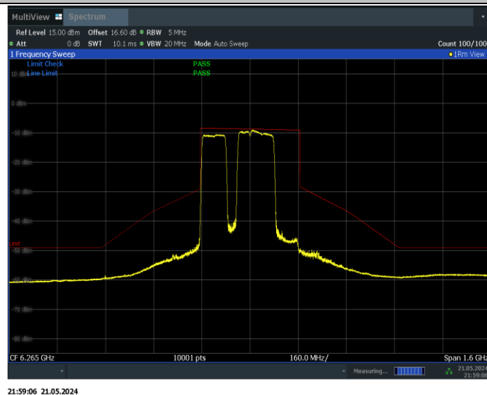
11BE320MIMO_Ant0_6265_2*996+484_Non-OFDMA_4
