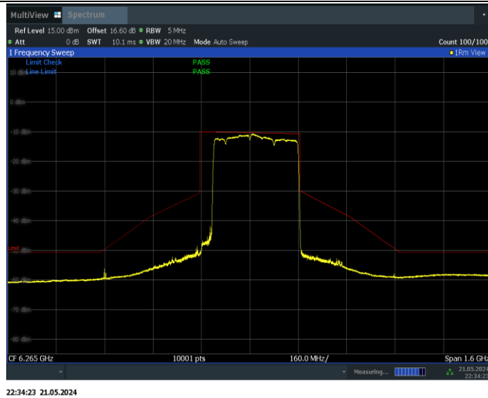
11BE320MIMO_Ant0_6265_3*996+484_Non-OFDMA_2
