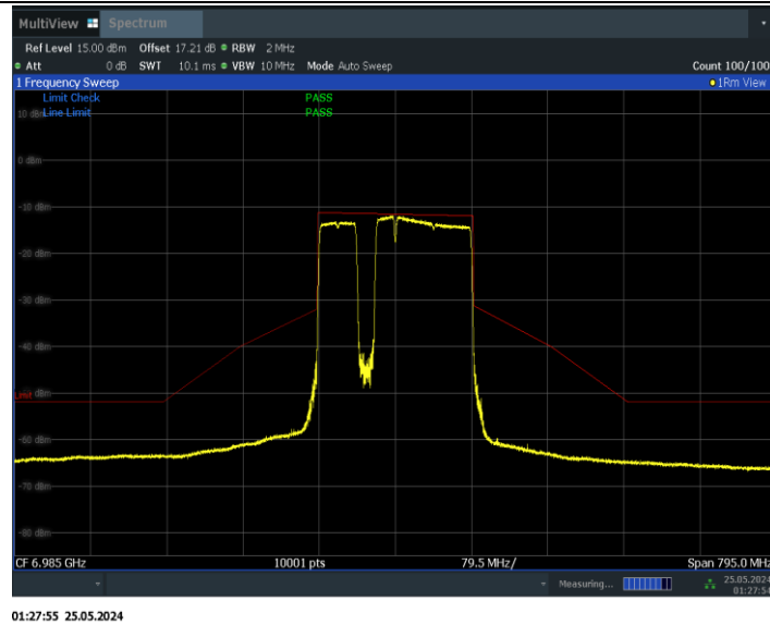
11BE160MIMO_Ant1_6985_996+484+242_Non-OFDMA_4
