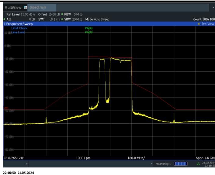
11BE320MIMO_Ant0_6265_2*996+484_Non-OFDMA_9
