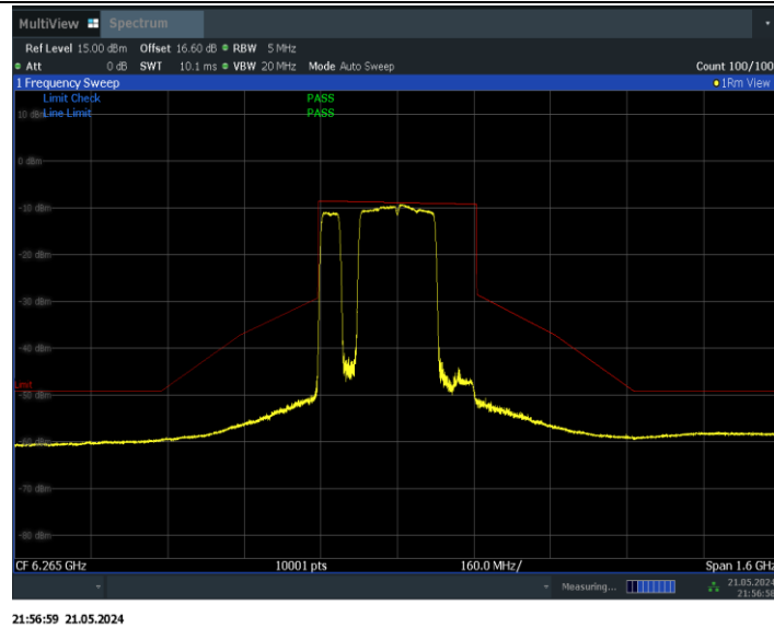
11BE320MIMO_Ant0_6265_2*996+484_Non-OFDMA_3
