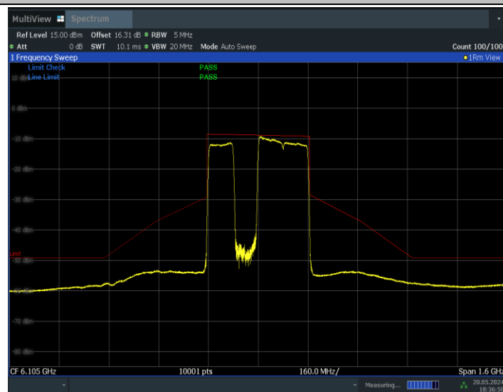
11BE320MIMO_Ant0_6105_3*996_Non-OFDMA_2
