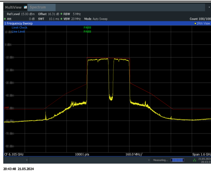
11BE320MIMO_Ant0_6105_3*996+484_Non-OFDMA_6
