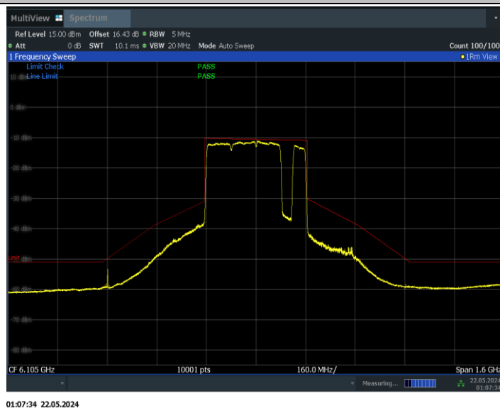
11BE320MIMO_Ant1_6105_3*996+484_Non-OFDMA_7
