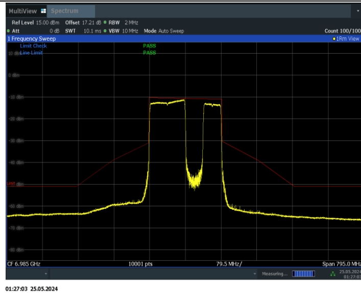
11BE160MIMO_Ant1_6985_996+484_Non-OFDMA_3
