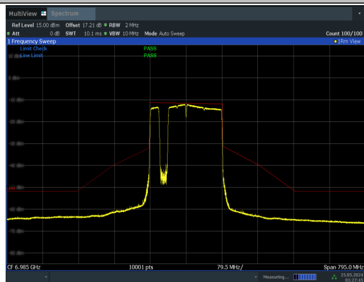
11BE160MIMO_Ant1_6985_996+484+242_Non-OFDMA_2
