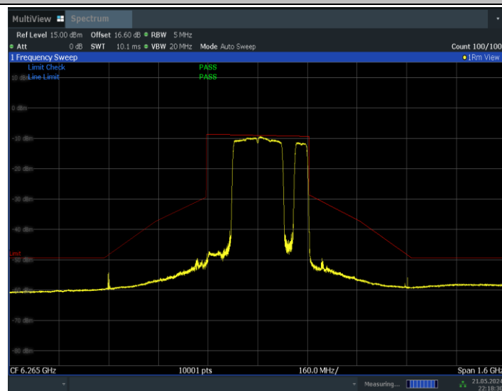
11BE320MIMO_Ant0_6265_2*996+484_Non-OFDMA_11
