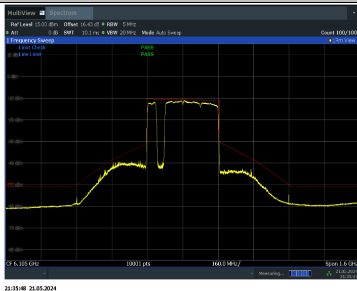
11BE320MIMO_Ant1_6105_3*996+484_Non-OFDMA_2
