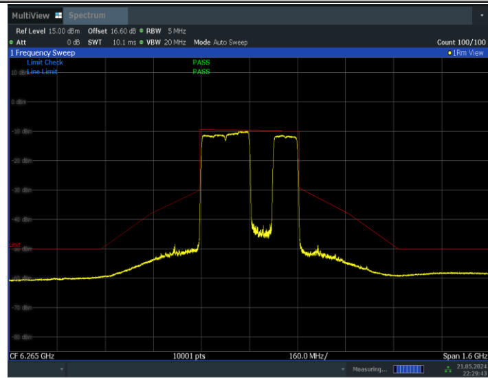
11BE320MIMO_Ant0_6265_3*996_Non-OFDMA_3
