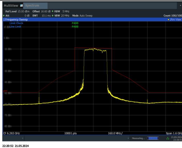
11BE320MIMO_Ant0_6265_3*996_Non-OFDMA_1
