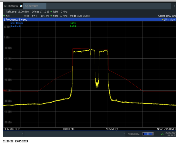
11BE160MIMO_Ant0_6985_996+484+242_Non-OFDMA_7
