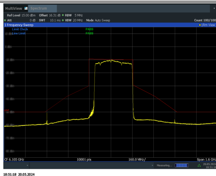
11BE320MIMO_Ant0_6105_3*996+484_Non-OFDMA_1
