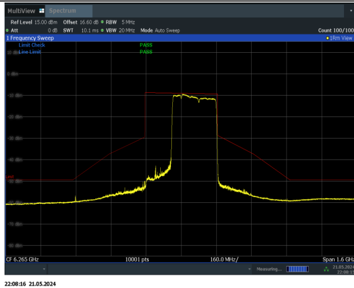
11BE320MIMO_Ant0_6265_2*996+484_Non-OFDMA_8
