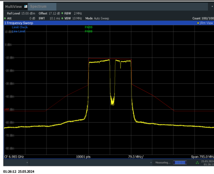
11BE160MIMO_Ant0_6985_996+484+242_Non-OFDMA_6
