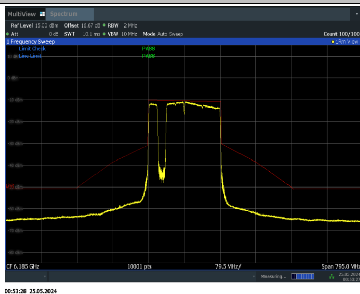
11BE160MIMO_Ant0_6185_996+484+242_Non-OFDMA_2
