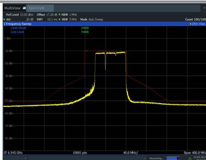
11BE80MIMO_Ant0_6945_484+242_Non-OFDMA_1
