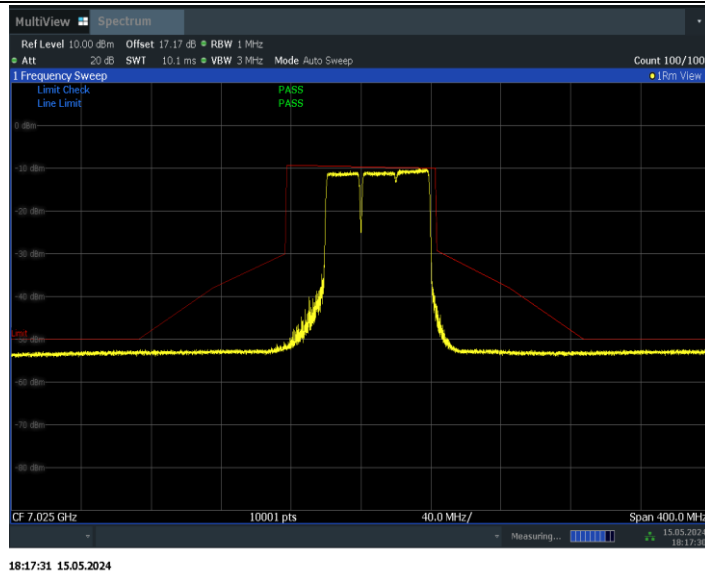
11BE80MIMO_Ant0_7025_484+242_Non-OFDMA_2
