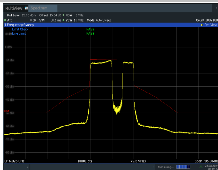
11BE160MIMO_Ant0_6025_996+484_Non-OFDMA_2
