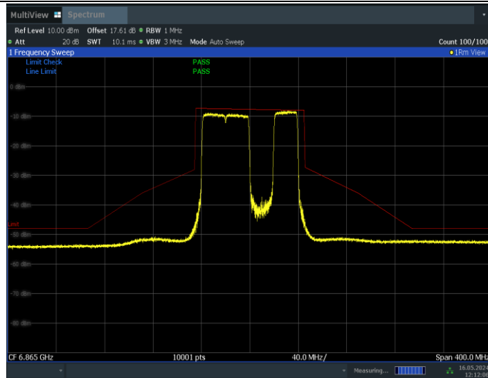
11BE80MIMO_Ant1_6865_484+242_Non-OFDMA_4
