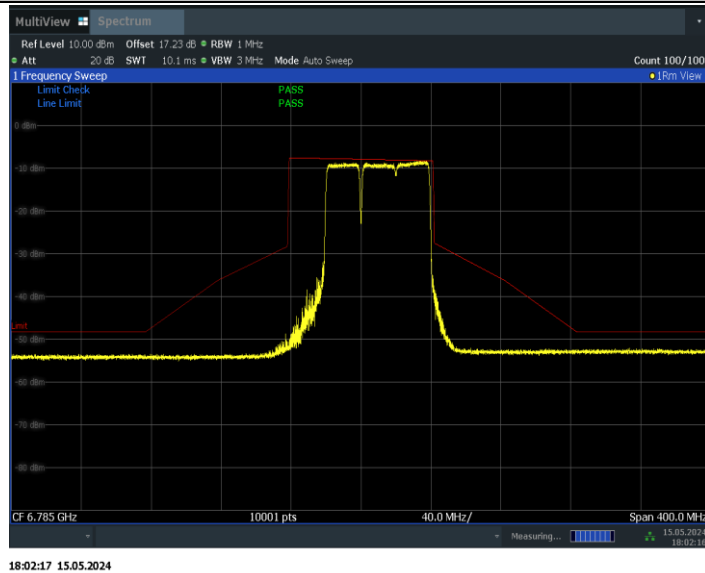
11BE80MIMO_Ant0_6785_484+242_Non-OFDMA_2
