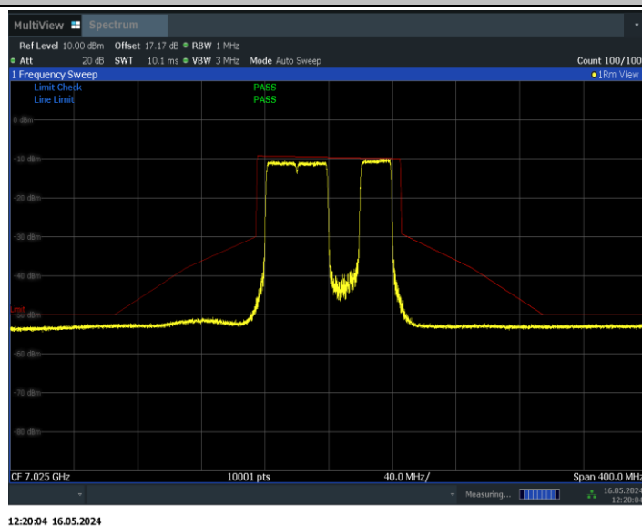
11BE80MIMO_Ant0_7025_484+242_Non-OFDMA_3
