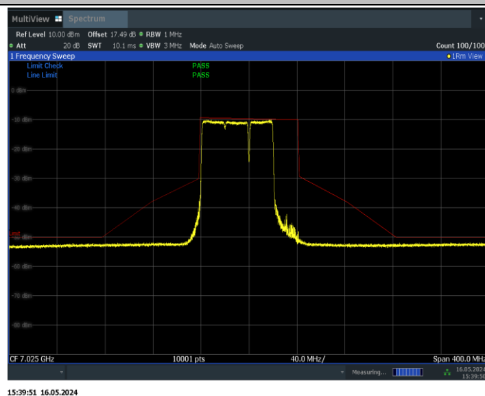
11BE80MIMO_Ant1_7025_484+242_Non-OFDMA_4
