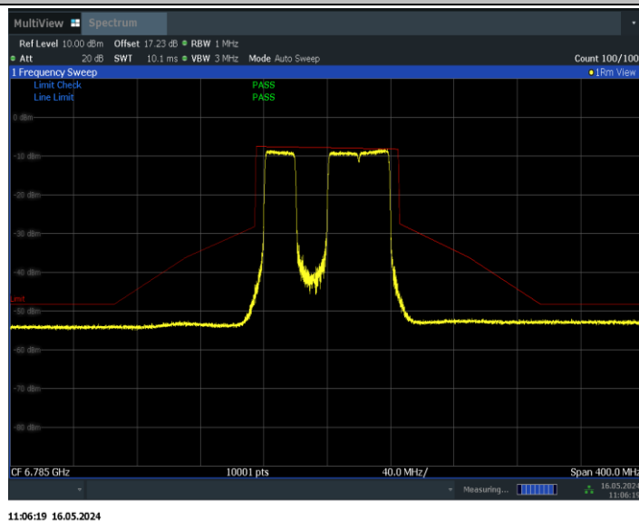
11BE80MIMO_Ant0_6785_484+242_Non-OFDMA_2
