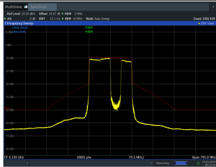
11BE160MIMO_Ant0_6185_996+484_Non-OFDMA_2
