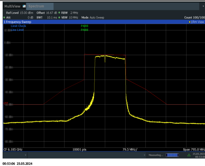
11BE160MIMO_Ant0_6185_996+484+242_Non-OFDMA_1
