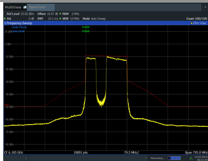
11BE160MIMO_Ant0_6185_996+484_Non-OFDMA_3
