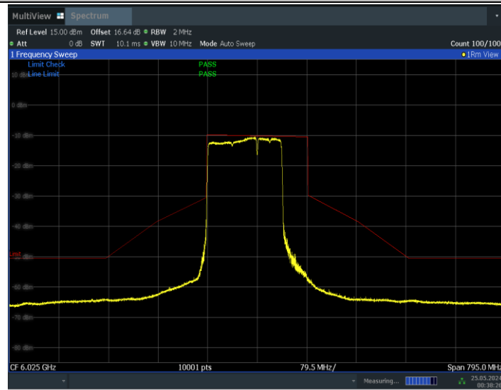
11BE160MIMO_Ant0_6025_996+484_Non-OFDMA_1
