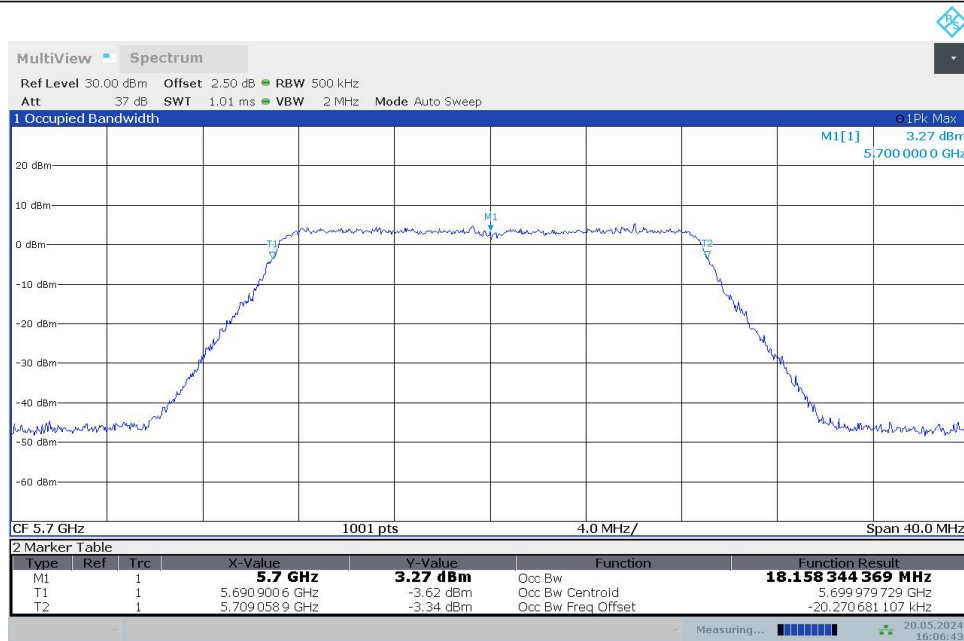
11AC20MIMO_Ant1_5700
