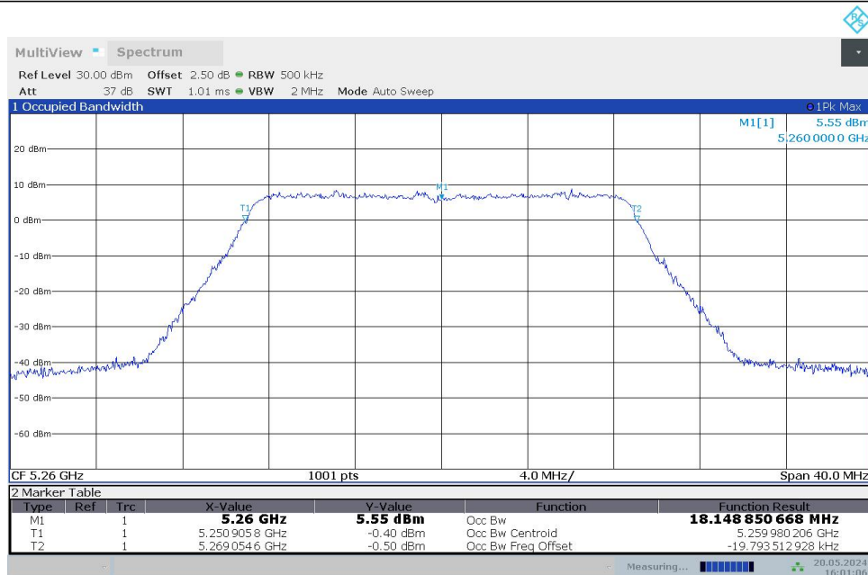
11AC20MIMO_Ant0_5260
