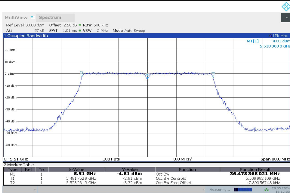
11N40MIMO_Ant1_5510
