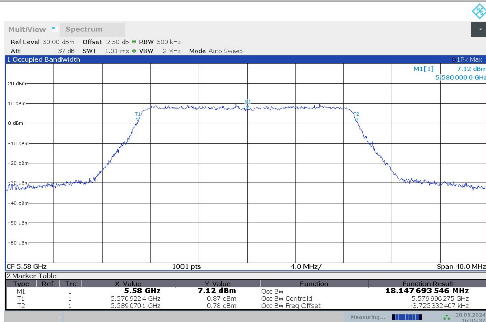
11AC20MIMO_Ant0_5580
