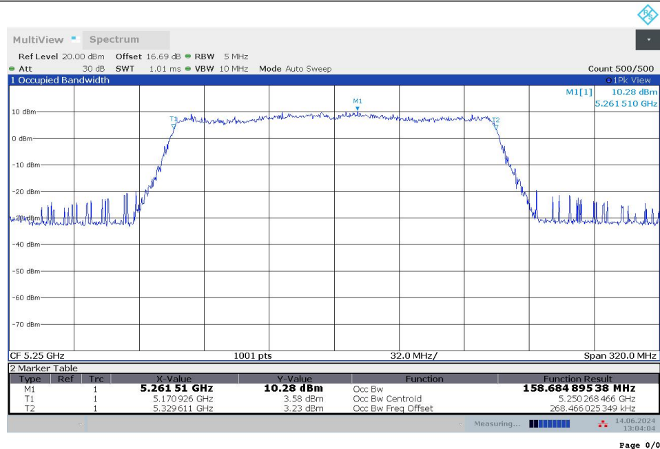
11AX160MIMO_Ant1_5250
