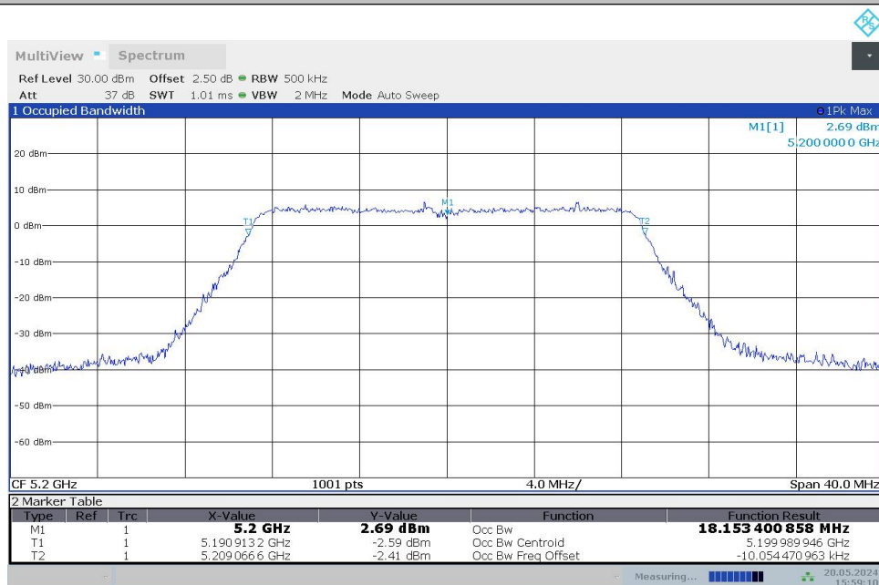
11AC20MIMO_Ant0_5200
