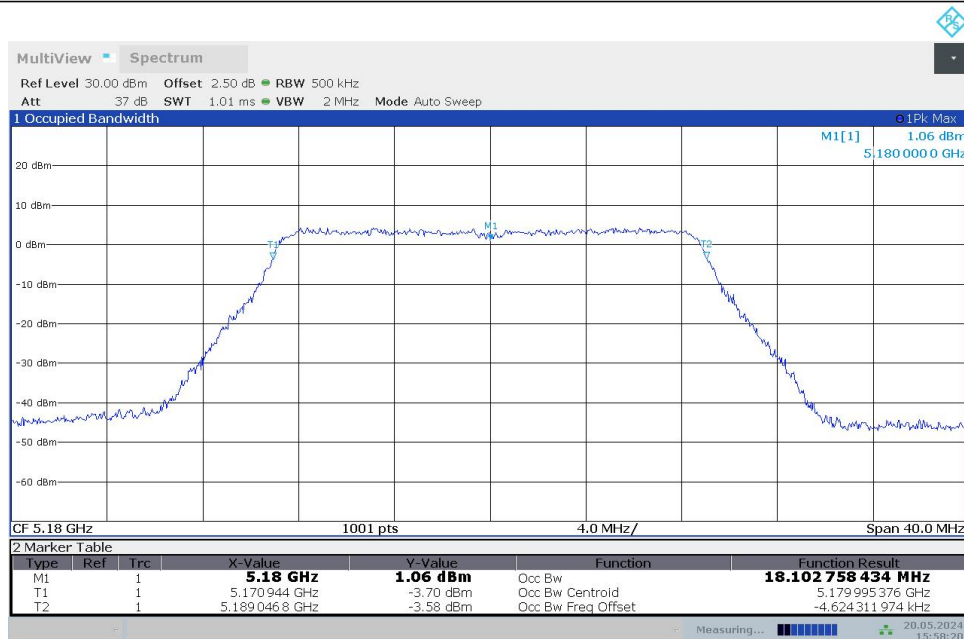
11AC20MIMO_Ant0_5180
