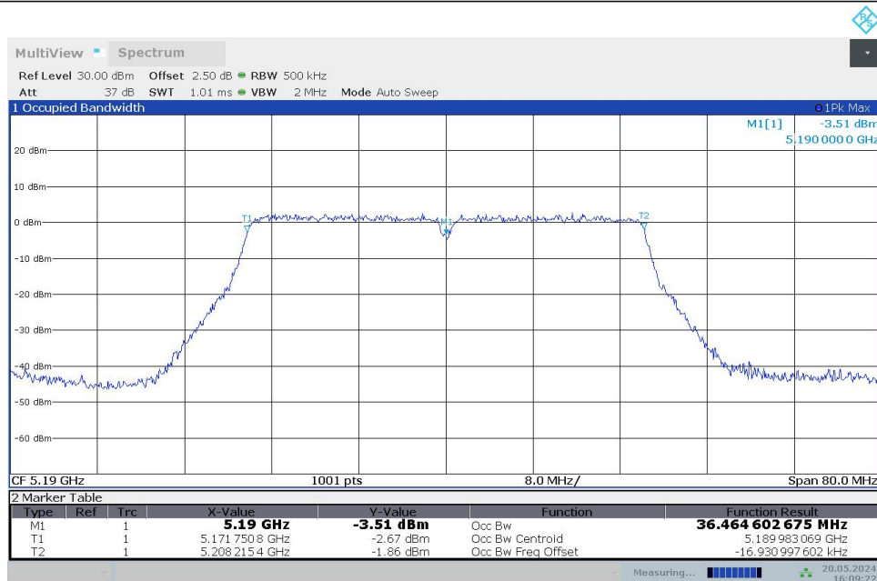
11N40MIMO_Ant0_5190
