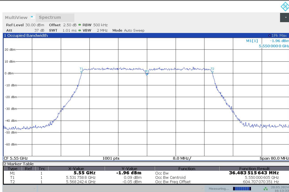
11N40MIMO_Ant1_5550
