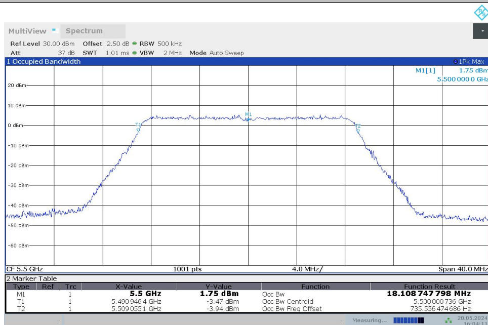
11AC20MIMO_Ant0_5500
