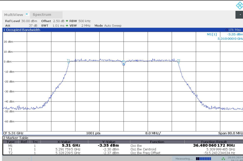
11N40MIMO_Ant0_5310
