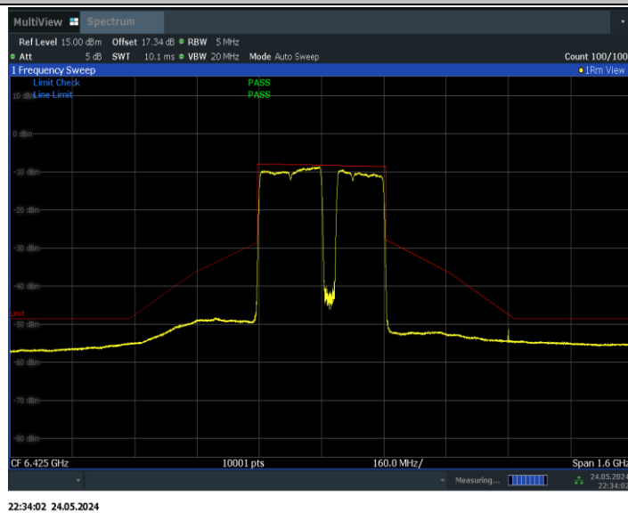
11BE320MIMO_Ant1_6425_3*996+484_Non-OFDMA_6
