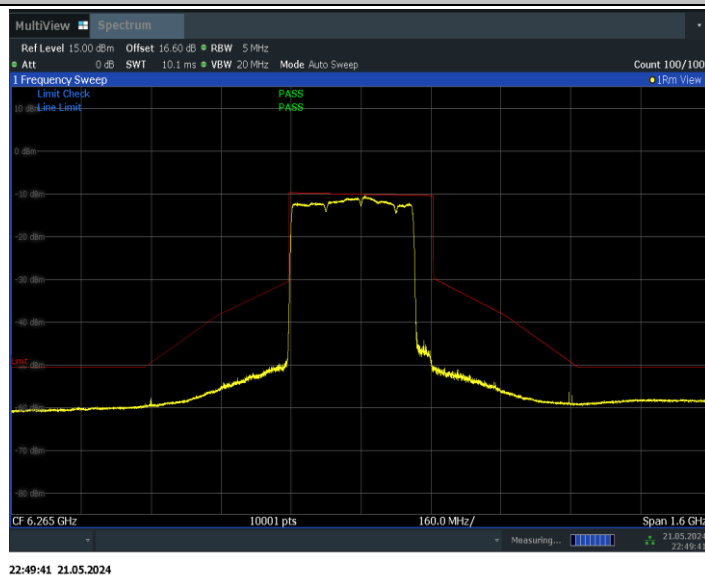
11BE320MIMO_Ant0_6265_3*996+484_Non-OFDMA_8
