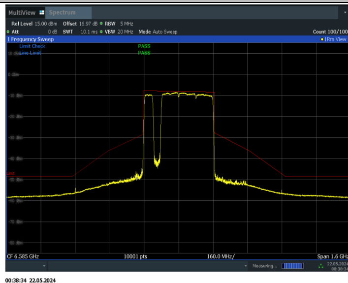
11BE320MIMO_Ant0_6585_3*996+484_Non-OFDMA_2
