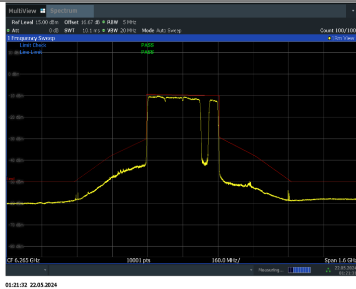
11BE320MIMO_Ant1_6265_3*996+484_Non-OFDMA_8
