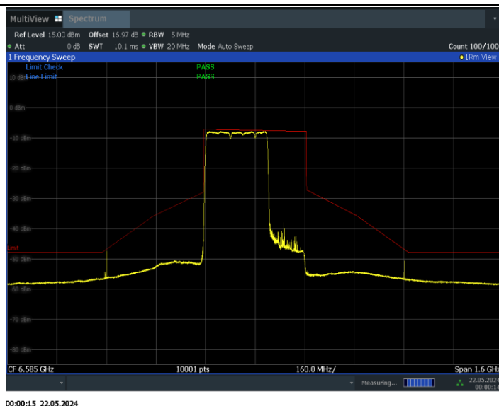
11BE320MIMO_Ant0_6585_2*996+484_Non-OFDMA_7
