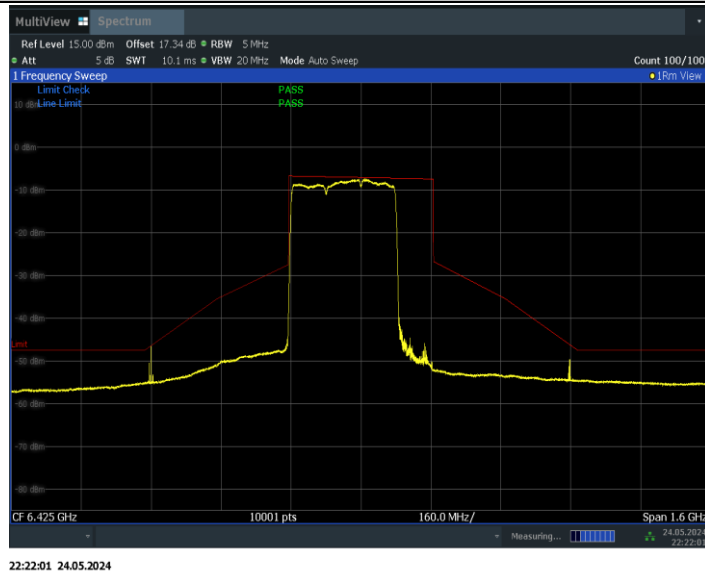
11BE320MIMO_Ant1_6425_3*996+484_Non-OFDMA_1
