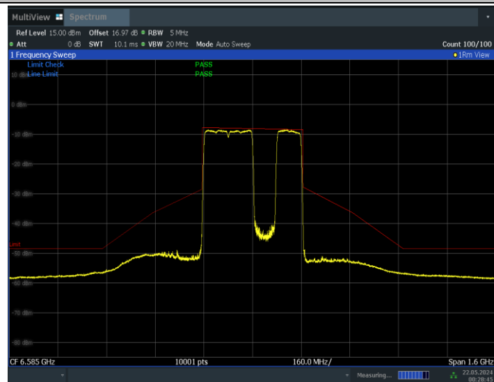
11BE320MIMO_Ant0_6585_3*996_Non-OFDMA_3
