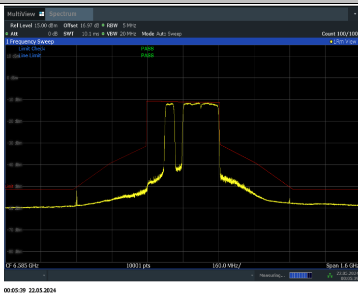
11BE320MIMO_Ant0_6585_2*996+484_Non-OFDMA_8
