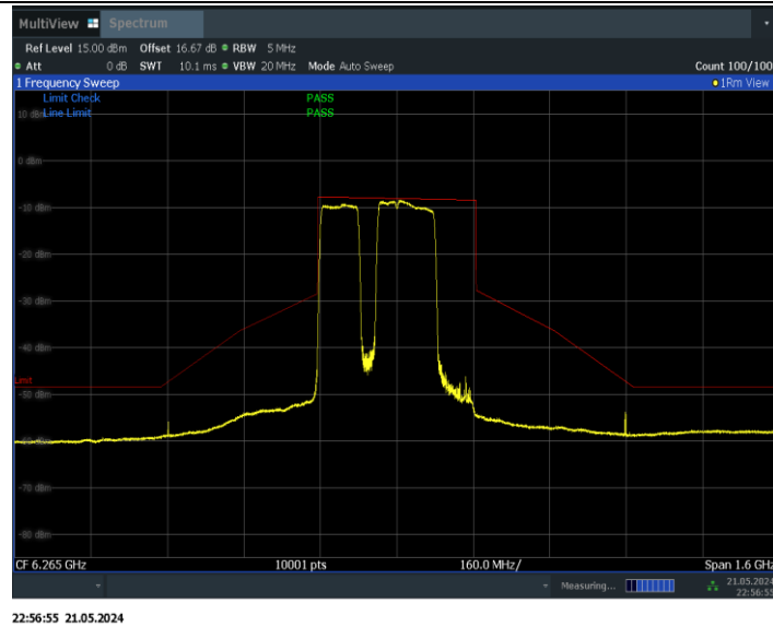
11BE320MIMO_Ant1_6265_2*996+484_Non-OFDMA_4
