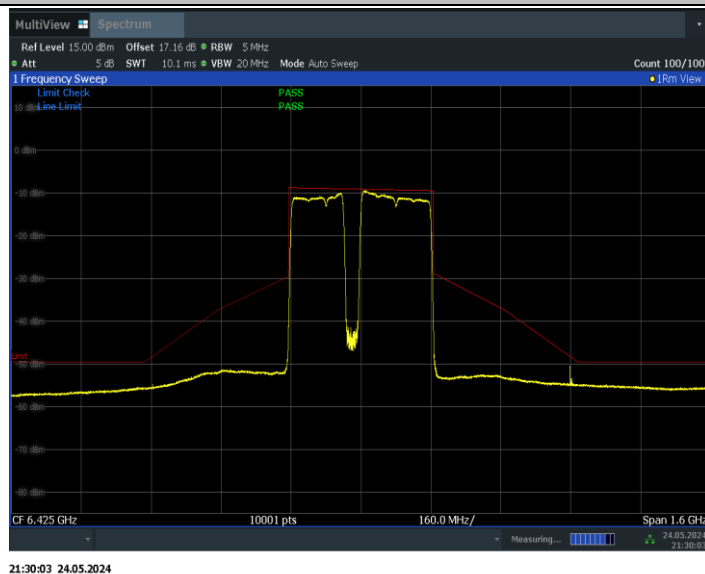
11BE320MIMO_Ant0_6425_3*996+484_Non-OFDMA_5
