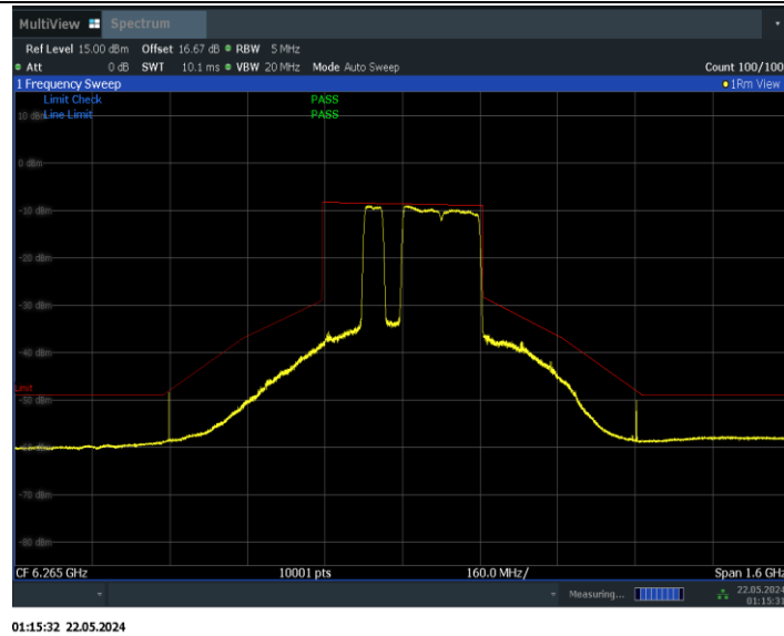
11BE320MIMO_Ant1_6265_2*996+484_Non-OFDMA_9
