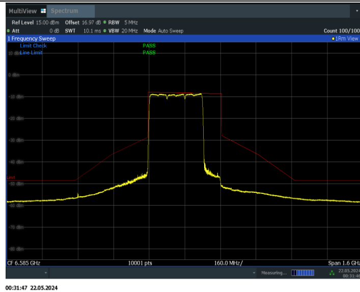
11BE320MIMO_Ant0_6585_3*996+484_Non-OFDMA_1
