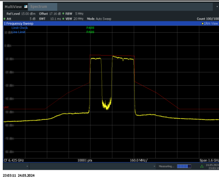
11BE320MIMO_Ant0_6425_3*996_Non-OFDMA_3
