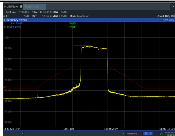
11BE320MIMO_Ant0_6425_3*996_Non-OFDMA_1
