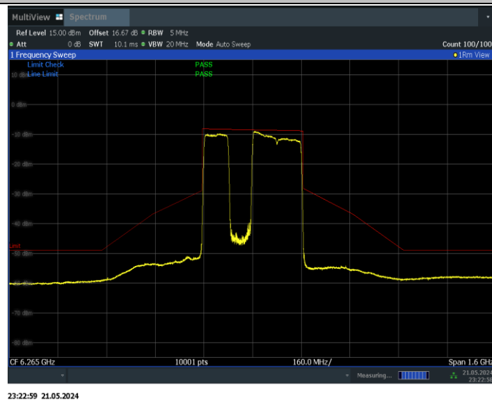
11BE320MIMO_Ant1_6265_3*996_Non-OFDMA_3
