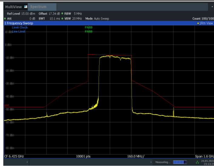
11BE320MIMO_Ant1_6425_3*996_Non-OFDMA_1
