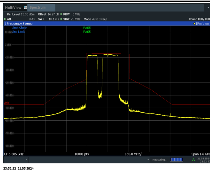
11BE320MIMO_Ant0_6585_2*996+484_Non-OFDMA_3
