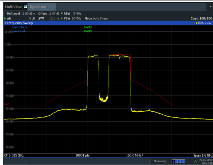
11BE320MIMO_Ant0_6585_3*996_Non-OFDMA_2
