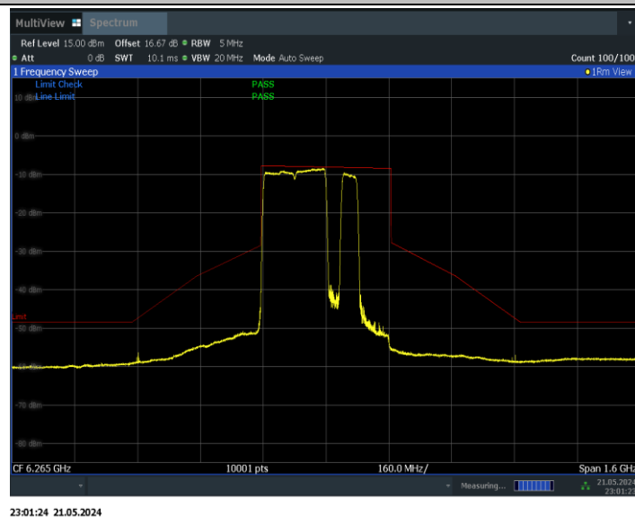
11BE320MIMO_Ant1_6265_2*996+484_Non-OFDMA_5
