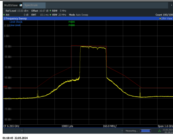
11BE320MIMO_Ant1_6265_3*996_Non-OFDMA_2
