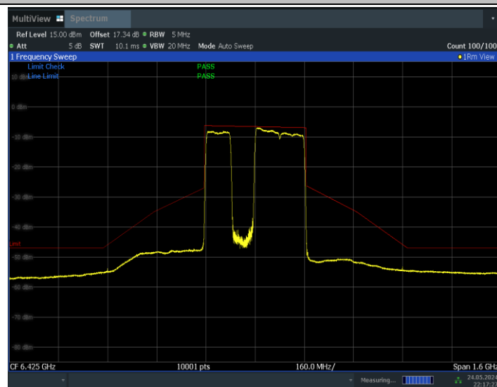
11BE320MIMO_Ant1_6425_3*996_Non-OFDMA_2
