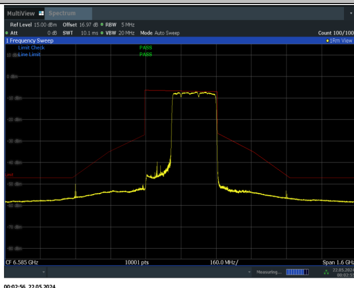
11BE320MIMO_Ant0_6585_2*996+484_Non-OFDMA_8
