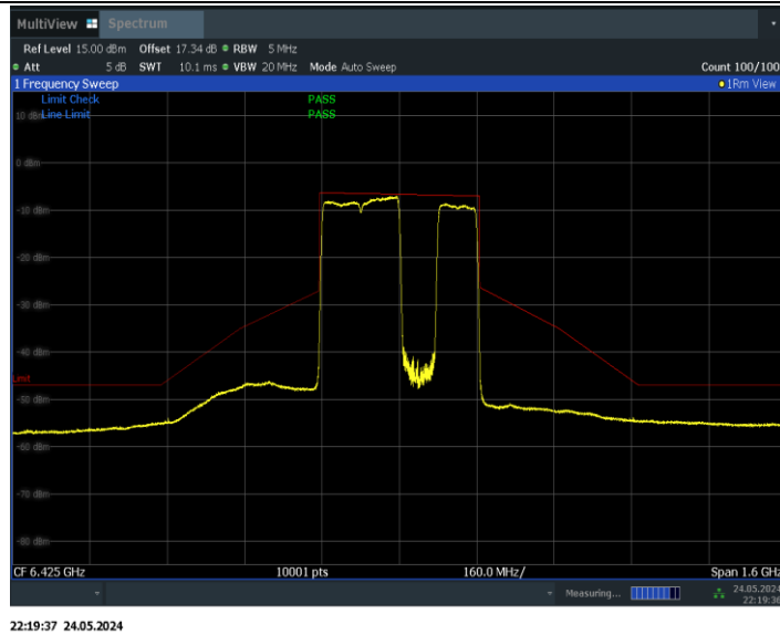
11BE320MIMO_Ant1_6425_3*996_Non-OFDMA_4
