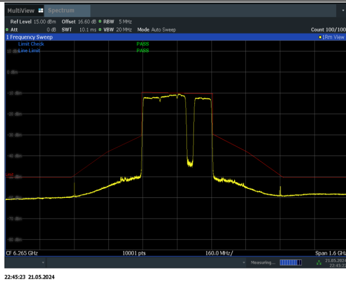
11BE320MIMO_Ant0_6265_3*996+484_Non-OFDMA_7
