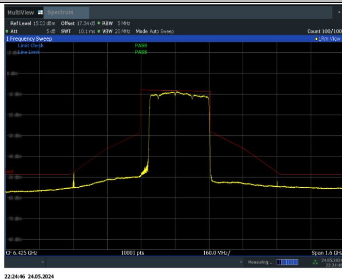
11BE320MIMO_Ant1_6425_3*996+484_Non-OFDMA_1
