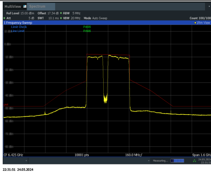
11BE320MIMO_Ant1_6425_3*996+484_Non-OFDMA_5
