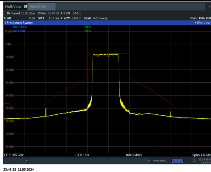
11BE320MIMO_Ant0_6585_2*996+484_Non-OFDMA_2
