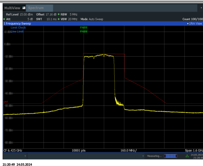
11BE320MIMO_Ant0_6425_3*996_Non-OFDMA_4
