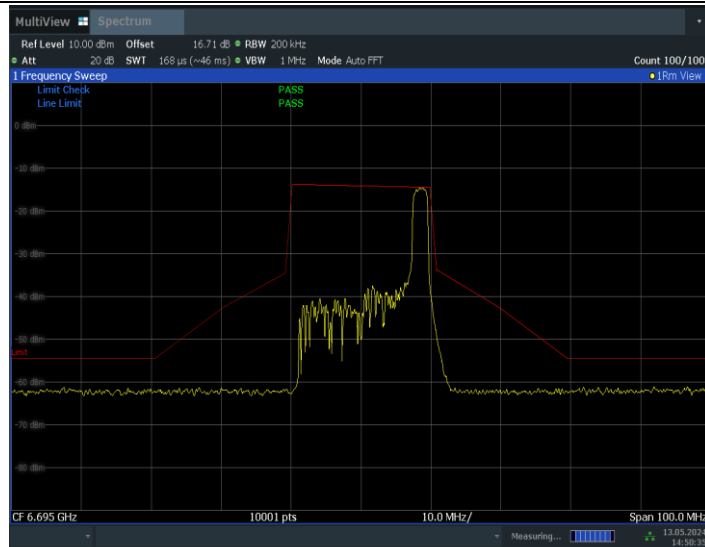
11BE20MIMO_Ant0_6695_52Tone_RU40
