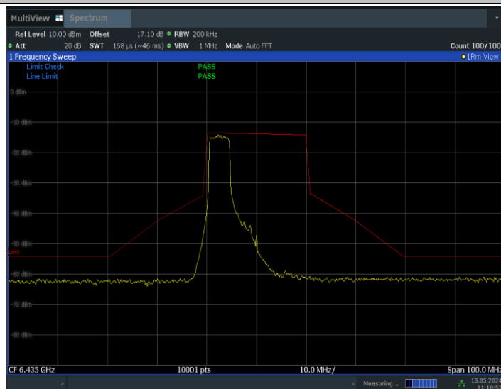
11BE20MIMO_Ant0_6435_52Tone_RU37
