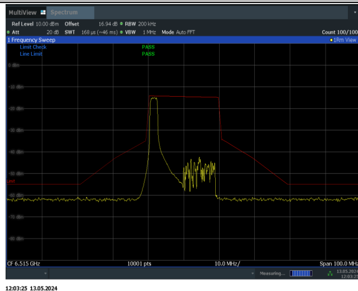
11BE20MIMO_Ant1_6515_52Tone_RU37
