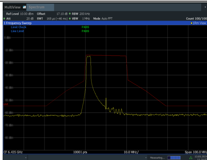
11BE20MIMO_Ant0_6435_26Tone_RU0
