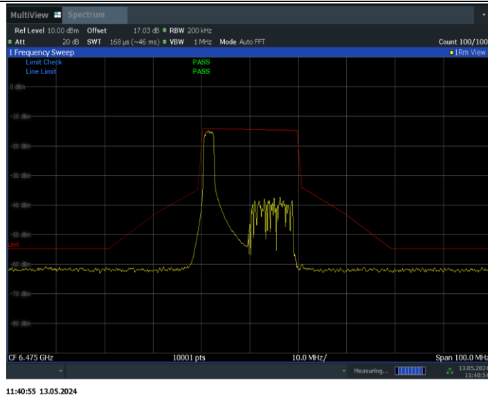
11BE20MIMO_Ant1_6475_52Tone_RU37
