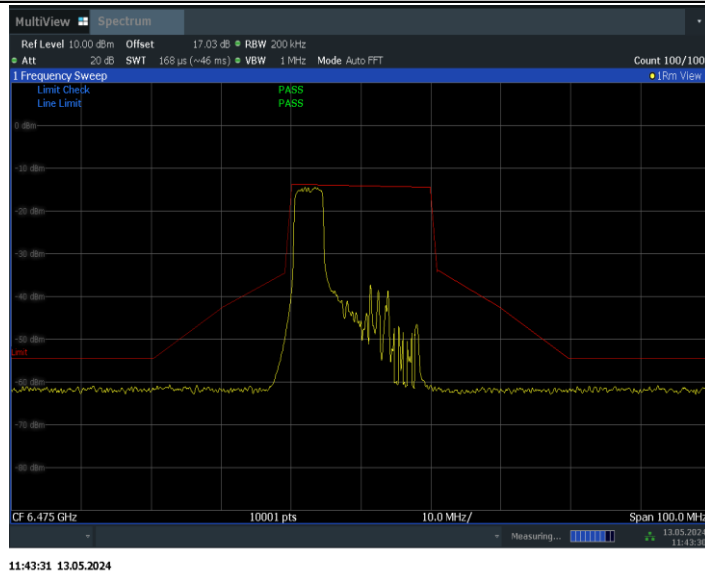
11BE20MIMO_Ant1_6475_106Tone_RU53
