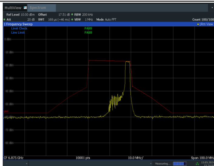
11BE20MIMO_Ant0_6875_26Tone_RU8
