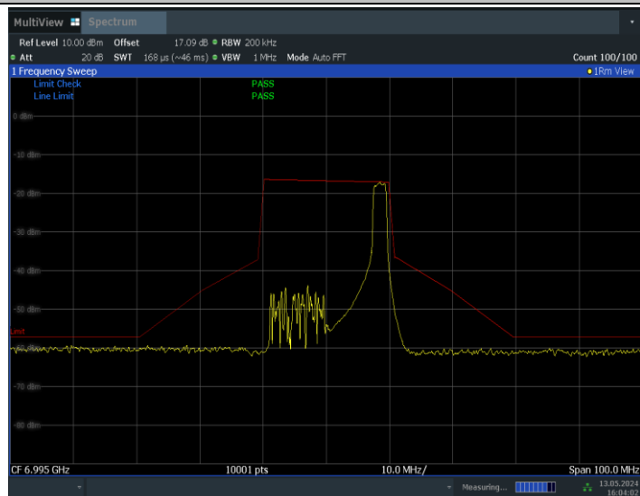
11BE20MIMO_Ant0_6995_26Tone_RU8
