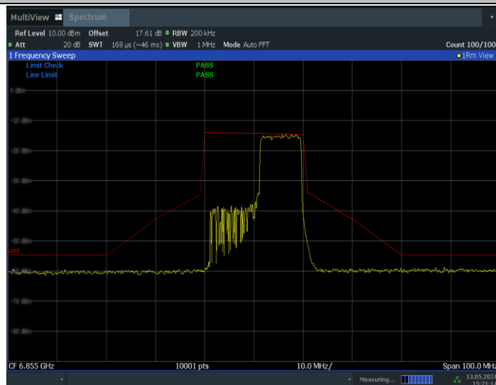
11BE20MIMO_Ant1_6855_106Tone_RU54
