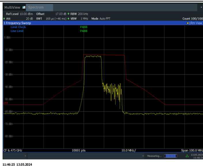
11BE20MIMO_Ant1_6475_106Tone_RU53
