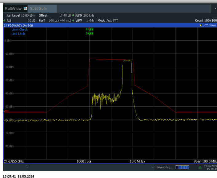
11BE20MIMO_Ant0_6855_52Tone_RU40
