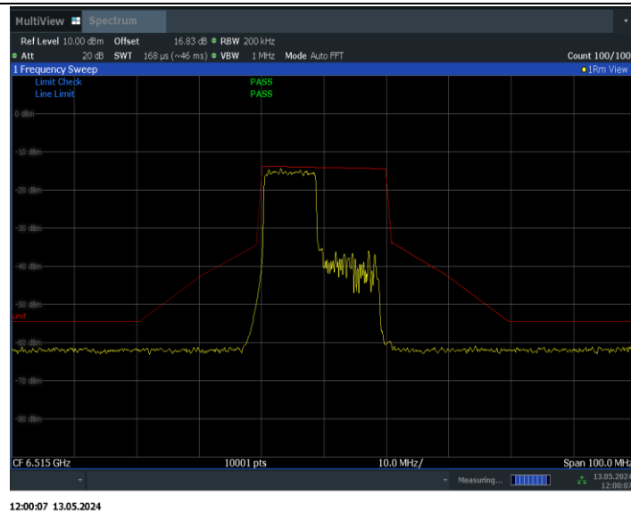
11BE20MIMO_Ant1_6515_26Tone_RU0
