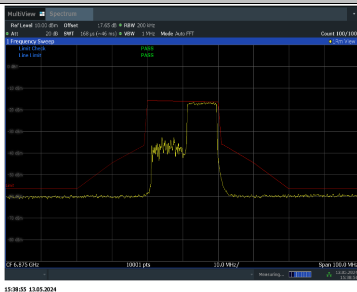
11BE20MIMO_Ant1_6875_106Tone_RU54
