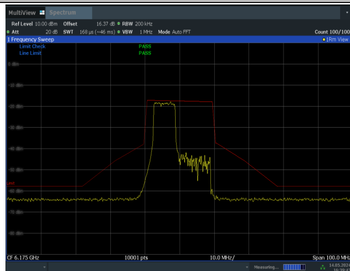
11BE20MIMO_Ant0_6175_52+26_OFDMA_1
