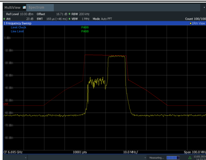
11BE20MIMO_Ant0_6695_106Tone_RU54
