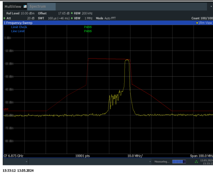
11BE20MIMO_Ant1_6875_52Tone_RU40
