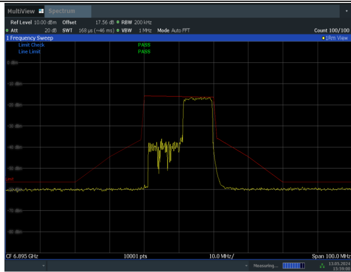
11BE20MIMO_Ant1_6895_106Tone_RU54
