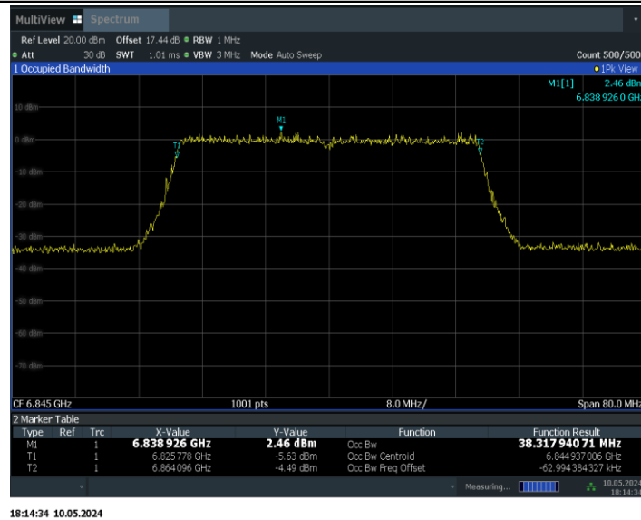
11BE40MIMO_Ant1_6845
