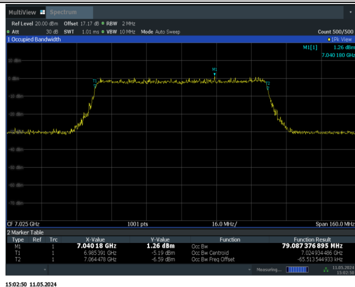
11BE80MIMO_Ant1_7025
