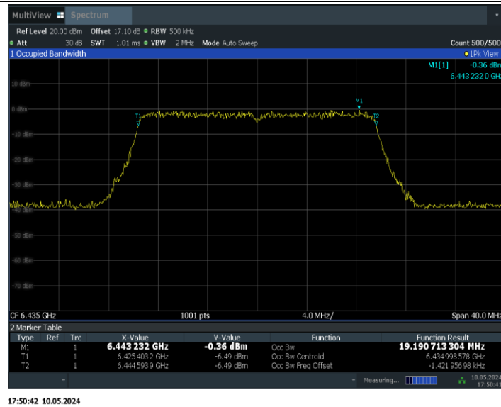
11BE20MIMO_Ant1_6435
