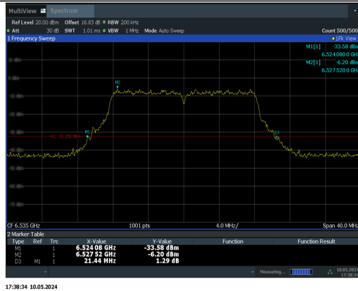
11A-MIMO_Ant1_6535
