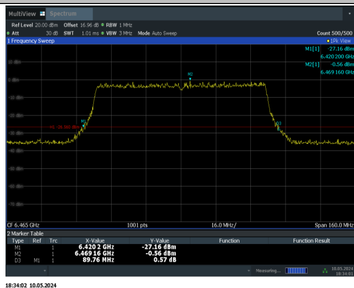
11BE80MIMO_Ant0_6465
