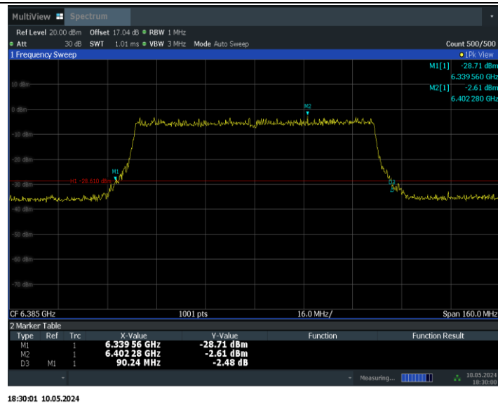
11BE80MIMO_Ant1_6385
