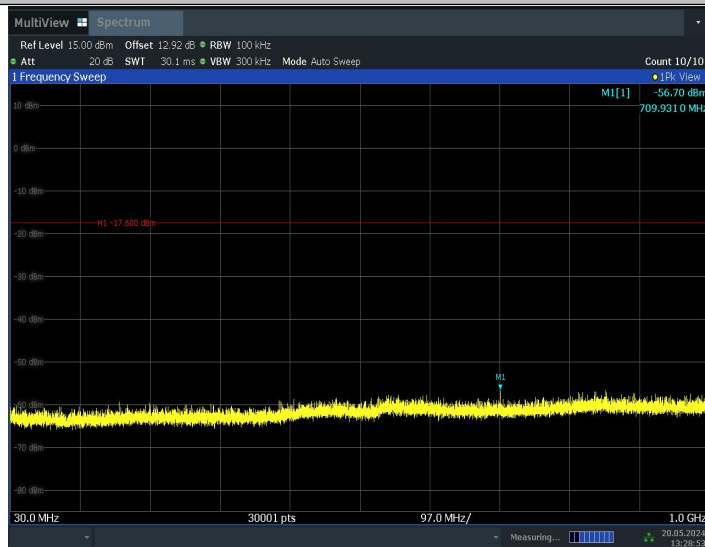
11BE20MIMO_Ant1_2412_52+26_OFDMA_3_30~1000
