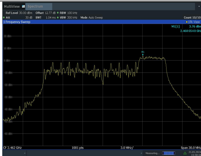
11BE20MIMO_Ant1_2462_52Tone_RU40_0~Reference
