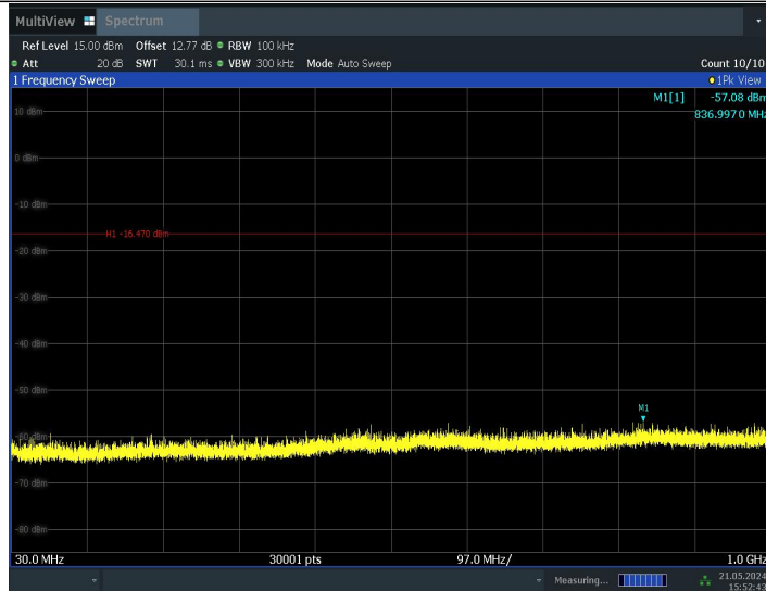
11BE20MIMO_Ant1_2462_106Tone_RU53_30~1000
