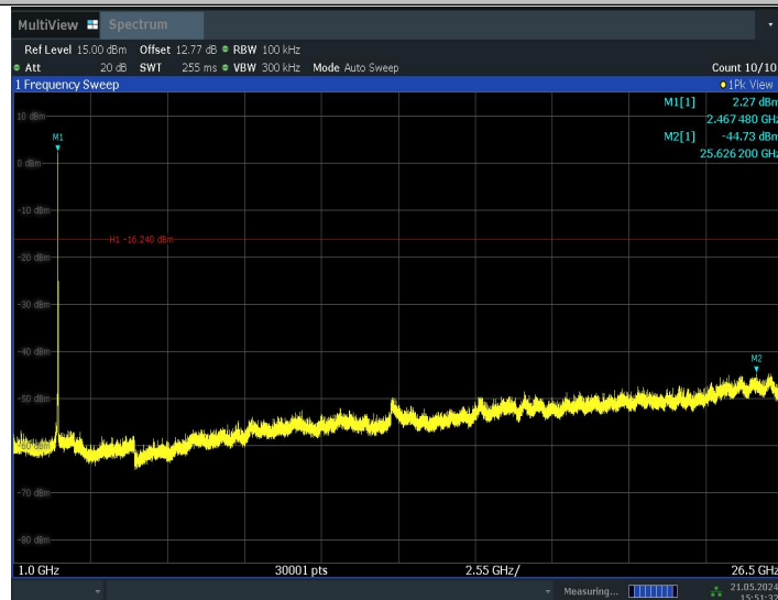
11BE20MIMO_Ant1_2462_52Tone_RU40_1000~26500
