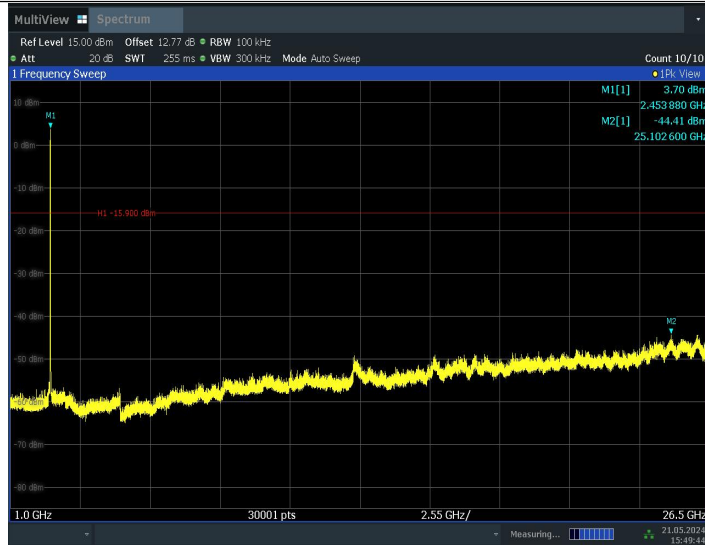
11BE20MIMO_Ant1_2462_52Tone_RU40_0~Reference
