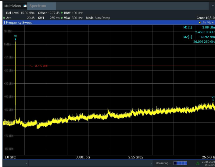
11BE20MIMO_Ant1_2462_106Tone_RU54_0~Reference
