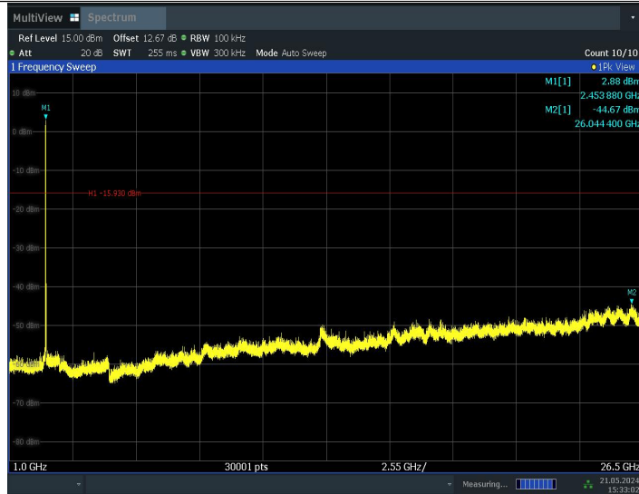
11BE20MIMO_Ant0_2462_26Tone_RU8_0~Reference
