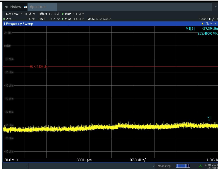
11BE20MIMO_Ant1_2437_52Tone_RU37_30~1000
