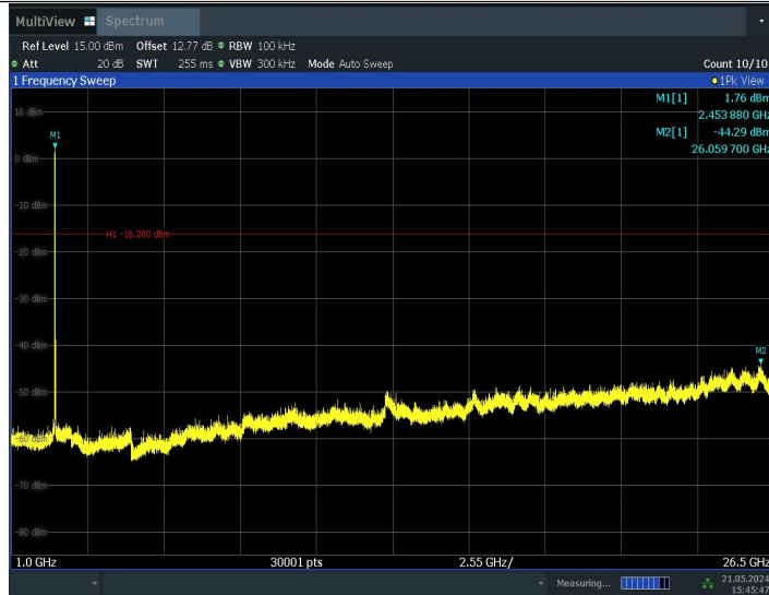
11BE20MIMO_Ant1_2462_26Tone_RU8_0~Reference
