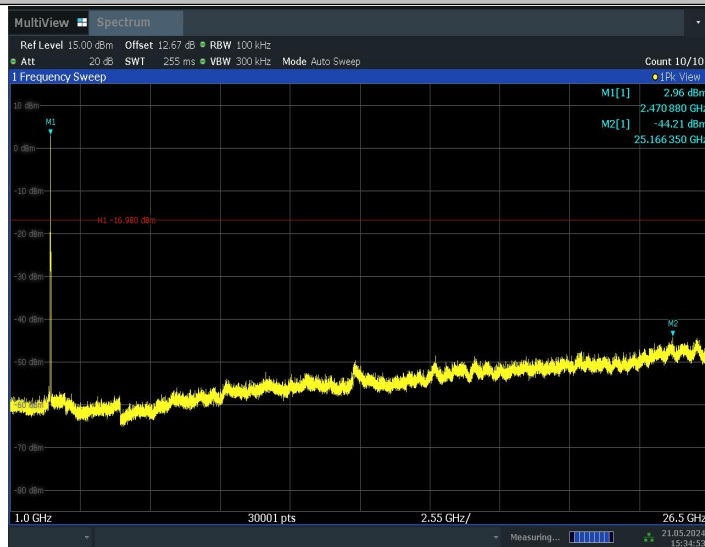
11BE20MIMO_Ant0_2462_26Tone_RU8_1000~26500
