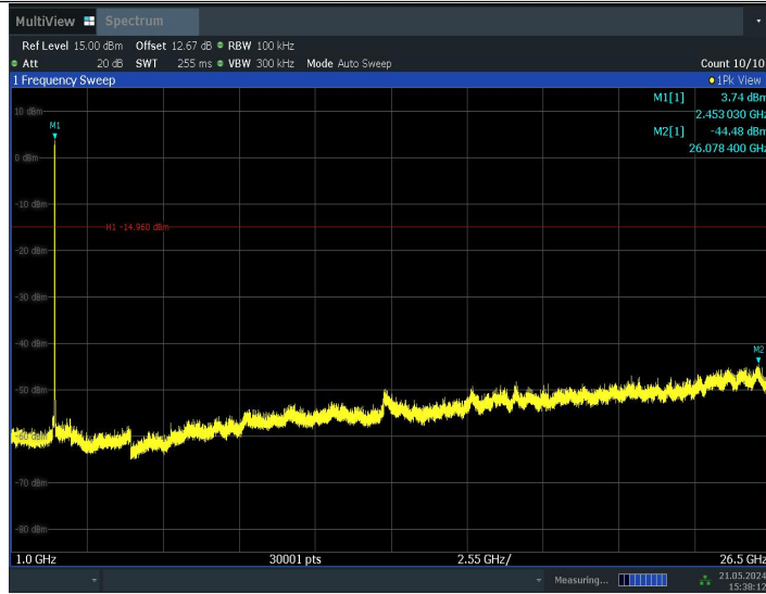
11BE20MIMO_Ant0_2462_52Tone_RU40_0~Reference
