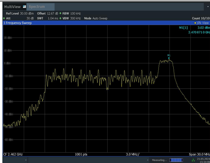
11BE20MIMO_Ant0_2462_26Tone_RU8_0~Reference
