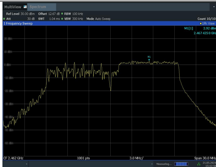
11BE20MIMO_Ant0_2462_106Tone_RU54_0~Reference
