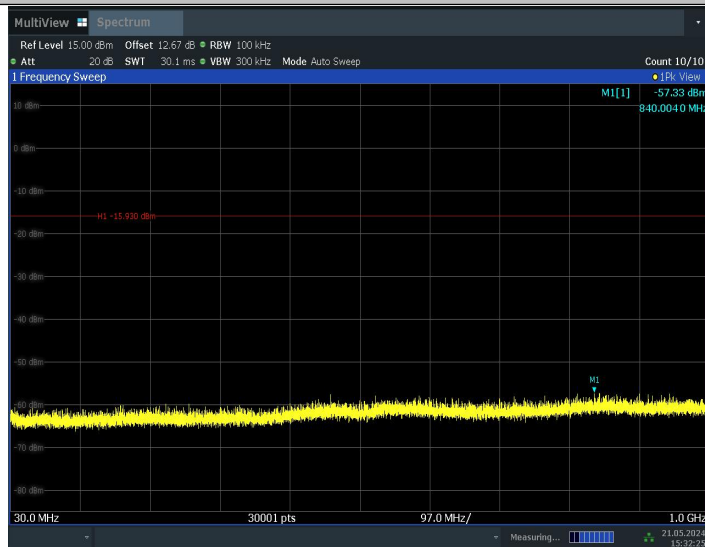
11BE20MIMO_Ant0_2462_26Tone_RU0_30~1000
