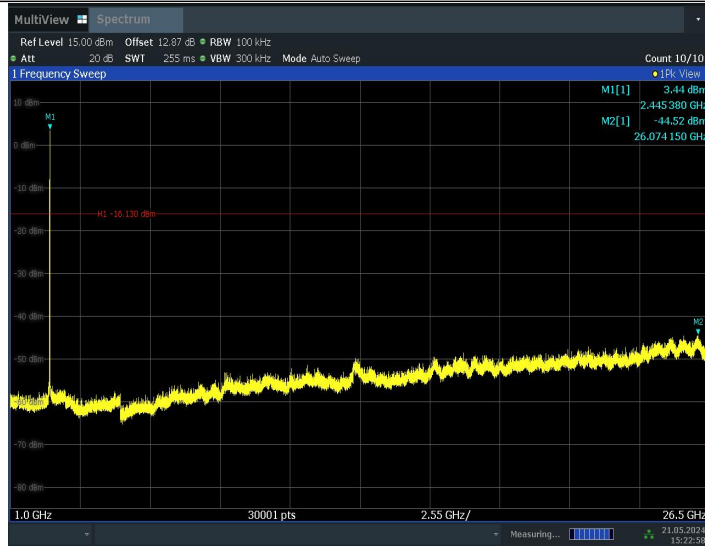
11BE20MIMO_Ant1_2437_26Tone_RU8_1000~26500
