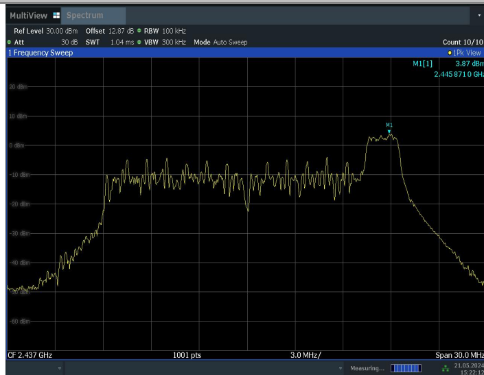
11BE20MIMO_Ant1_2437_26Tone_RU8_0~Reference
