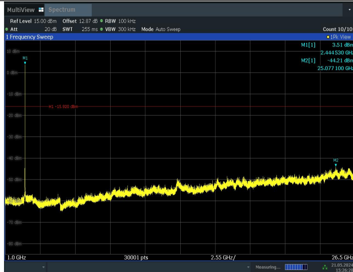
11BE20MIMO_Ant1_2437_52Tone_RU40_1000~26500
