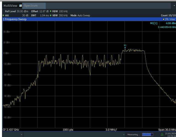
11BE20MIMO_Ant1_2437_52Tone_RU40_0~Reference
