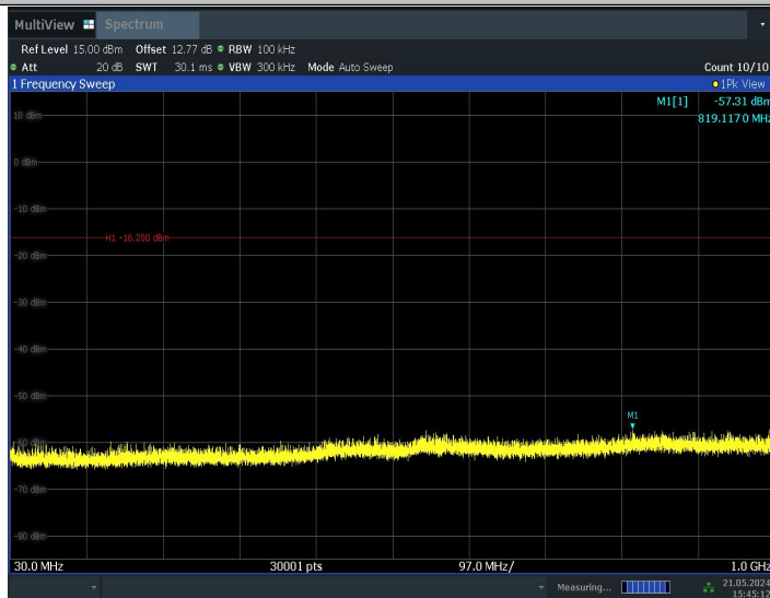
11BE20MIMO_Ant1_2462_26Tone_RU0_30~1000
