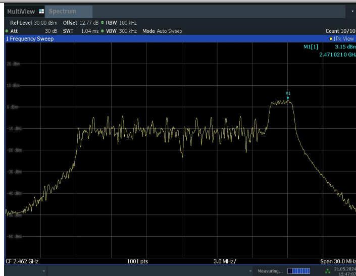
11BE20MIMO_Ant1_2462_26Tone_RU8_0~Reference
