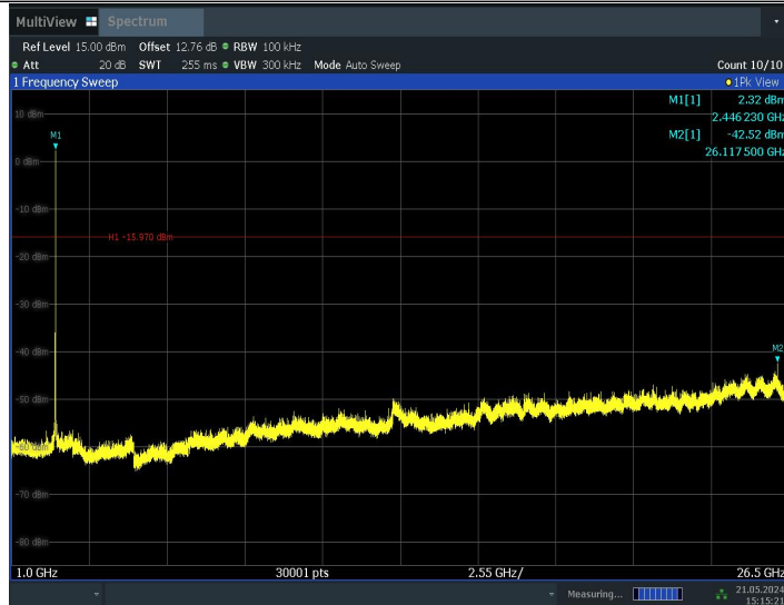
11BE20MIMO_Ant0_2437_52Tone_RU40_1000~26500
