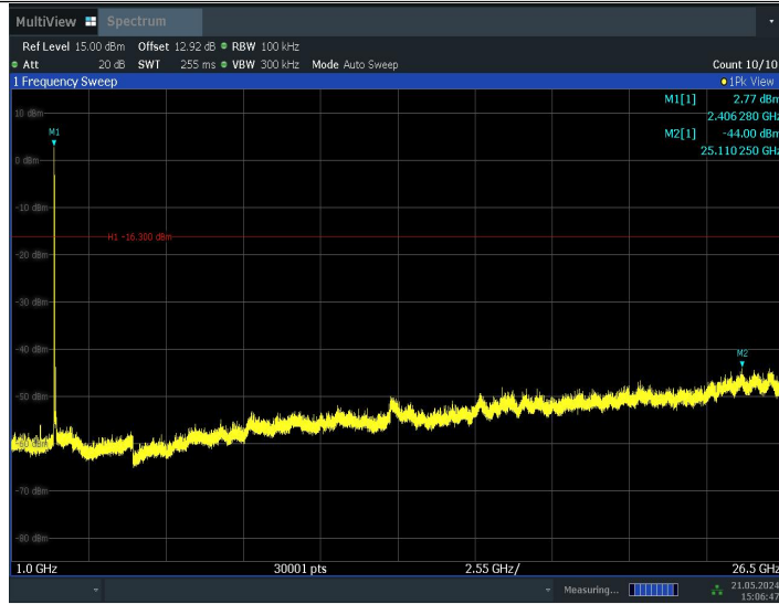
11BE20MIMO_Ant1_2412_106Tone_RU54_0~Reference
