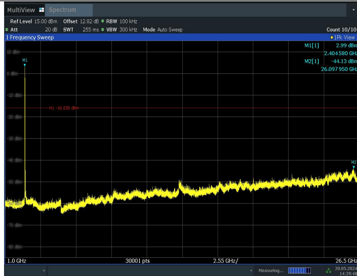
11BE20MIMO_Ant0_2412_106Tone_RU54_0~Reference
