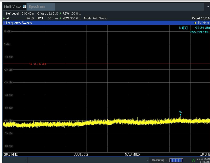
11BE20MIMO_Ant1_2412_52Tone_RU37_30~1000
