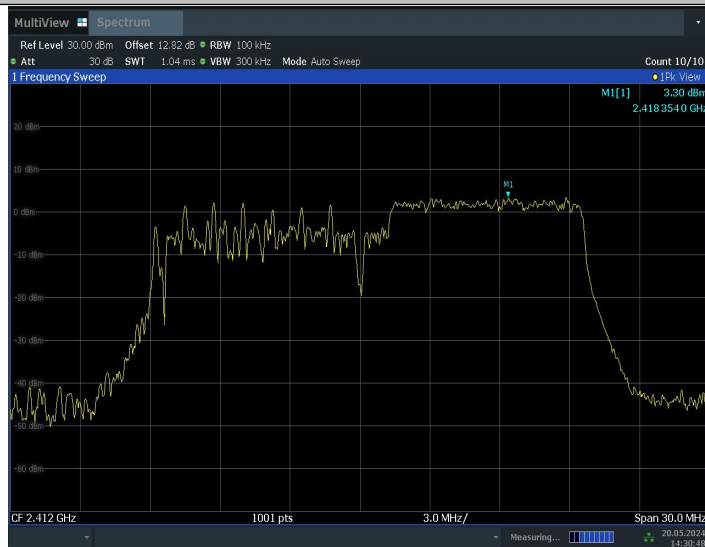
11BE20MIMO_Ant0_2412_106Tone_RU54_0~Reference
