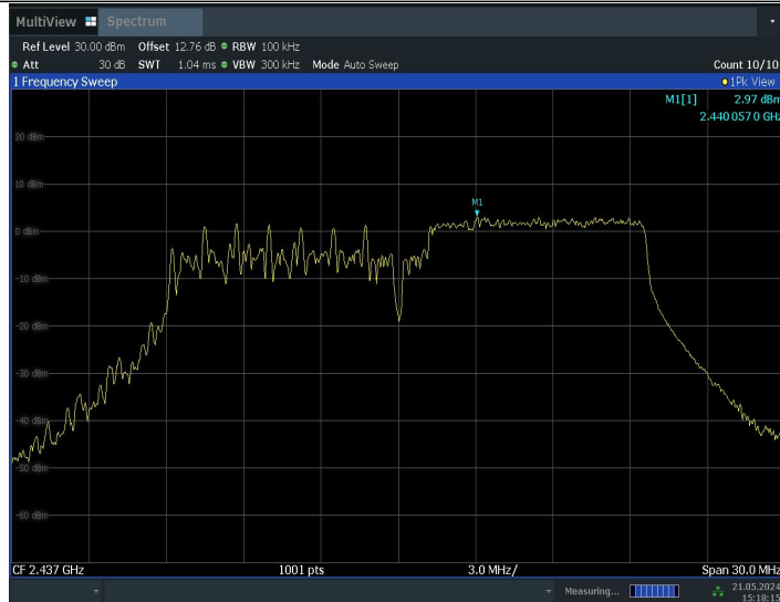
11BE20MIMO_Ant0_2437_106Tone_RU54_0~Reference
