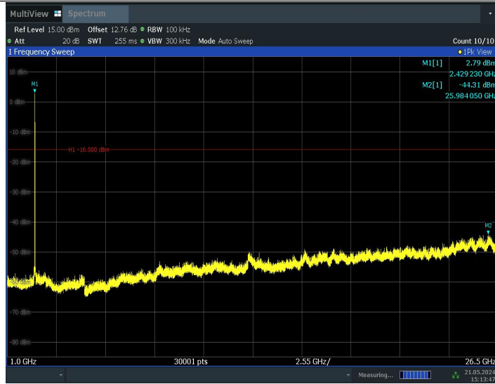
11BE20MIMO_Ant0_2437_52Tone_RU40_0~Reference
