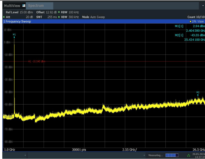
11BE20MIMO_Ant1_2412_52Tone_RU40_0~Reference
