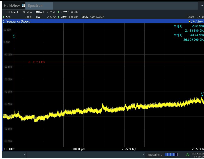
11BE20MIMO_Ant0_2437_26Tone_RU8_0~Reference
