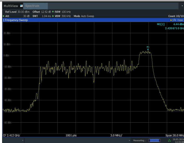
11BE20MIMO_Ant1_2412_26Tone_RU8_0~Reference
