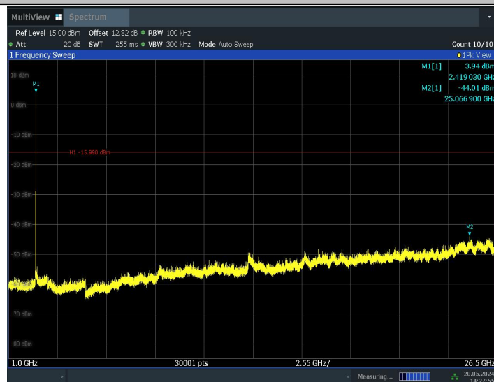
11BE20MIMO_Ant0_2412_52Tone_RU40_1000~26500
