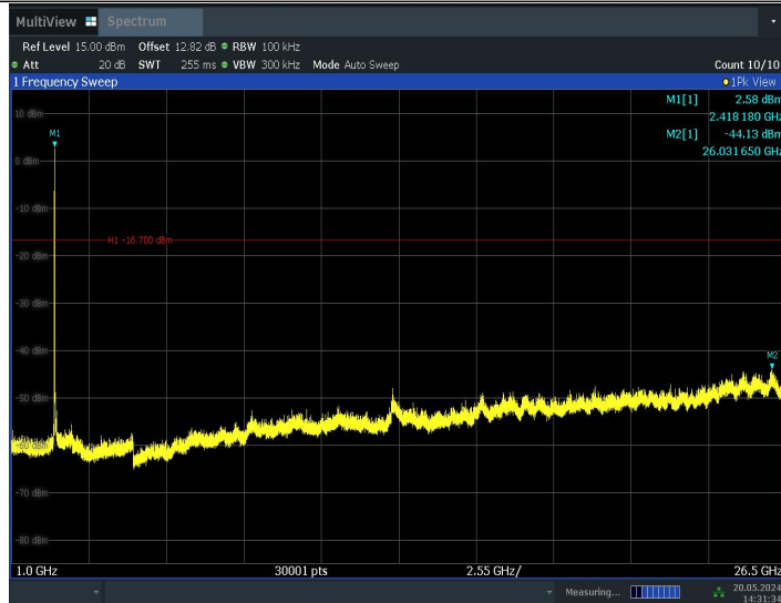
11BE20MIMO_Ant0_2412_106Tone_RU54_1000~26500
