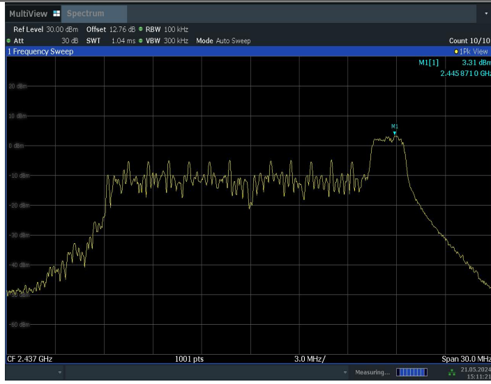
11BE20MIMO_Ant0_2437_26Tone_RU8_0~Reference
