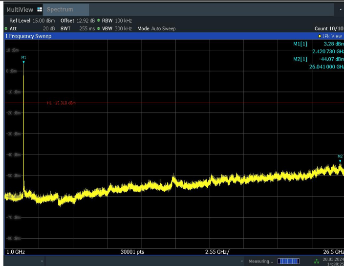
11BE20MIMO_Ant1_2412_52Tone_RU40_1000~26500
