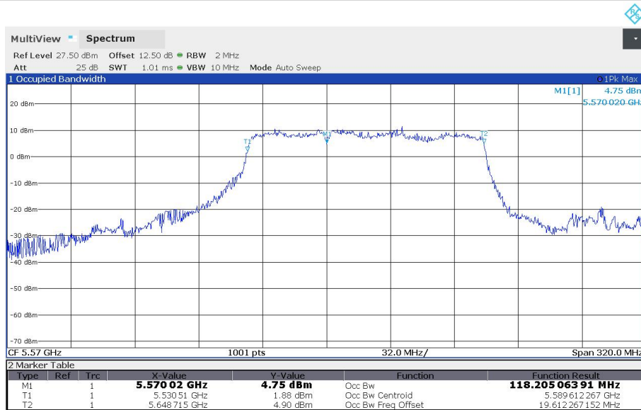
11BE160MIMO_Ant0_5570_Puncturing 40M_2
