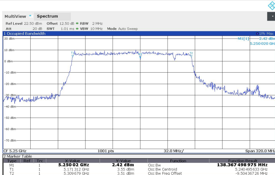
11BE160MIMO_Ant1_5250_Puncturing 40M_3
