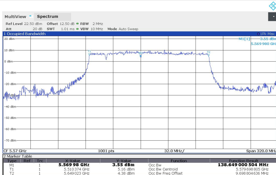
11BE160MIMO_Ant1_5570_Puncturing 20M_2
