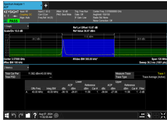
N48(40M)_DFT-s-OFDM_PI_2-BPSK_Edge_1RB_Left_Low_CH
