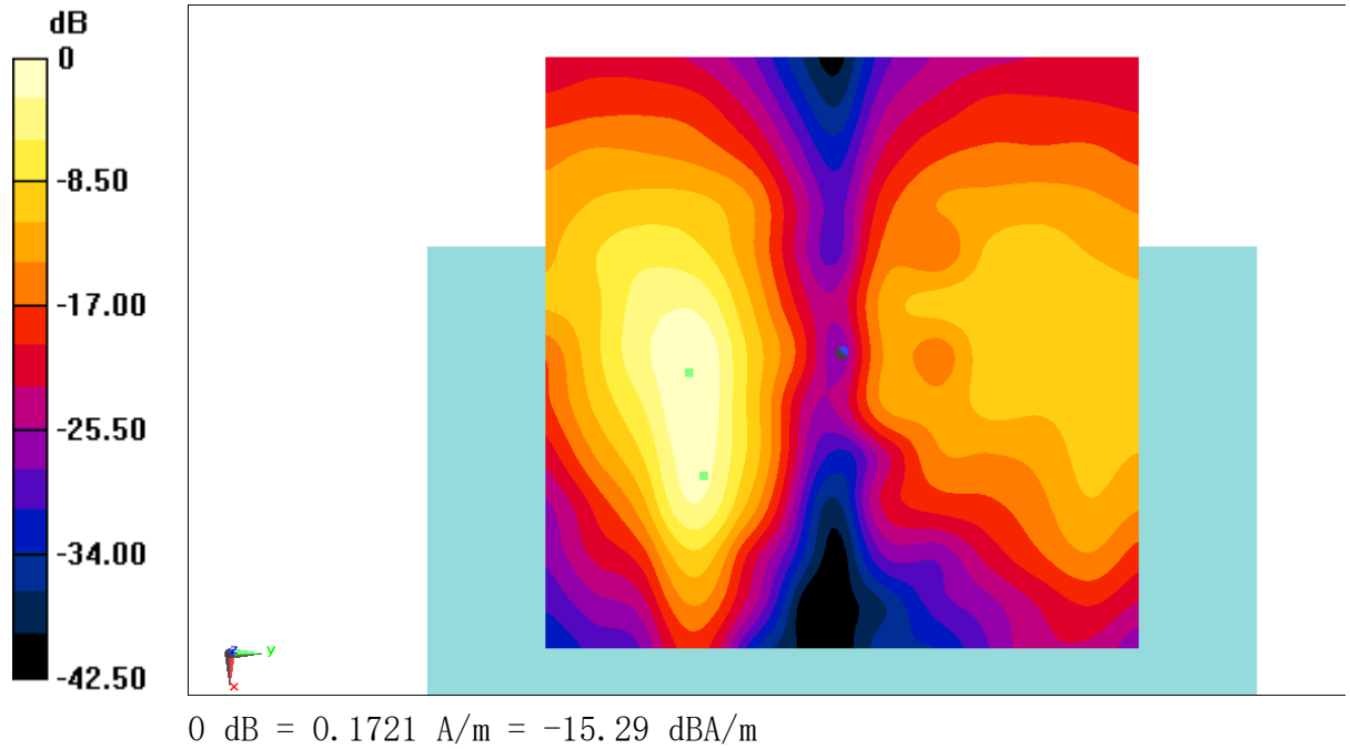
Fig B.7 T-Coil WiFi-2. 4G
