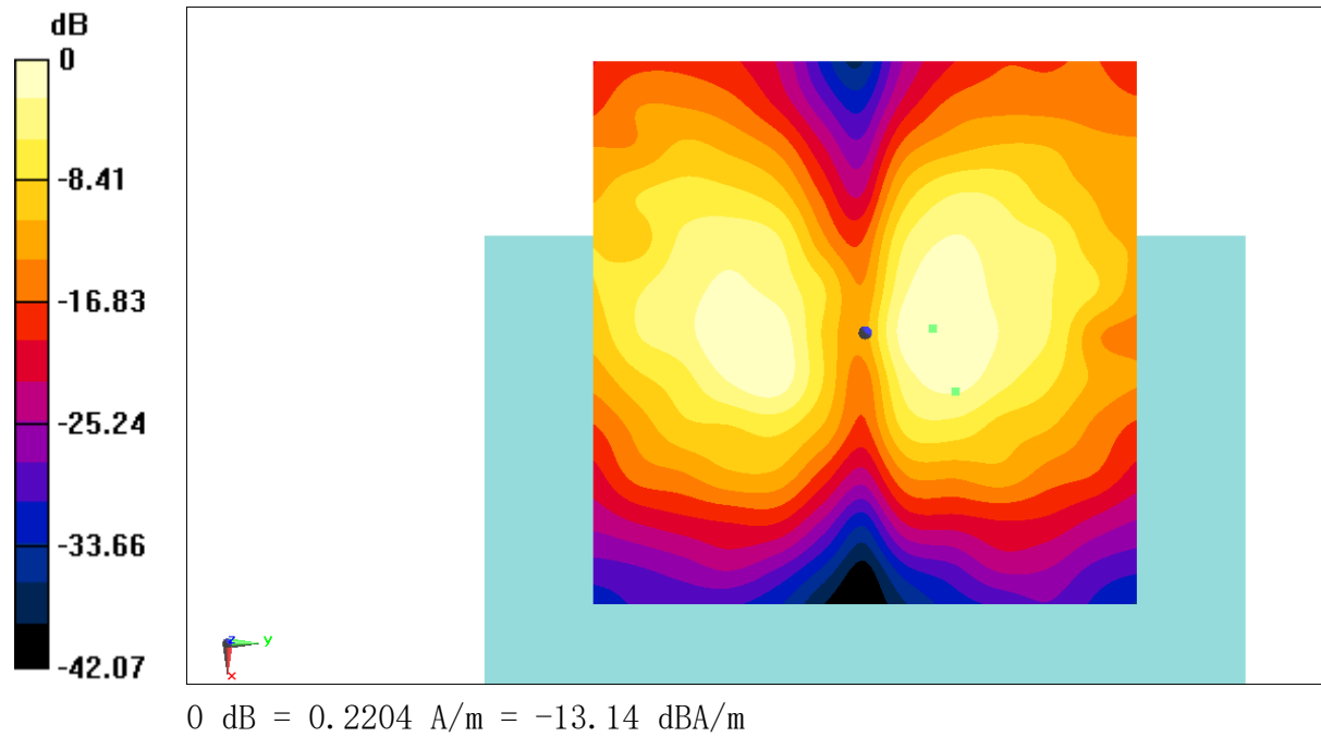
Fig B.11 T-Coil WCDMA 850
