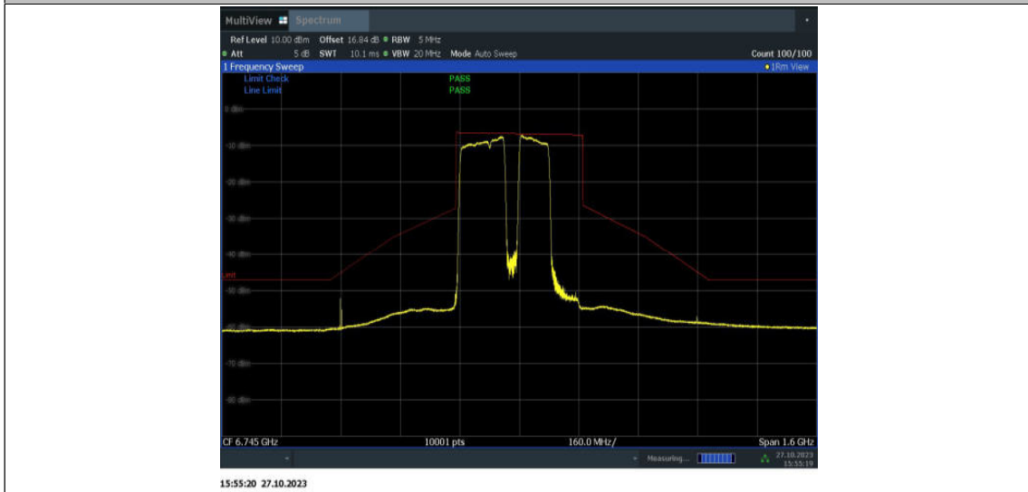
11BE320MIMO_Ant9_6745_2*996+484_OFDMA_5
