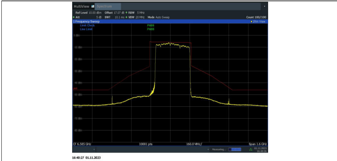
11BE320MIMO_Ant15_6585_3*996+484_OFDMA_2
