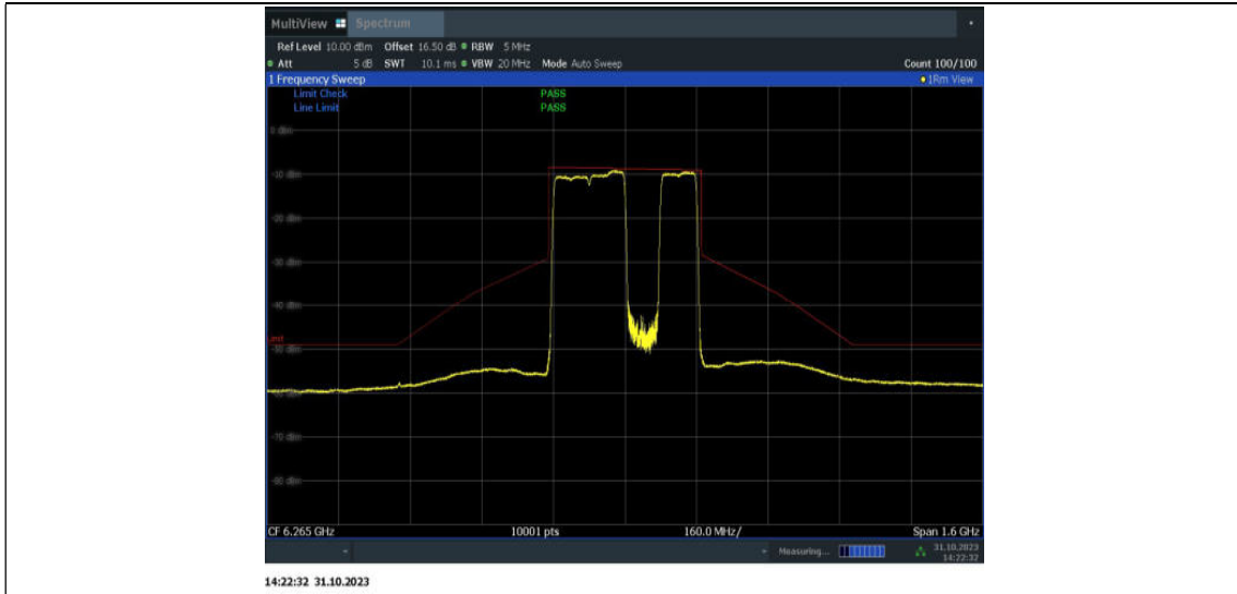
11BE320MIMO_Ant9_6265_3*996_OFDMA_4
