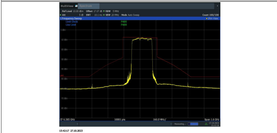
11BE320MIMO_Ant15_6585_3*996_OFDMA_1
