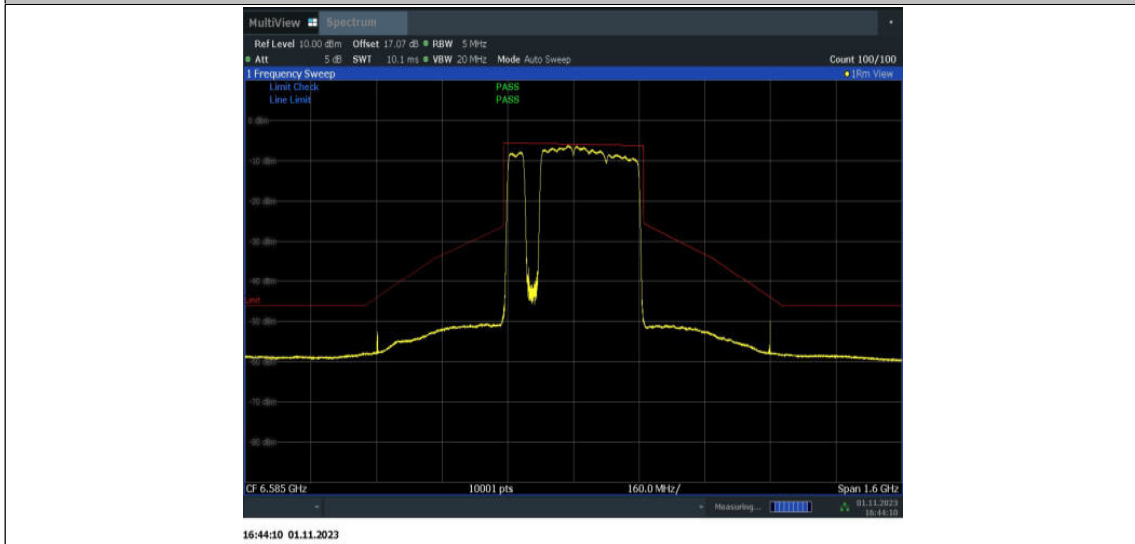
11BE320MIMO_Ant15_6585_3*996+484_OFDMA_3
