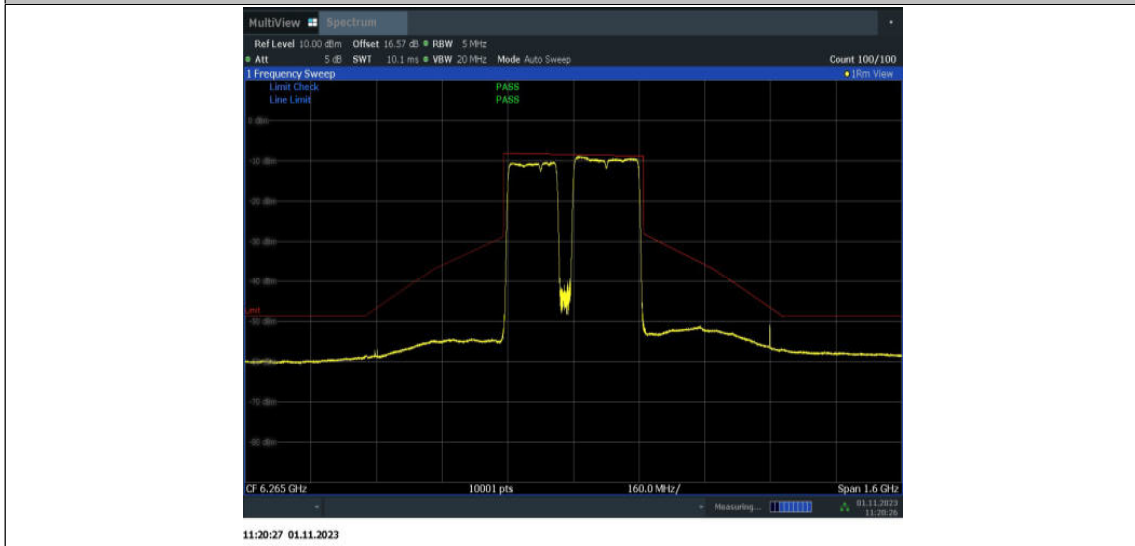
11BE320MIMO_Ant15_6265_3*996+484_OFDMA_5
