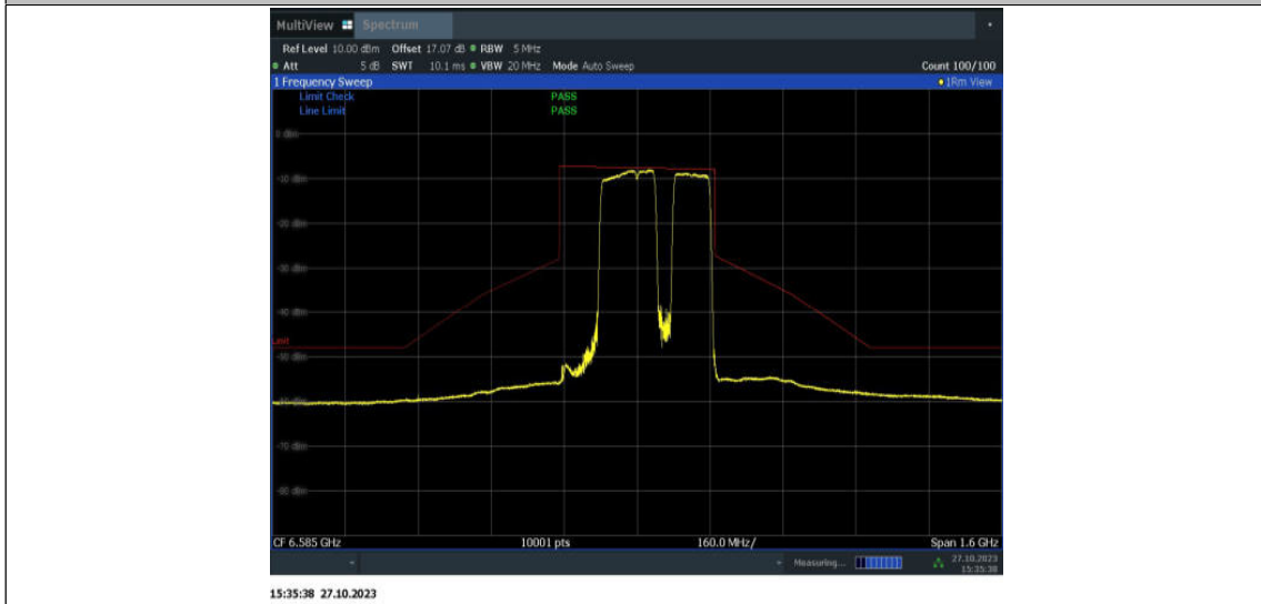
11BE320MIMO_Ant15_6585_2*996+484_OFDMA_11
