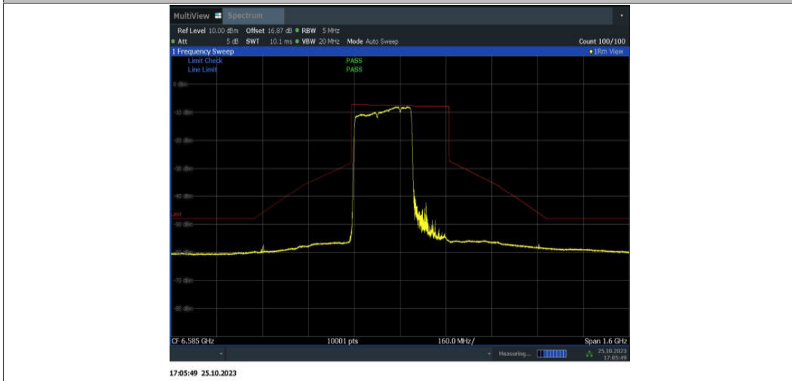
11BE320MIMO_Ant9_6585_2*996+484_OFDMA_7
