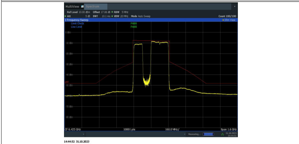
11BE320MIMO_Ant9_6425_3*996_OFDMA_3
