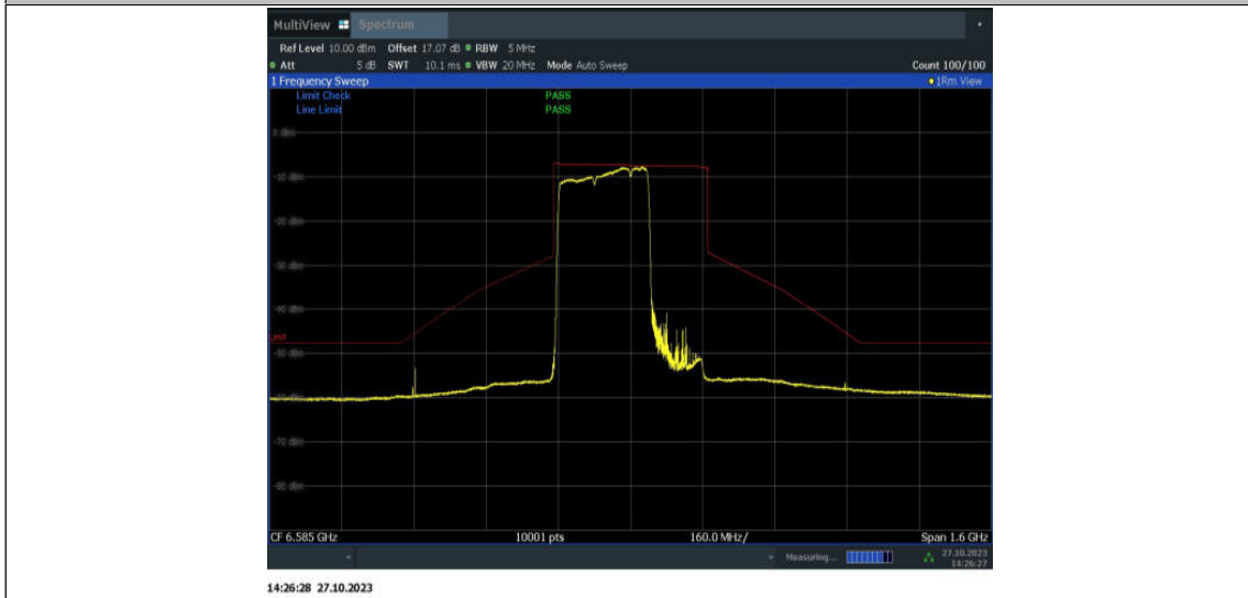
11BE320MIMO_Ant15_6585_2*996+484_OFDMA_7
