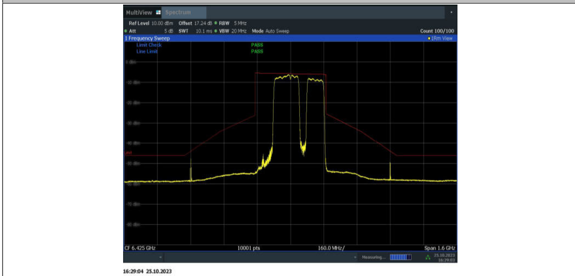
11BE320MIMO_Ant15_6425_2*996+484_OFDMA_11
