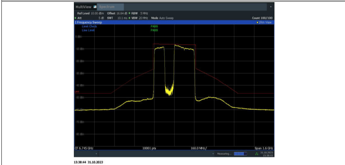
11BE320MIMO_Ant9_6745_3*996_OFDMA_3
