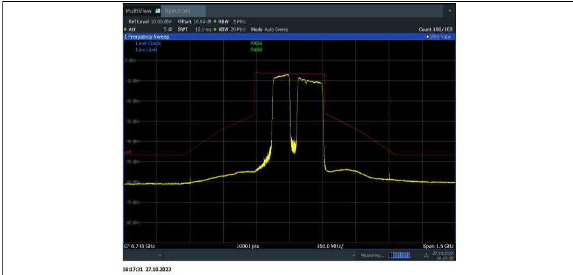
11BE320MIMO_Ant9_6745_2*996+484_OFDMA_10
