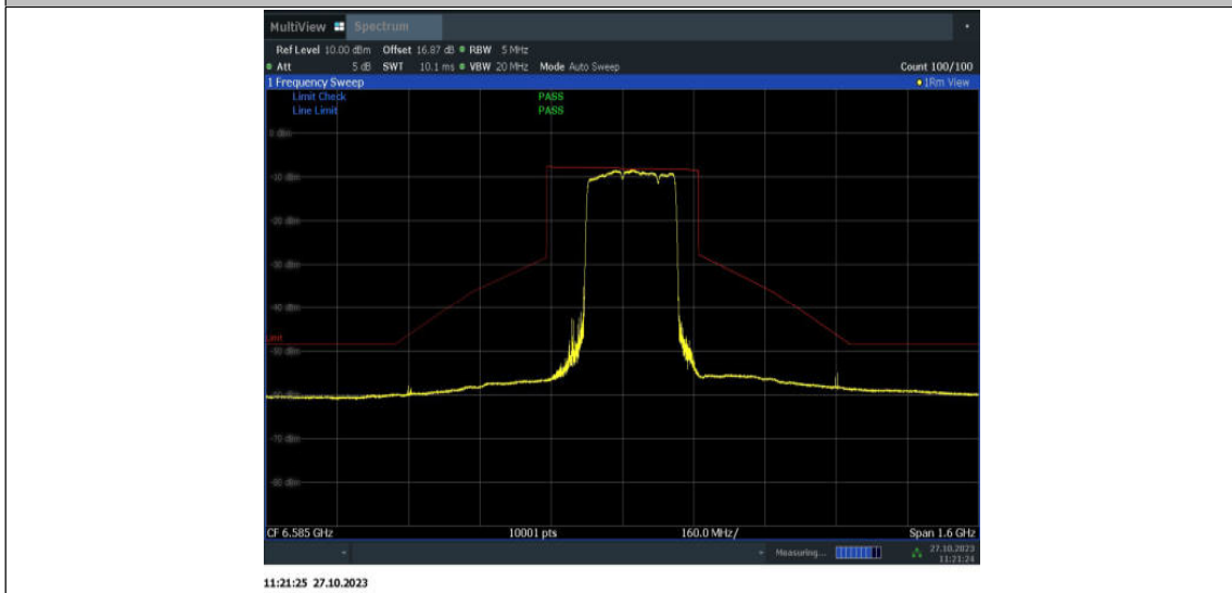
11BE320MIMO_Ant9_6585_3*996_OFDMA_1
