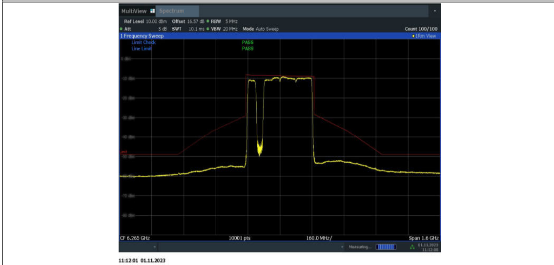
11BE320MIMO_Ant15_6265_3*996+484_OFDMA_3
