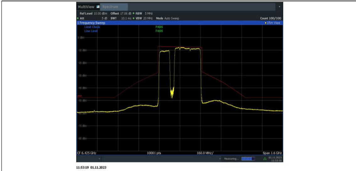
11BE320MIMO_Ant9_6425_3*996+484_OFDMA_4
