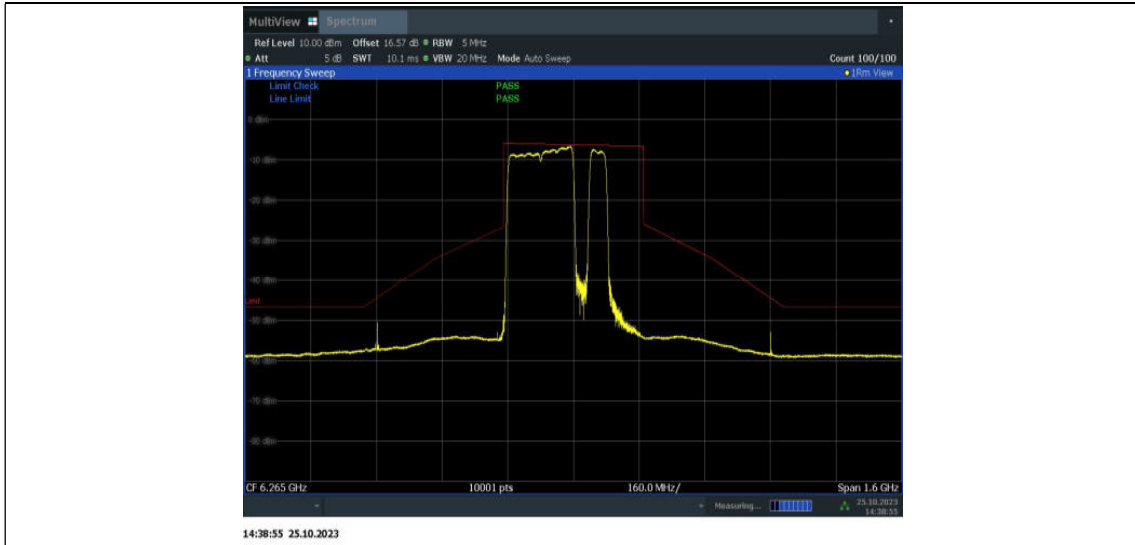
11BE320MIMO_Ant15_6265_2*996+484_OFDMA_6
