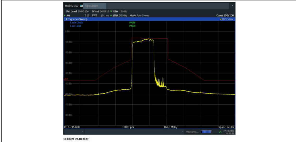
11BE320MIMO_Ant9_6745_2*996+484_OFDMA_7
