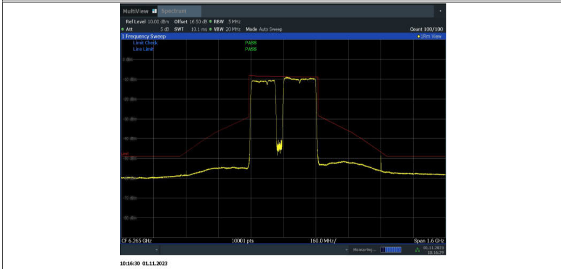
11BE320MIMO_Ant9_6265_3*996+484_OFDMA_5
