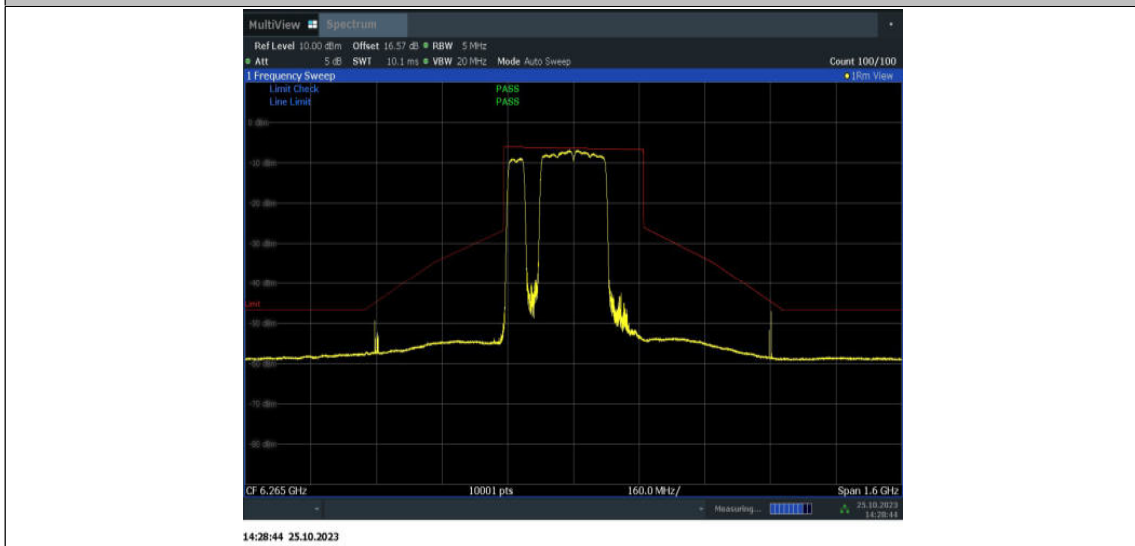
11BE320MIMO_Ant15_6265_2*996+484_OFDMA_3
