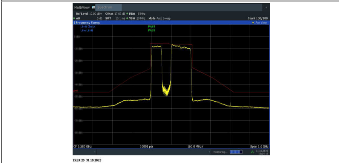
11BE320MIMO_Ant15_6585_3*996_OFDMA_3
