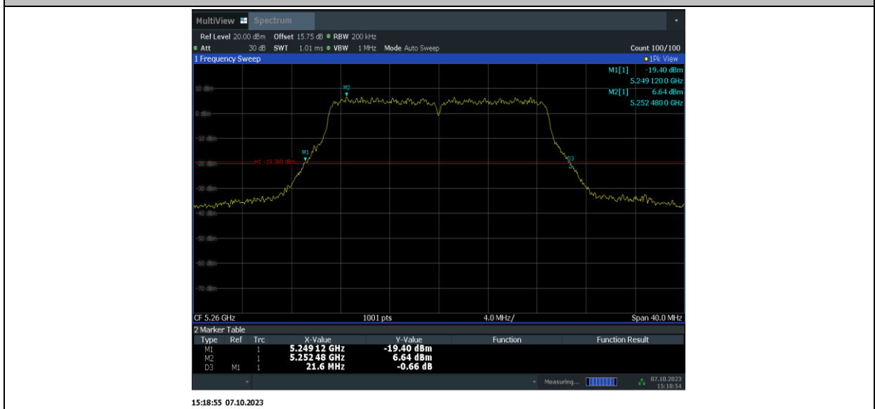
11N20MIMO_Ant9_5260
