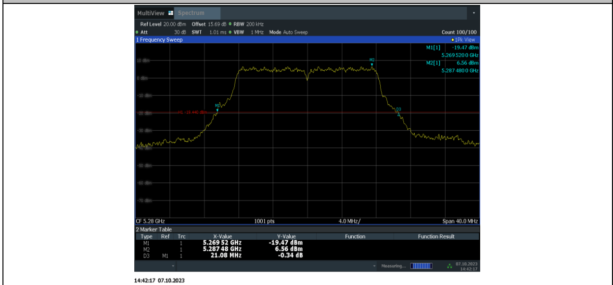
11A-MIMO_Ant15_5280
