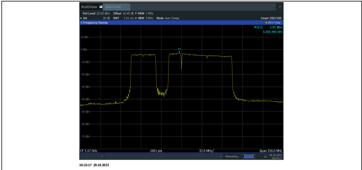
11BE160MIMO_Ant15_5570_996+484+242_OFDMA_4
