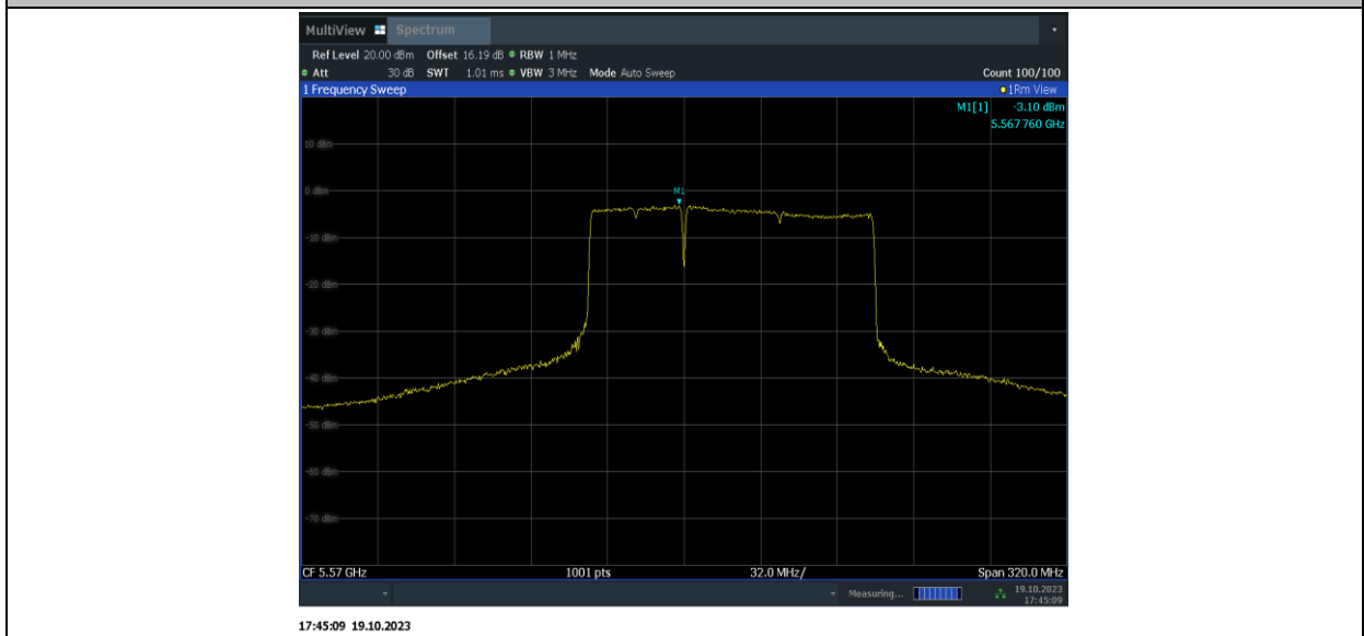
11BE160MIMO_Ant9_5570_996+484_OFDMA_1
