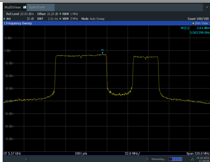
11BE160MIMO_Ant9_5570_996+484_OFDMA_3
