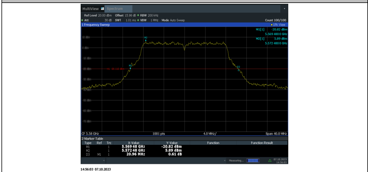
11A-MIMO_Ant9_5580
