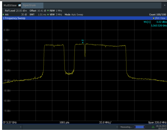
11BE160MIMO_Ant9_5570_996+484+242_OFDMA_3
