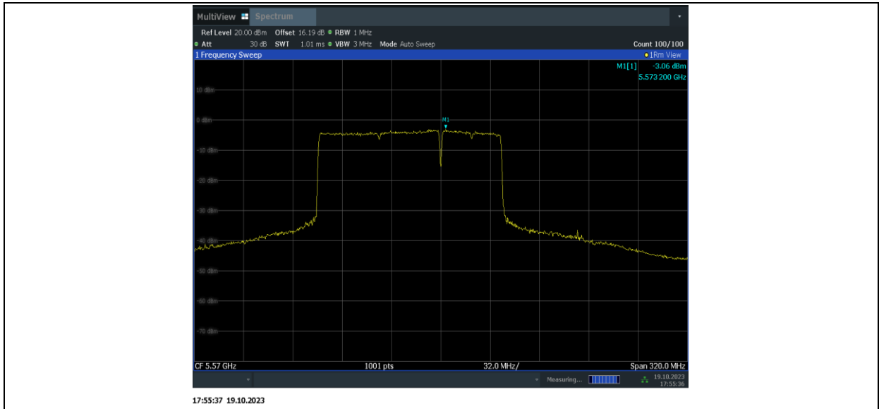
11BE160MIMO_Ant9_5570_996+484+242_OFDMA_1
