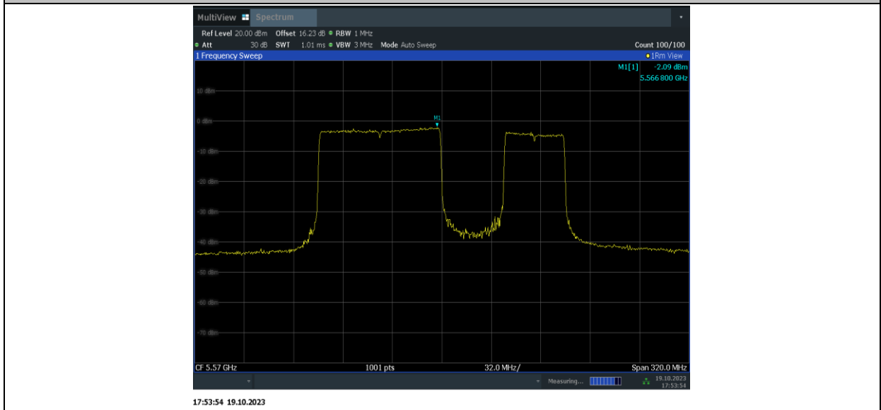
11BE160MIMO_Ant15_5570_996+484_OFDMA_4
