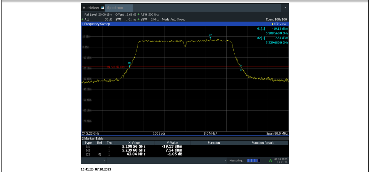
11N40MIMO_Ant15_5230
