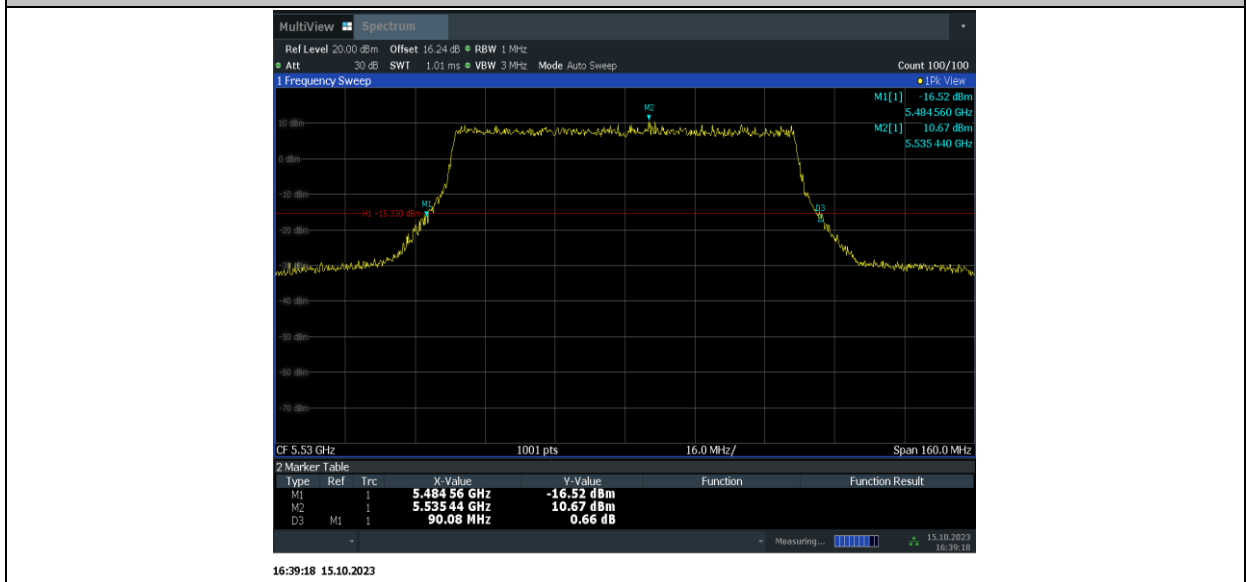
11BE80MIMO_Ant15_5530
