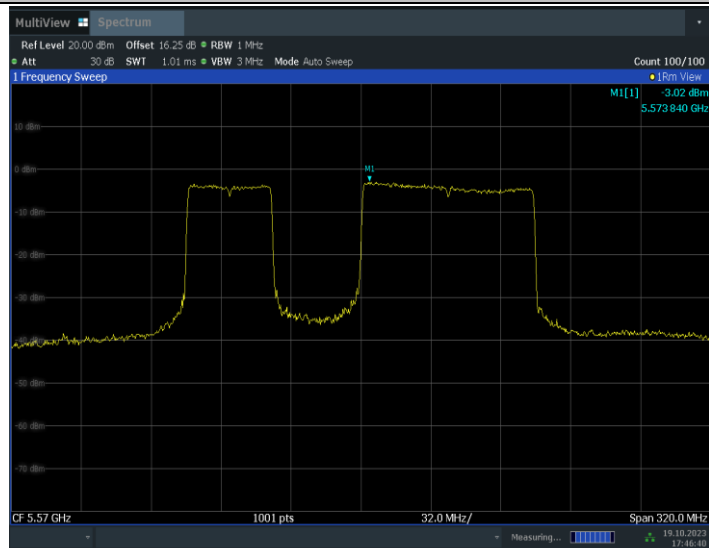
11BE160MIMO_Ant9_5570_996+484_OFDMA_2
