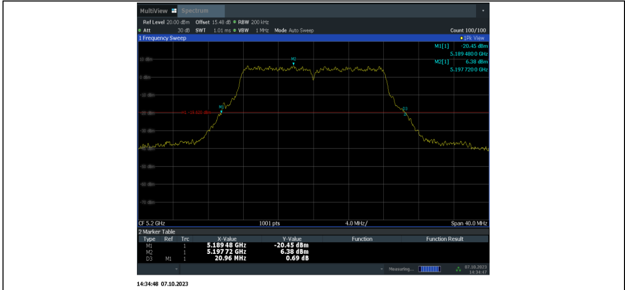
11A-MIMO_Ant15_5200
