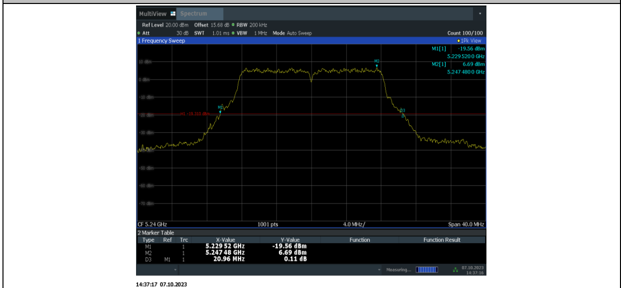
11A-MIMO_Ant9_5240
