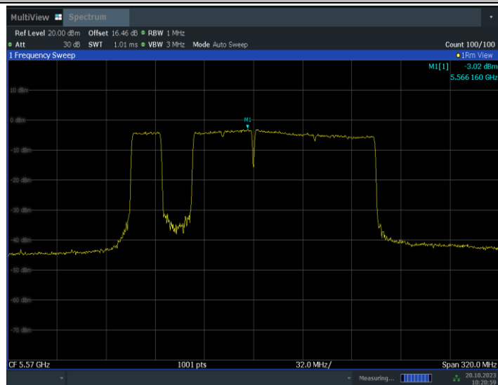
11BE160MIMO_Ant15_5570_996+484+242_OFDMA_2
