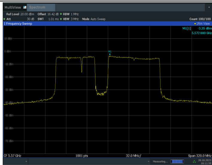
11BE160MIMO_Ant9_5570_996+484+242_OFDMA_4
