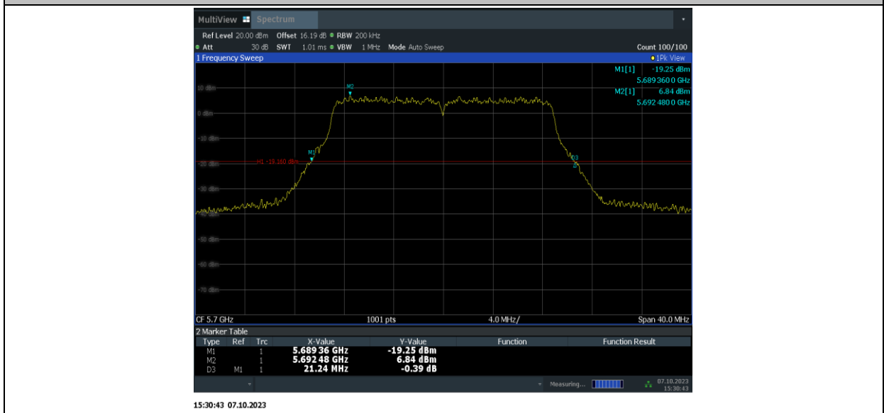
11N20MIMO_Ant9_5700
