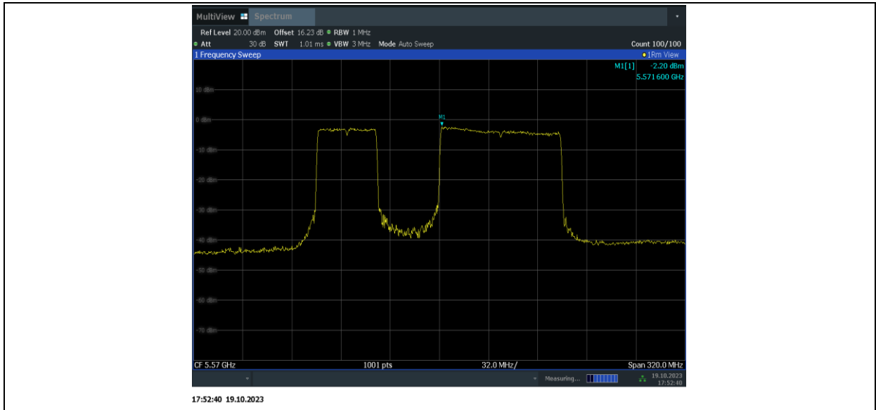
11BE160MIMO_Ant15_5570_996+484_OFDMA_3
