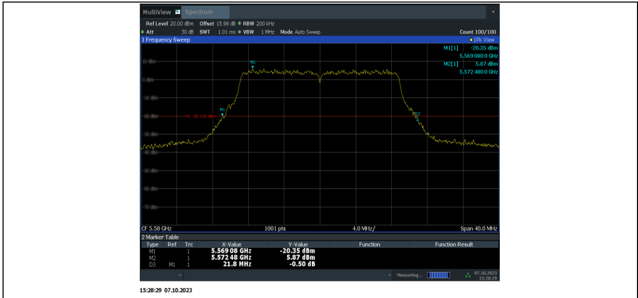
11N20MIMO_Ant15_5580
