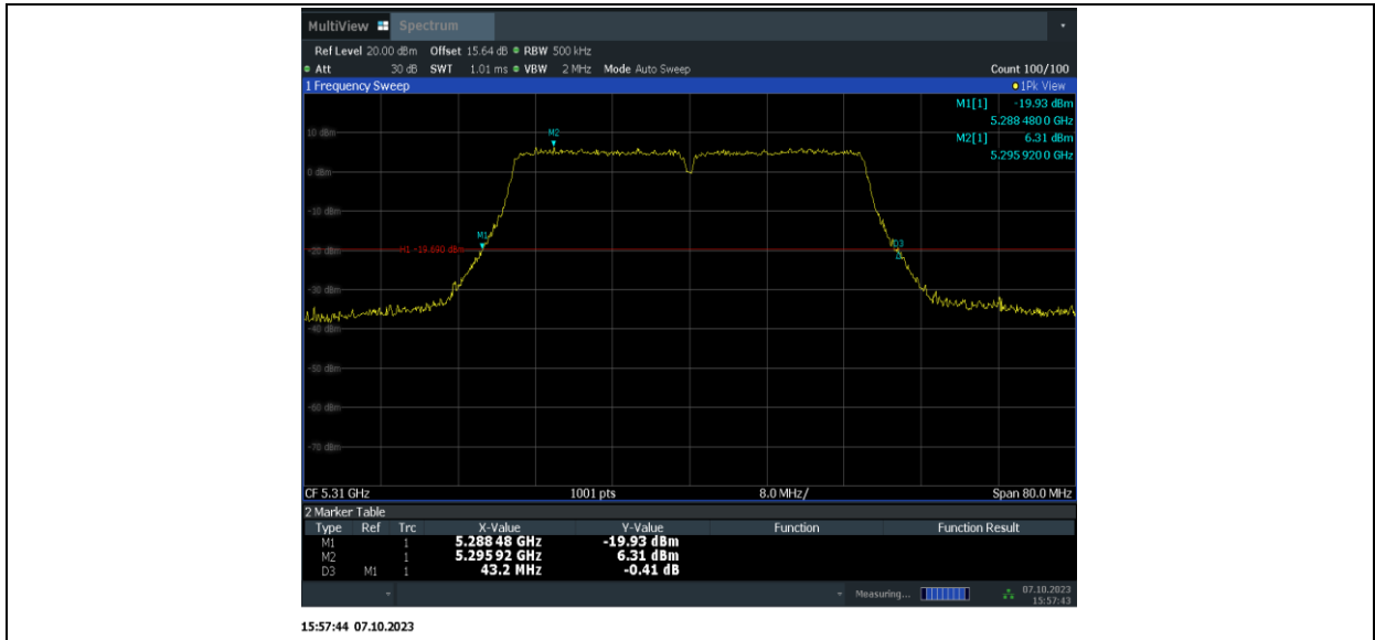
11N40MIMO_Ant15_5310
