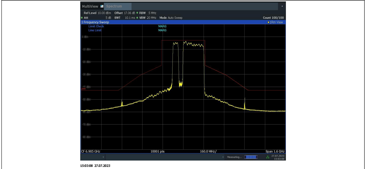
11BE320MIMO_Ant1_6905_996+996+484_9
