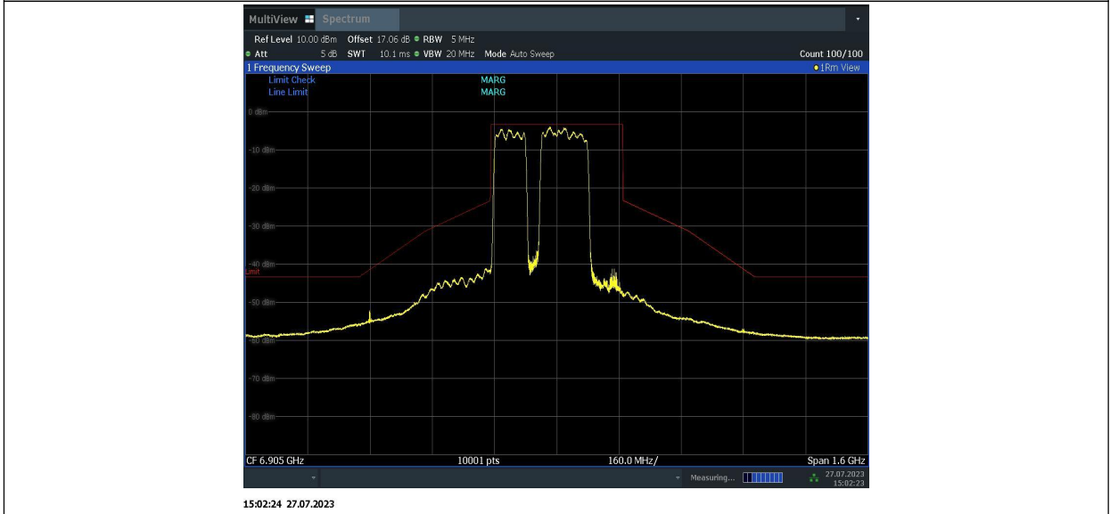
11BE320MIMO_Ant1_6905_996+996+484_4
