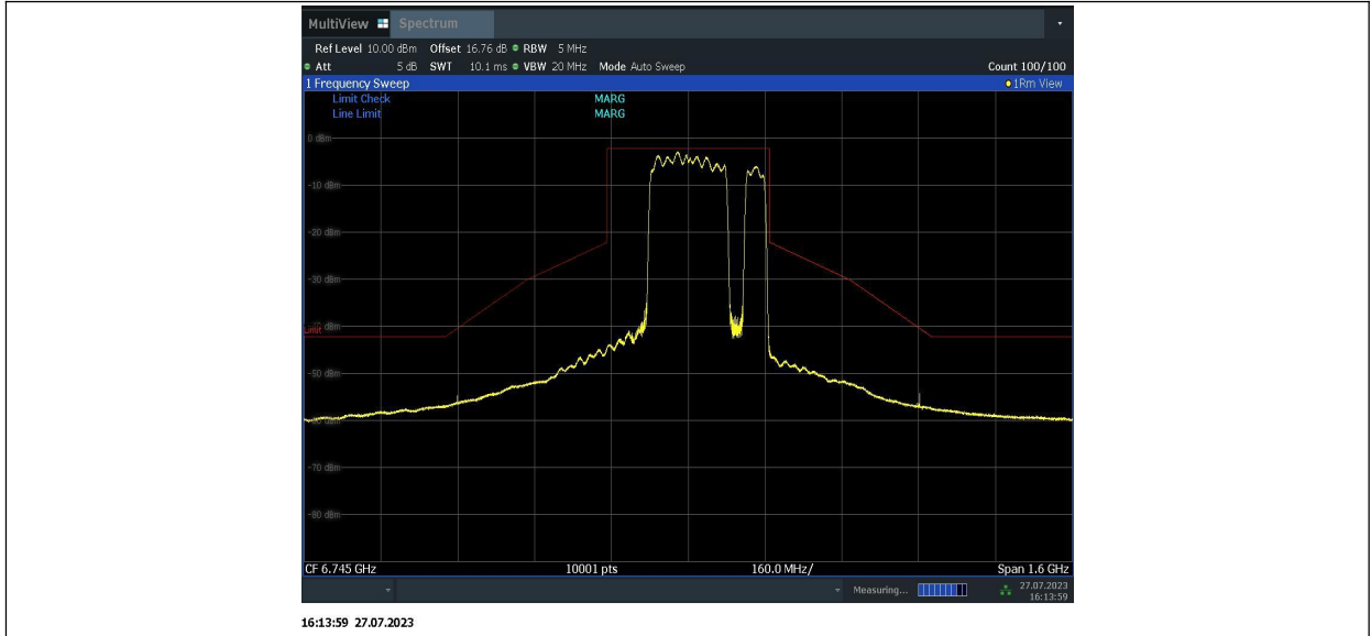
11BE320MIMO_Ant2_6745_996+996+484_12
