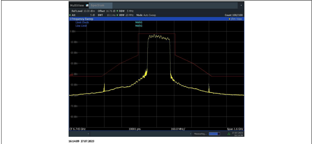
11BE320MIMO_Ant2_6745_996+996+996+484_1
