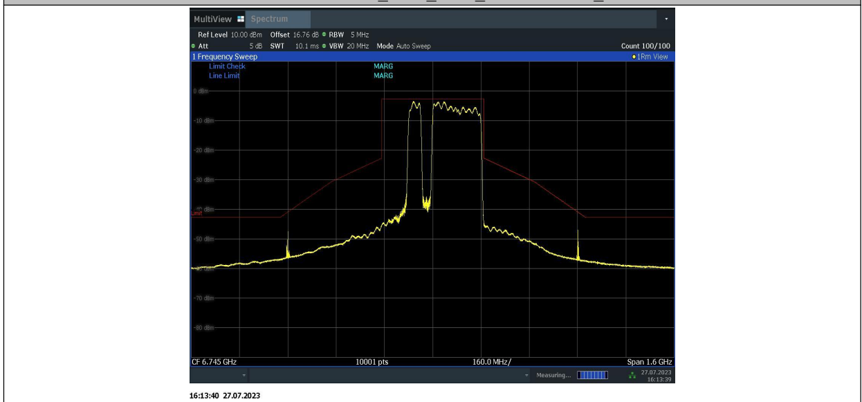
11BE320MIMO_Ant2_6745_996+996+484_8
