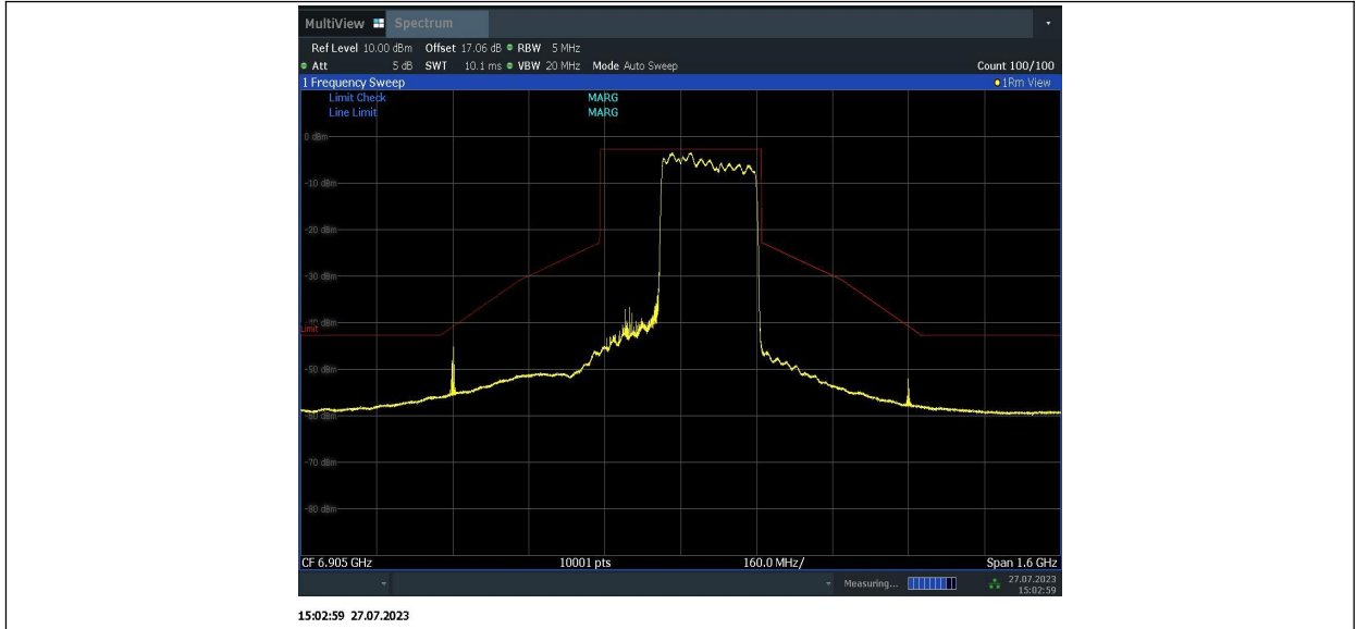
11BE320MIMO_Ant1_6905_996+996+484_8
