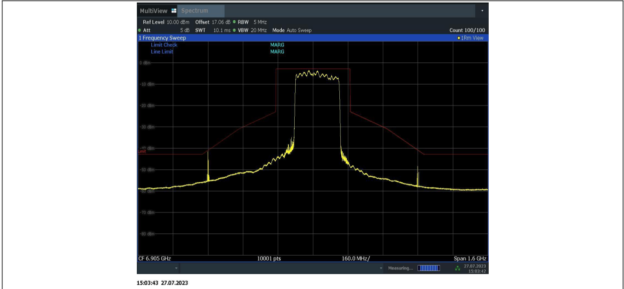
11BE320MIMO_Ant1_6905_996+996+996+484_1
