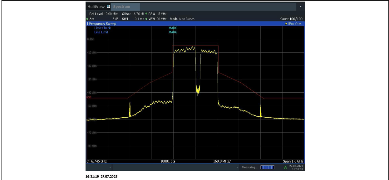
11BE320MIMO_Ant2_6745_996+996+996+484_6
