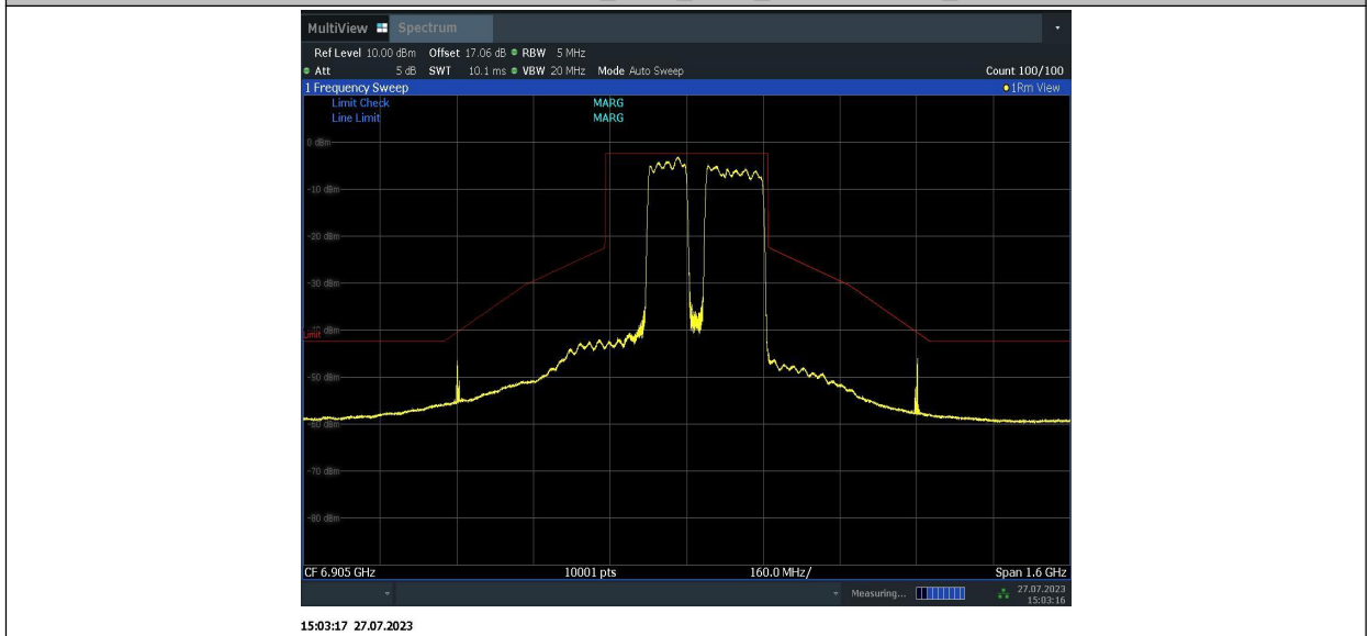
11BE320MIMO_Ant1_6905_996+996+484_9
