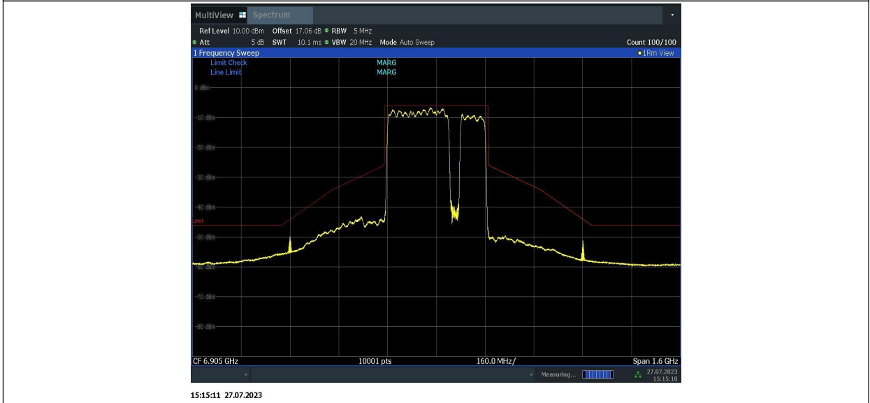
11BE320MIMO_Ant1_6905_996+996+996+484_7
