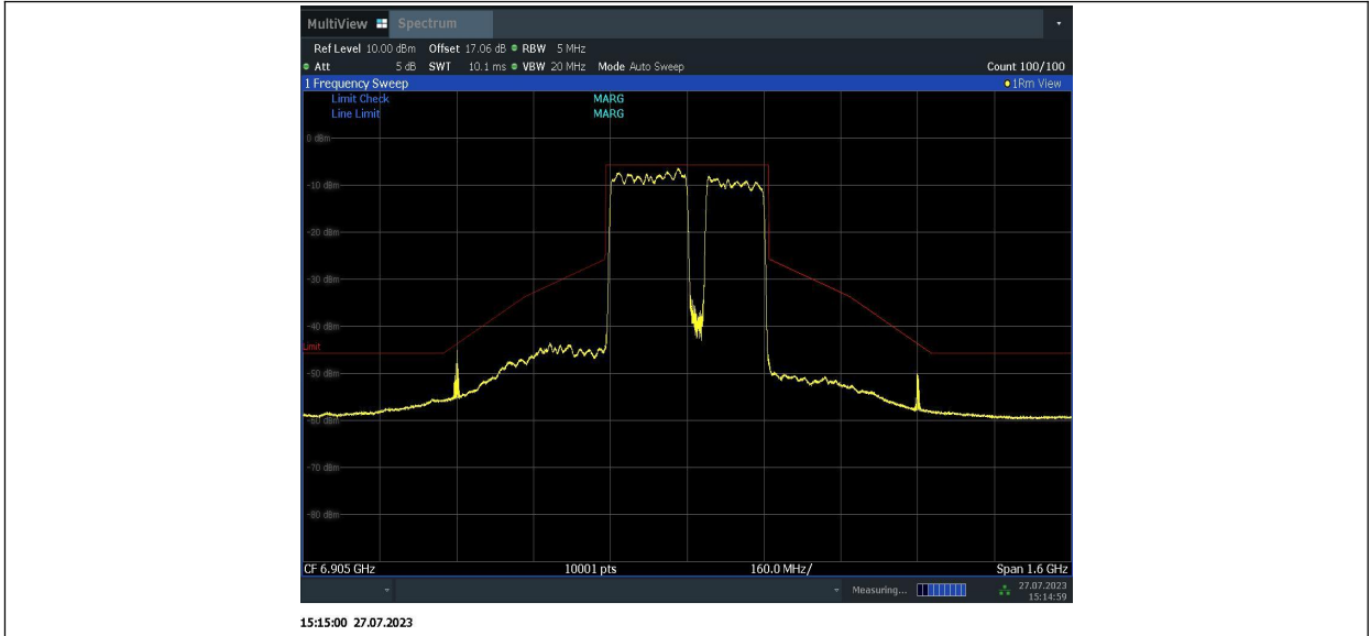
11BE320MIMO_Ant1_6905_996+996+996+484_6
