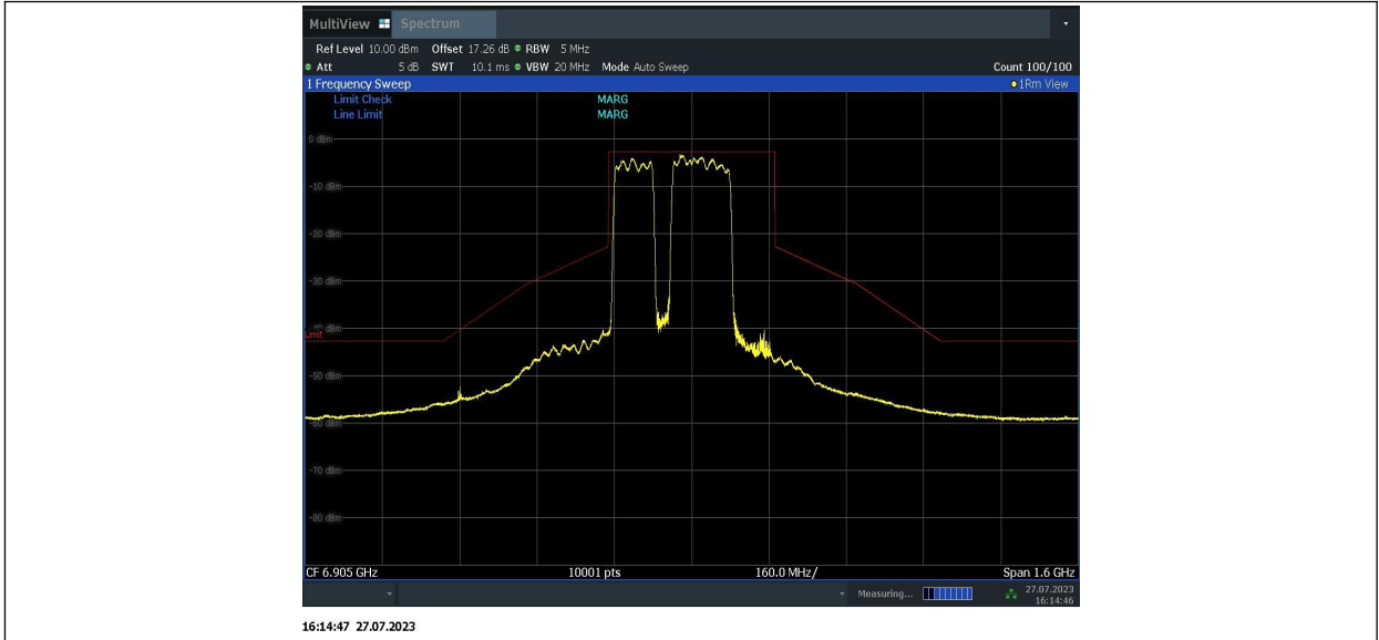
11BE320MIMO_Ant2_6905_996+996+484_4
