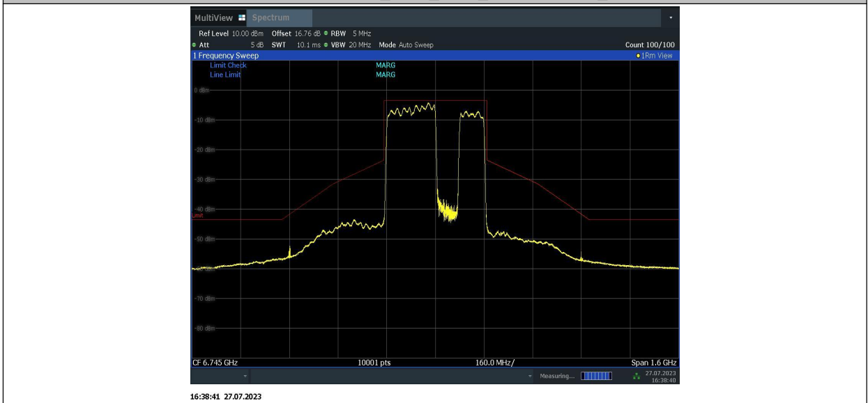
11BE320MIMO_Ant2_6745_996+996+996_3
