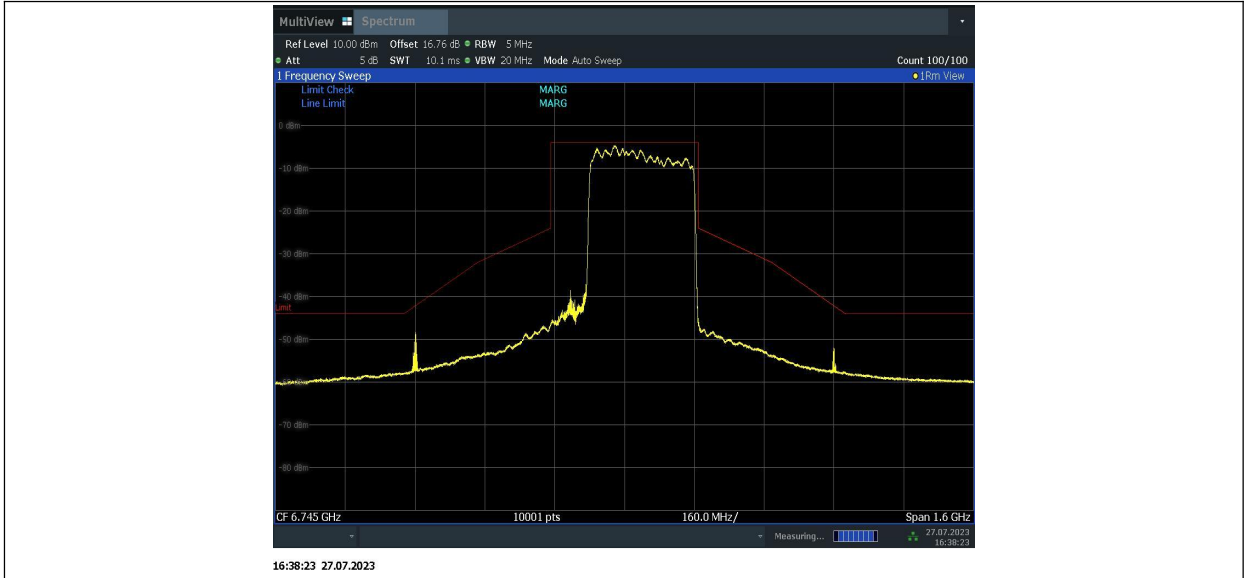
11BE320MIMO_Ant2_6745_996+996+996_2
