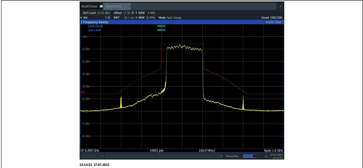
11BE320MIMO_Ant1_6905_996+996+996+484_2
