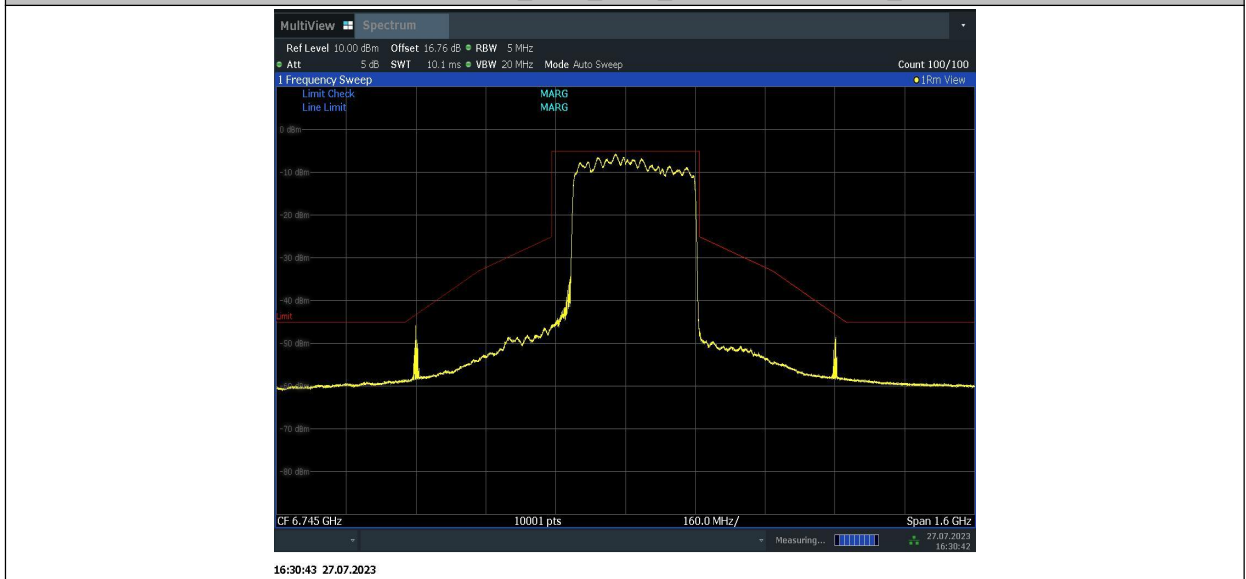
11BE320MIMO_Ant2_6745_996+996+996+484_1
