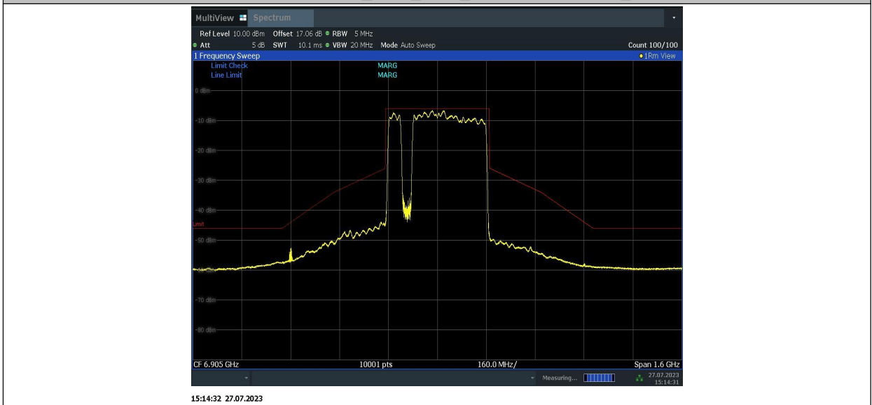
11BE320MIMO_Ant1_6905_996+996+996+484_2
