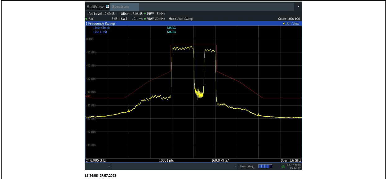
11BE320MIMO_Ant1_6905_996+996+996_4
