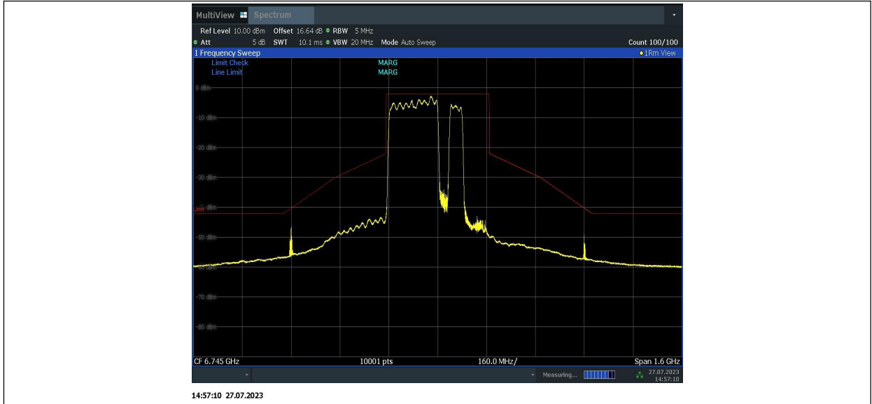
11BE320MIMO_Ant1_6745_996+996+484_6
