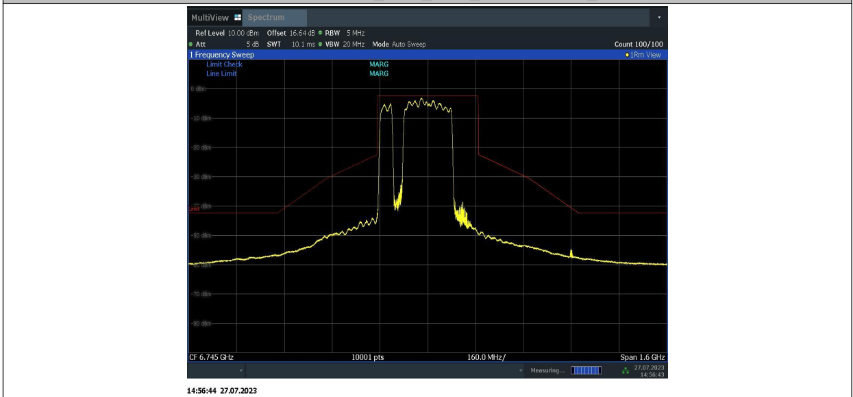
11BE320MIMO_Ant1_6745_996+996+484_2
