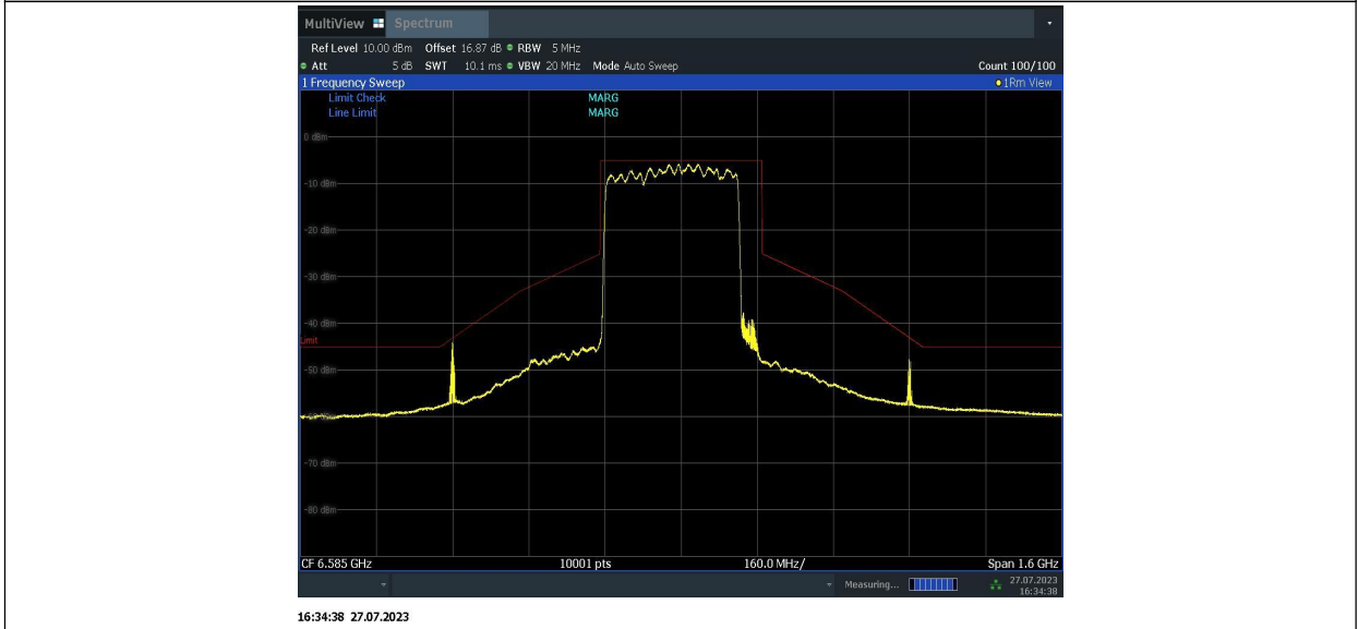
11BE320MIMO_Ant2_6585_996+996+996_1
