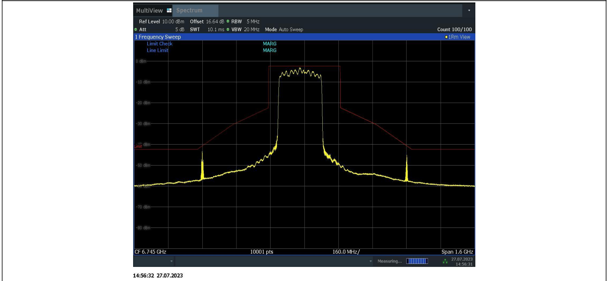
11BE320MIMO_Ant1_6745_996+996+484_2
