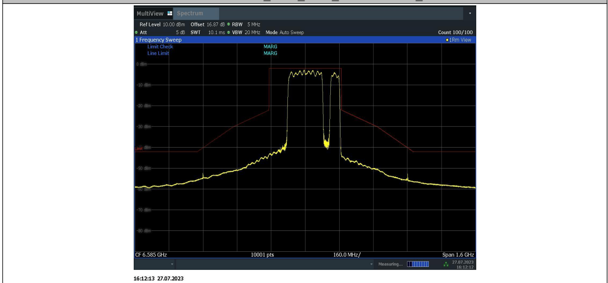
11BE320MIMO_Ant2_6585_996+996+484_11
