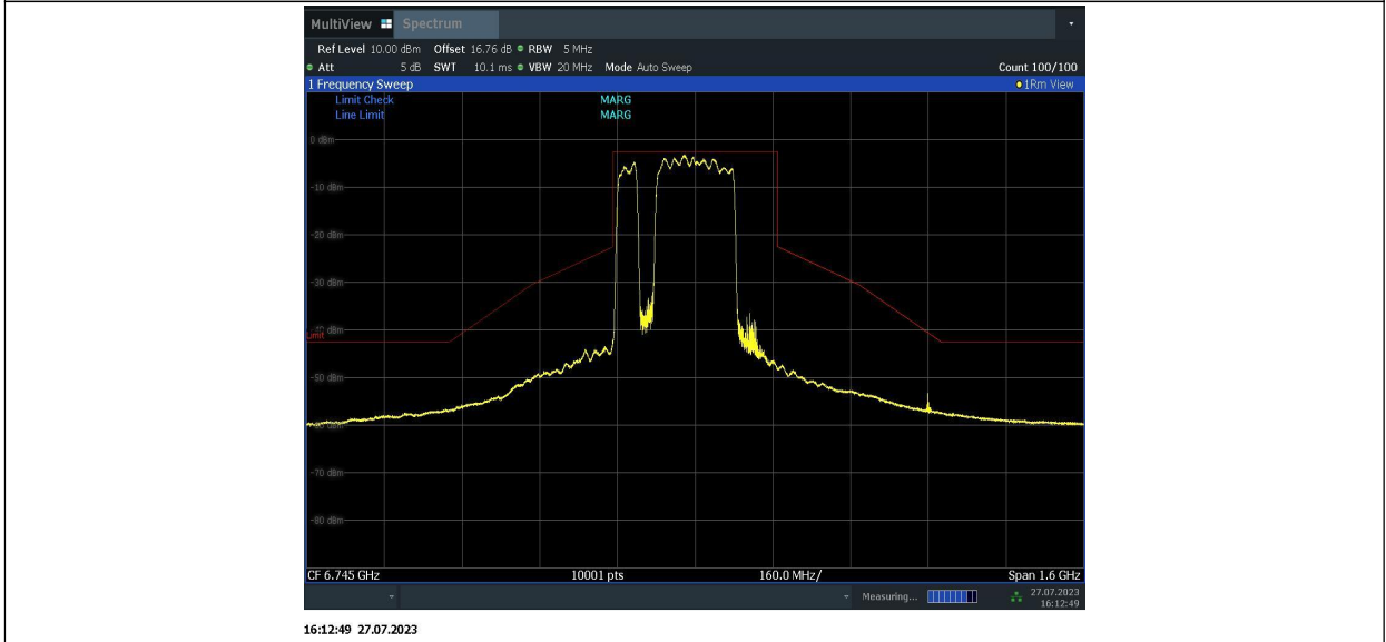
11BE320MIMO_Ant2_6745_996+996+484_3
