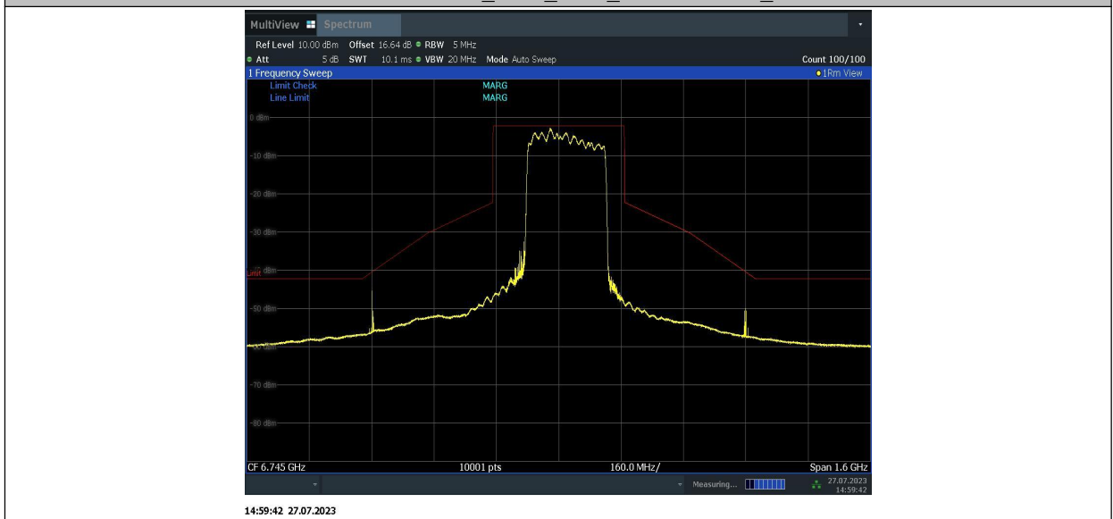
11BE320MIMO_Ant1_6745_996+996+484_12
