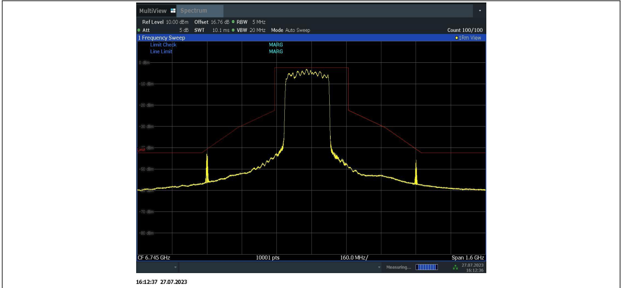
11BE320MIMO_Ant2_6745_996+996+484_2
