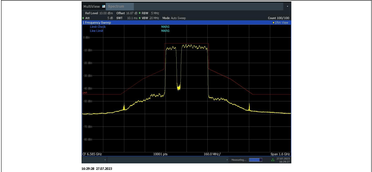
11BE320MIMO_Ant2_6585_996+996+996+484_4
