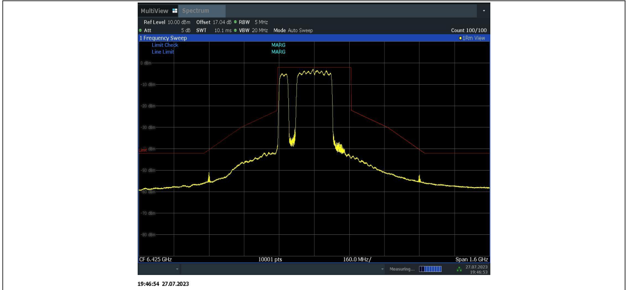
11BE320MIMO_Ant2_6425_996+996+484_3
