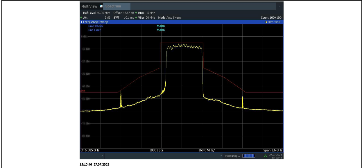
11BE320MIMO_Ant1_6585_996+996+996+484_2
