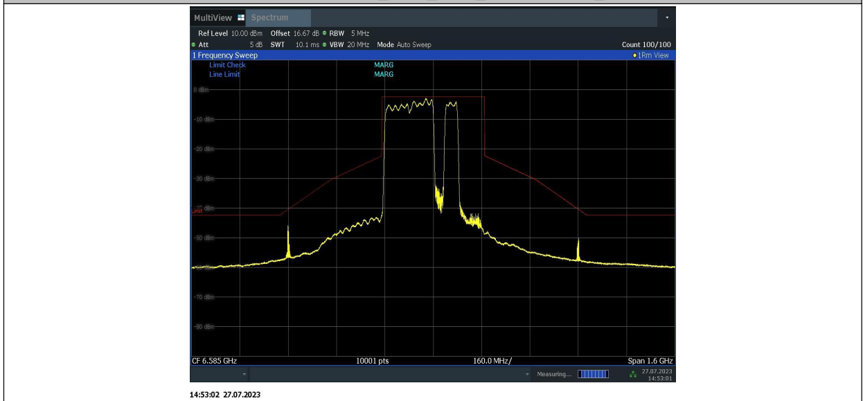
11BE320MIMO_Ant1_6585_996+996+484_5
