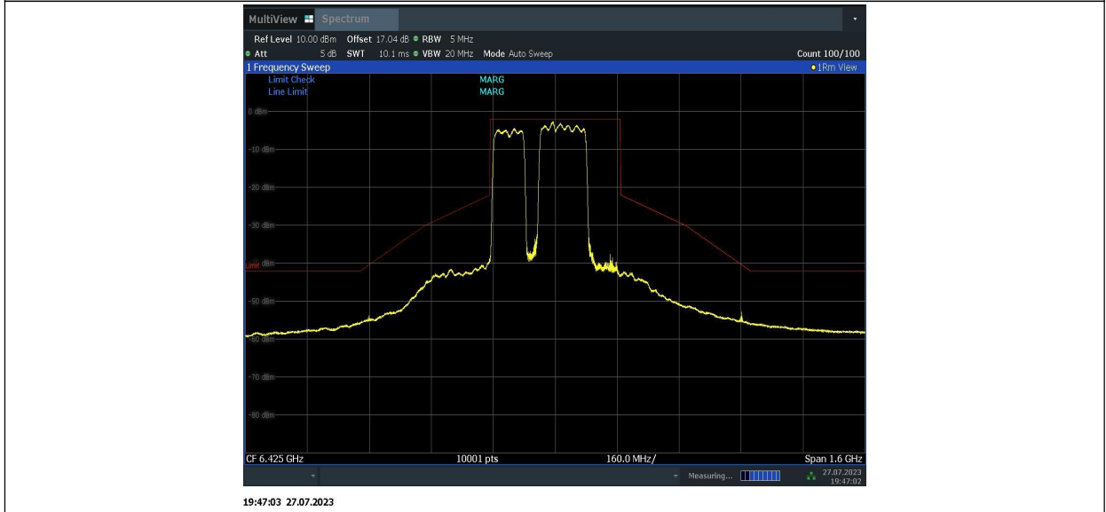
11BE320MIMO_Ant2_6425_996+996+484_4
