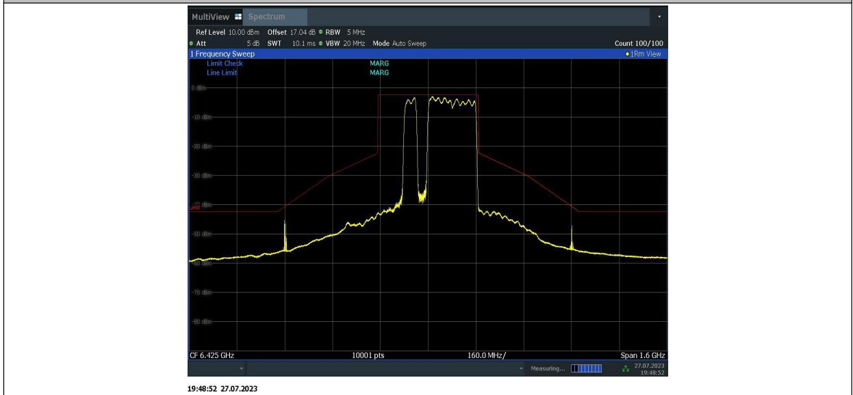
11BE320MIMO_Ant2_6425_996+996+484_9
