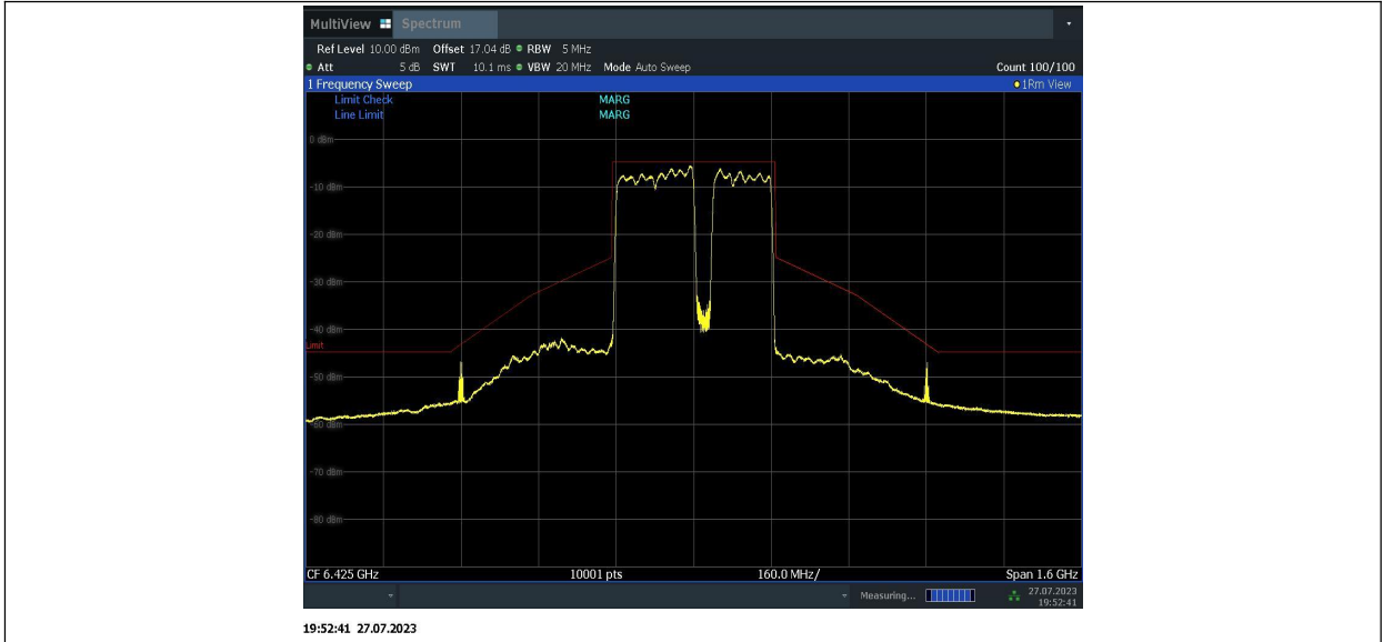
11BE320MIMO_Ant2_6425_996+996+996+484_6
