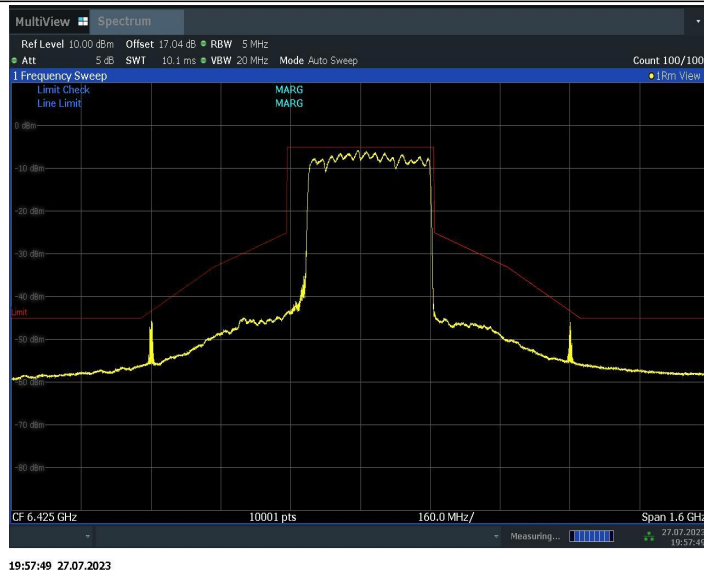
11BE320MIMO_Ant2_6425_996+996+996+484_2
