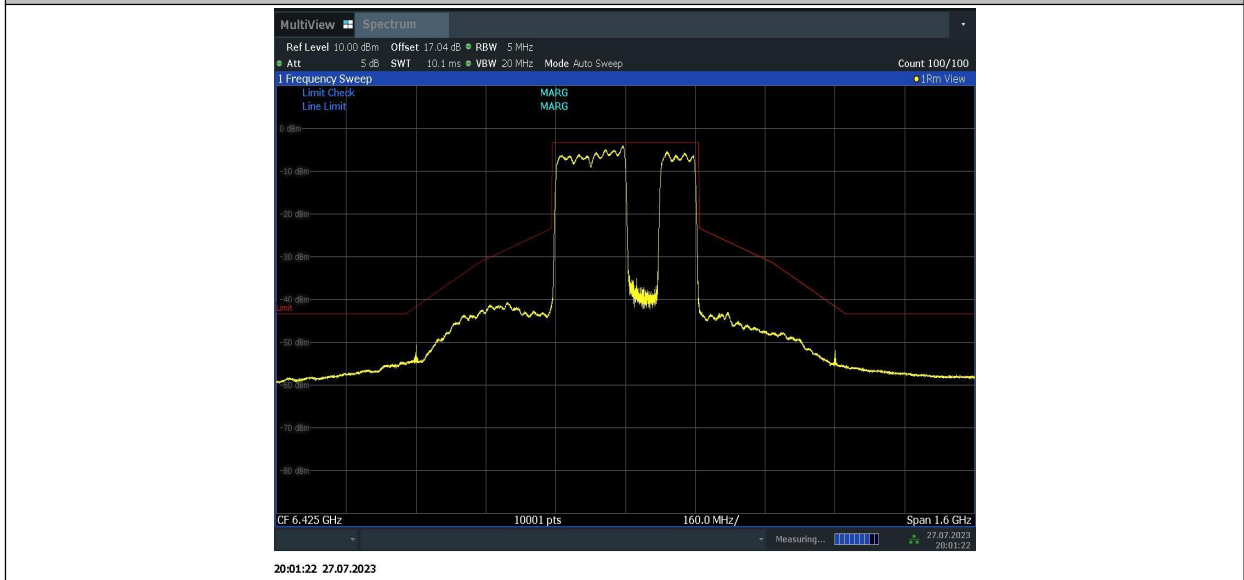
11BE320MIMO_Ant2_6425_996+996+996_4
