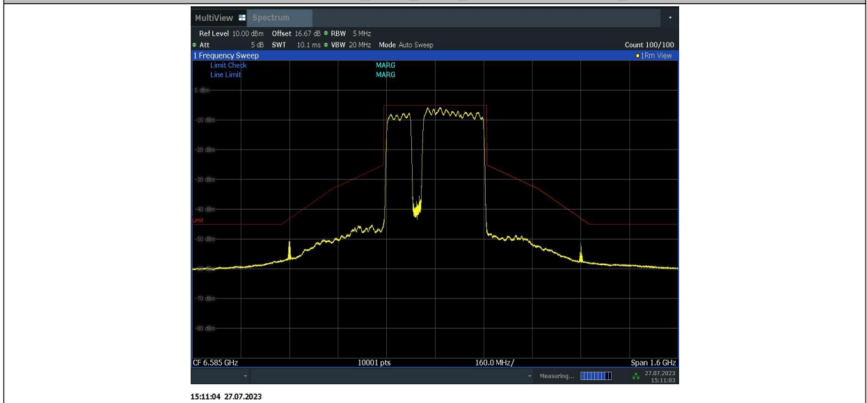
11BE320MIMO_Ant1_6585_996+996+996+484_3
