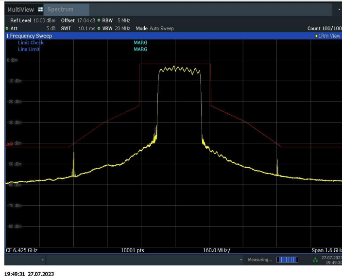
11BE320MIMO_Ant2_6425_996+996+996+484_1
