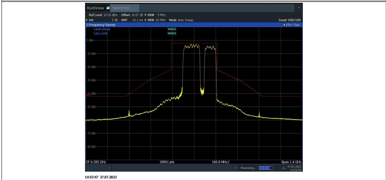
11BE320MIMO_Ant1_6585_996+996+484_10
