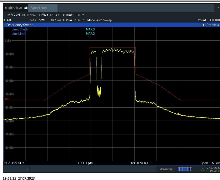
11BE320MIMO_Ant2_6425_996+996+996+484_2
