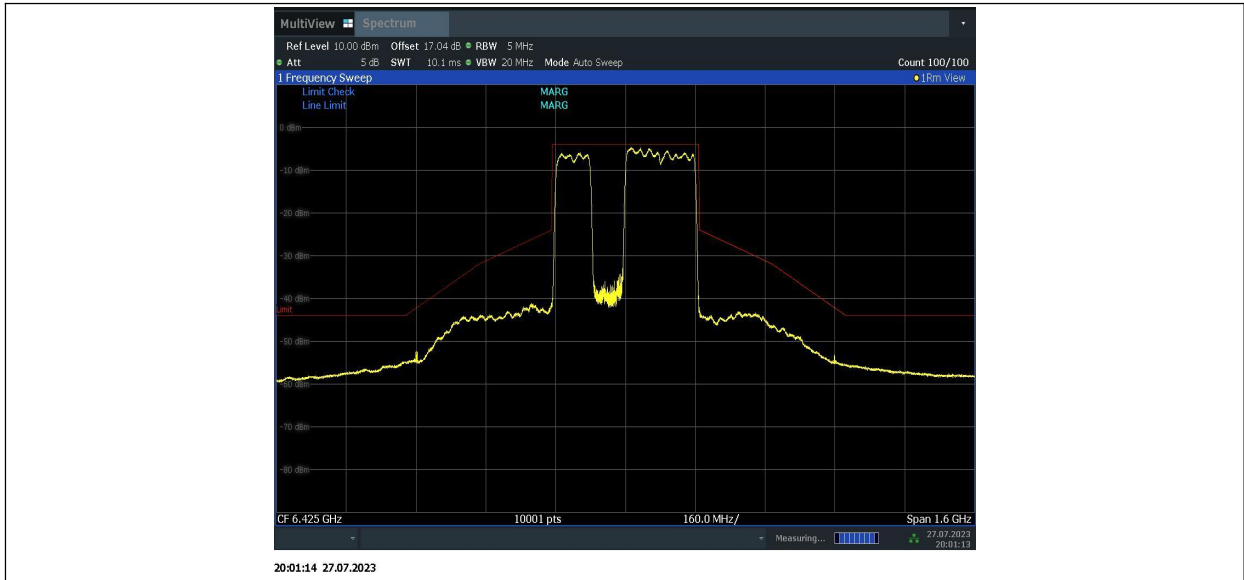
11BE320MIMO_Ant2_6425_996+996+996_3
