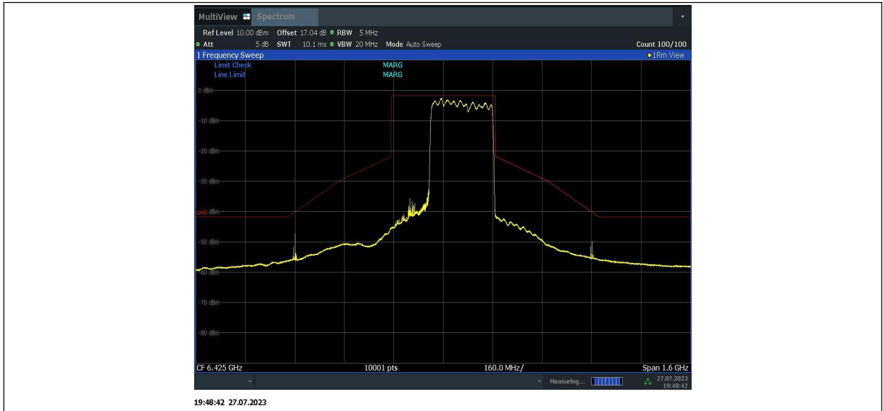
11BE320MIMO_Ant2_6425_996+996+484_8
