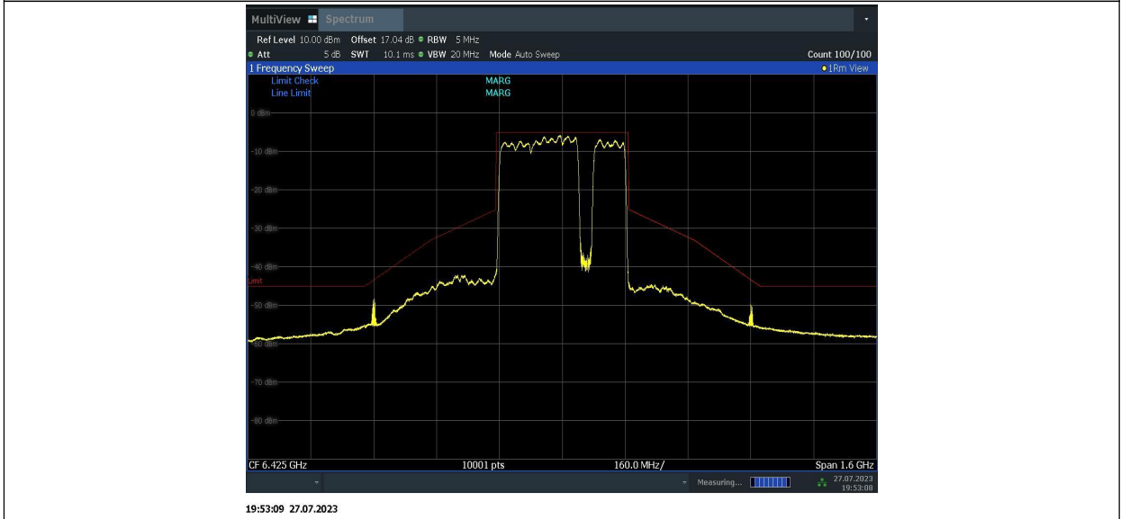
11BE320MIMO_Ant2_6425_996+996+996+484_7
