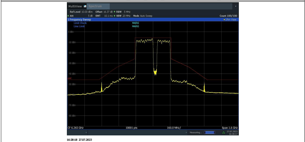
11BE320MIMO_Ant2_6265_996+996+996+484_5
