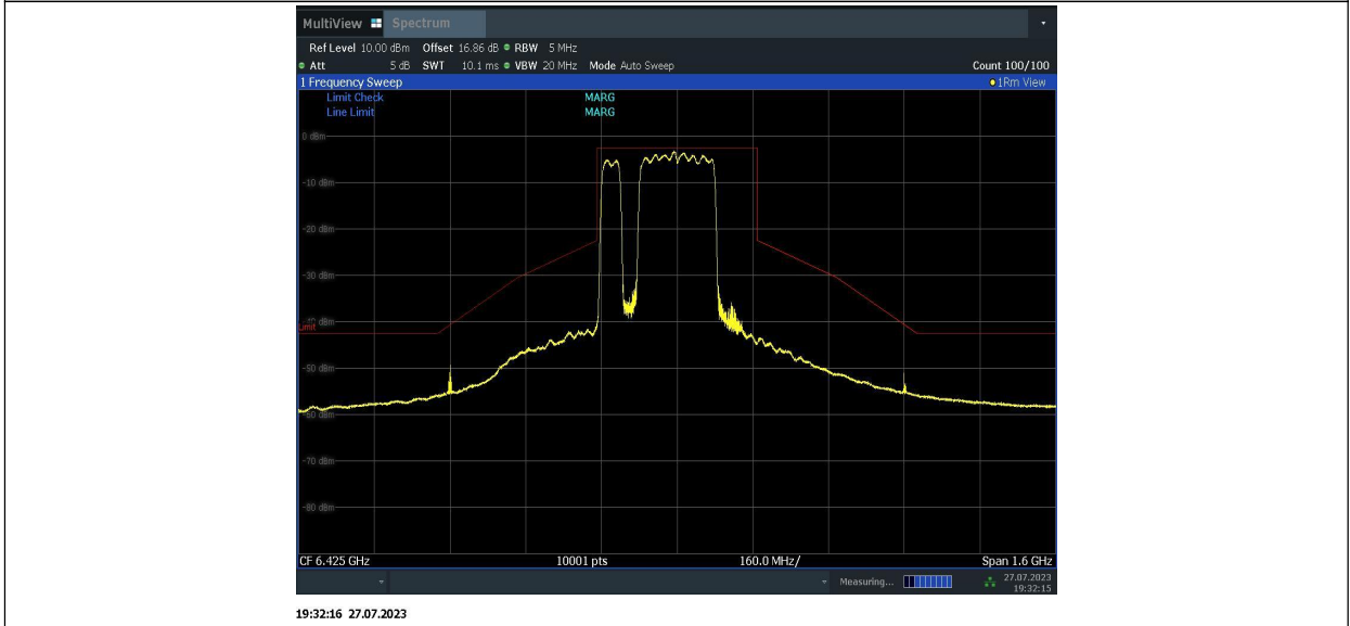
11BE320MIMO_Ant1_6425_996+996+484_3
