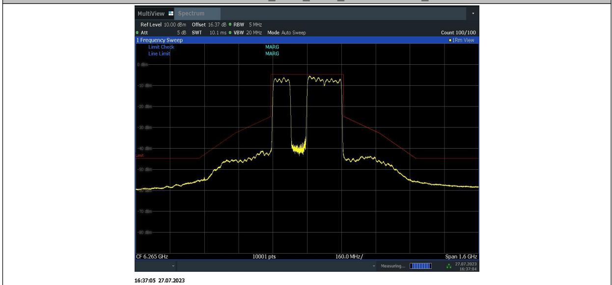
11BE320MIMO_Ant2_6265_996+996+996_2
