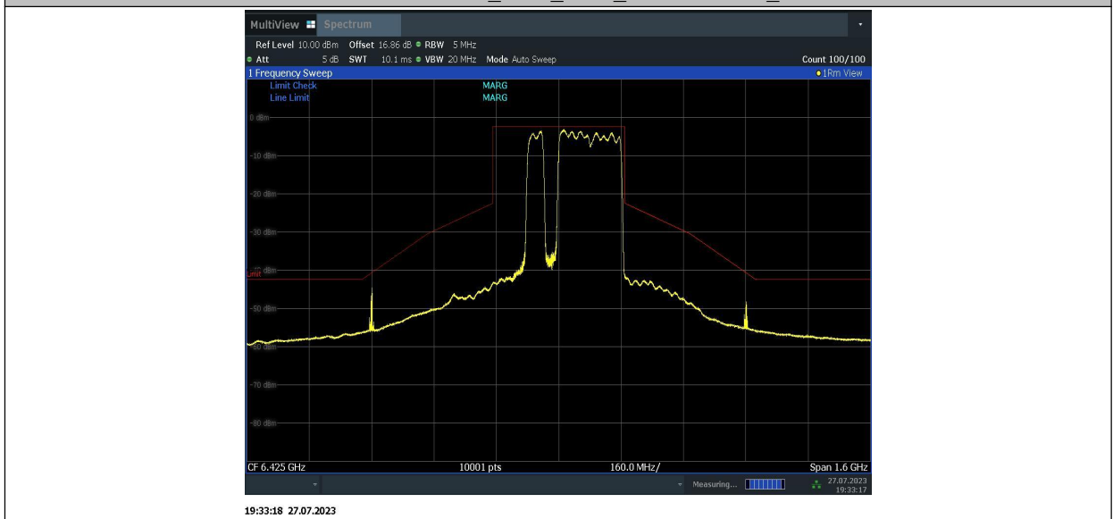
11BE320MIMO_Ant1_6425_996+996+484_8
