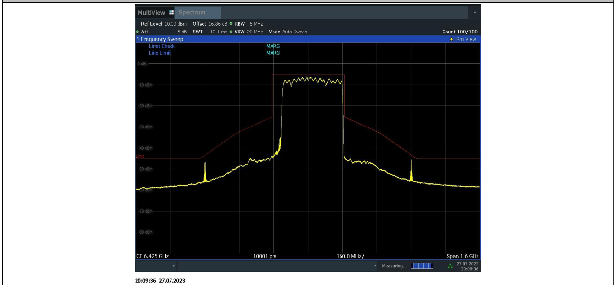
11BE320MIMO_Ant1_6425_996+996+484_1
