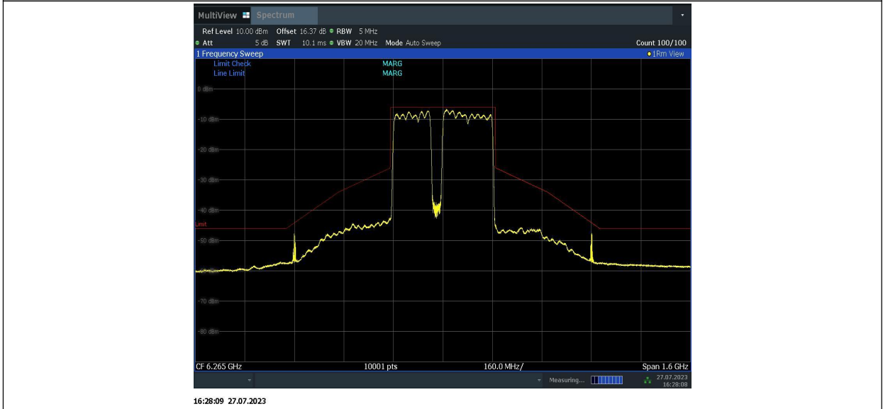
11BE320MIMO_Ant2_6265_996+996+996+484_5
