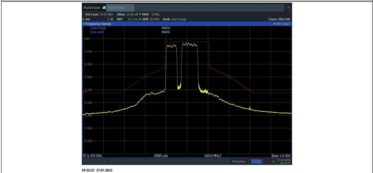
11BE320MIMO_Ant1_6425_996+996+484_3
