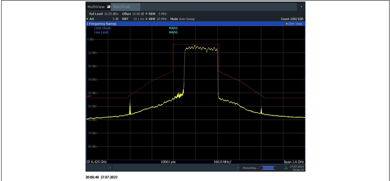
11BE320MIMO_Ant1_6425_996+996+996_2
