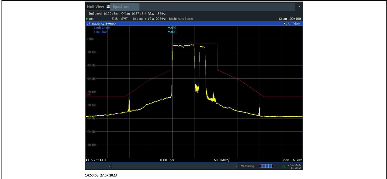
11BE320MIMO_Ant2_6265_996+996+484_6
