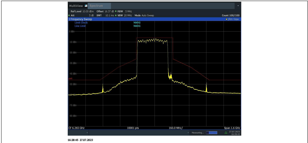
11BE320MIMO_Ant2_6265_996+996+996_1
