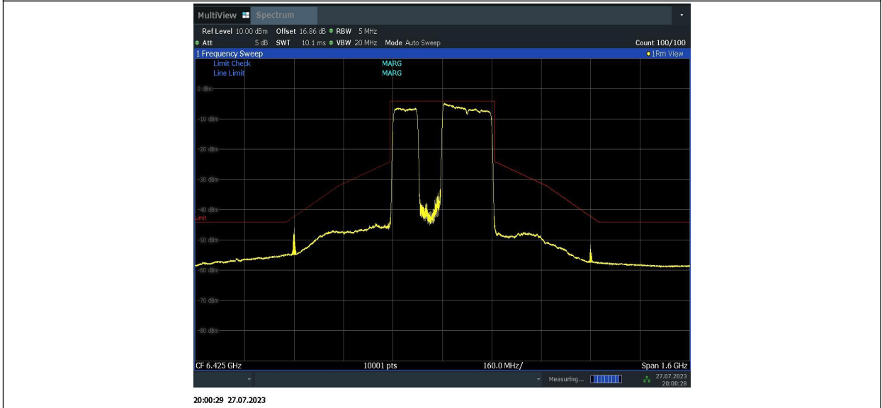
11BE320MIMO_Ant1_6425_996+996+996_3
