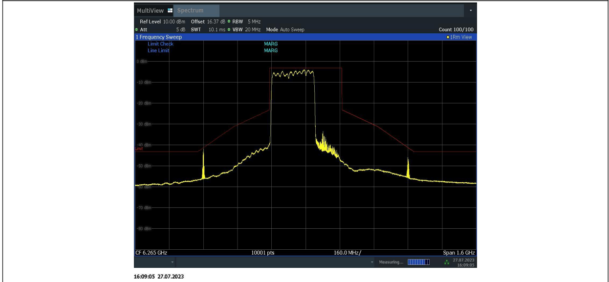
11BE320MIMO_Ant2_6265_996+996+484_7
