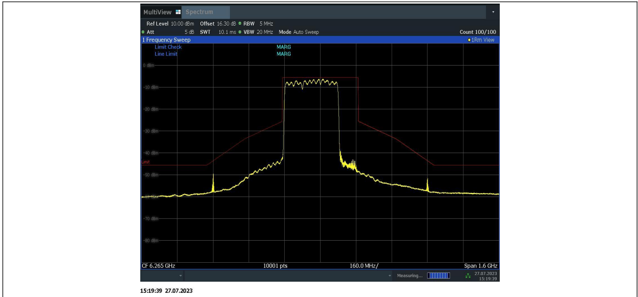
11BE320MIMO_Ant2_6265_996+996+484_1
