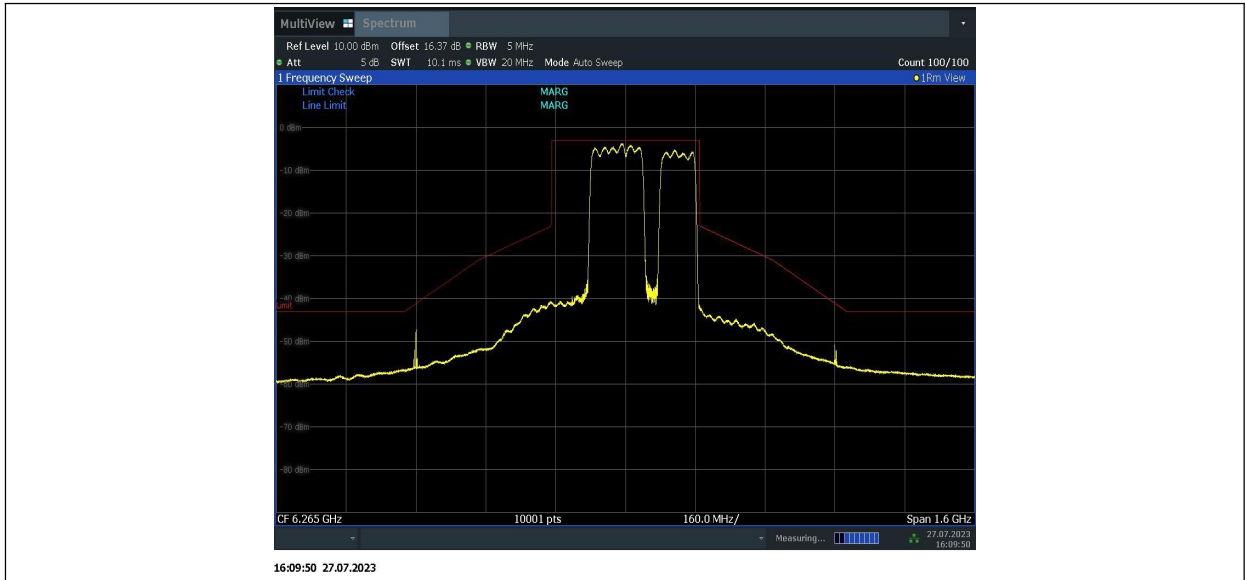
11BE320MIMO_Ant2_6265_996+996+484_11
