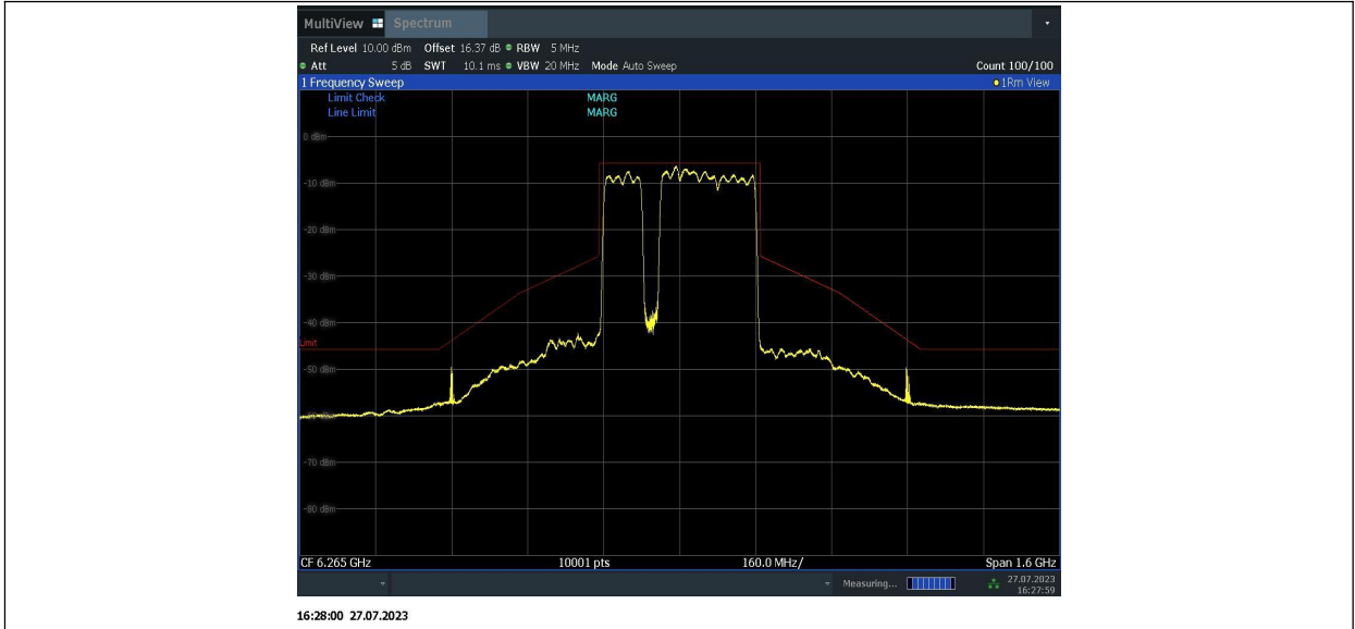
11BE320MIMO_Ant2_6265_996+996+996+484_4
