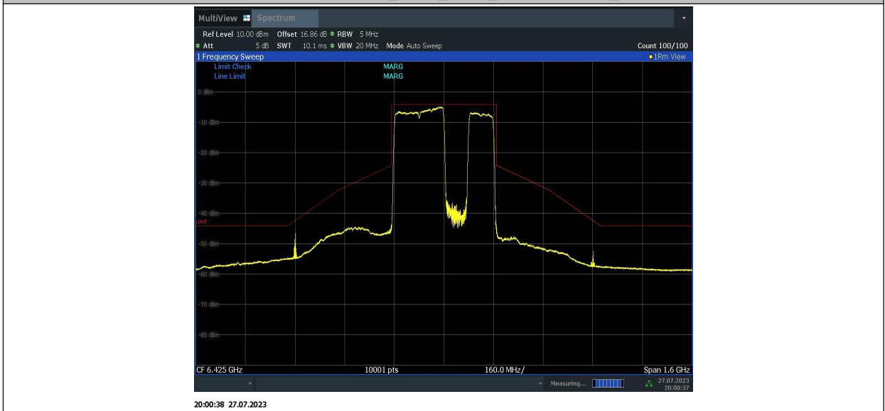
11BE320MIMO_Ant1_6425_996+996+996_3
