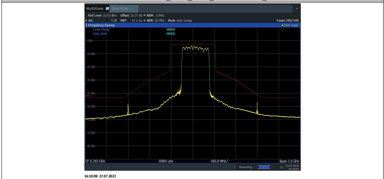
11BE320MIMO_Ant2_6265_996+996+484_12
