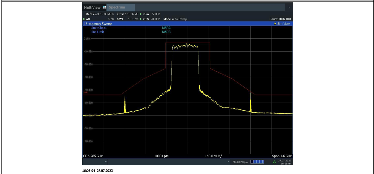
11BE320MIMO_Ant2_6265_996+996+484_2
