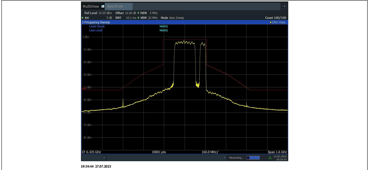
11BE320MIMO_Ant1_6425_996+996+484_12
