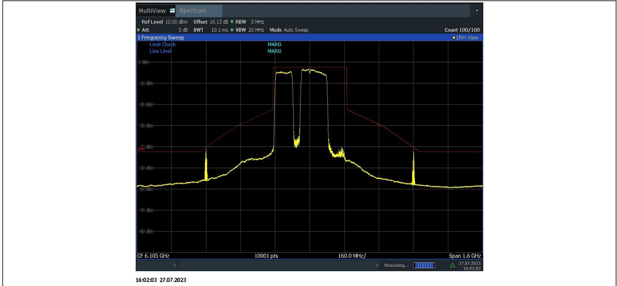
11BE320MIMO_Ant2_6105_996+996+484_4
