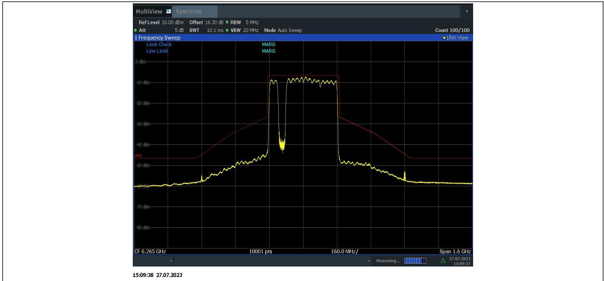
11BE320MIMO_Ant1_6265_996+996+996+484_3
