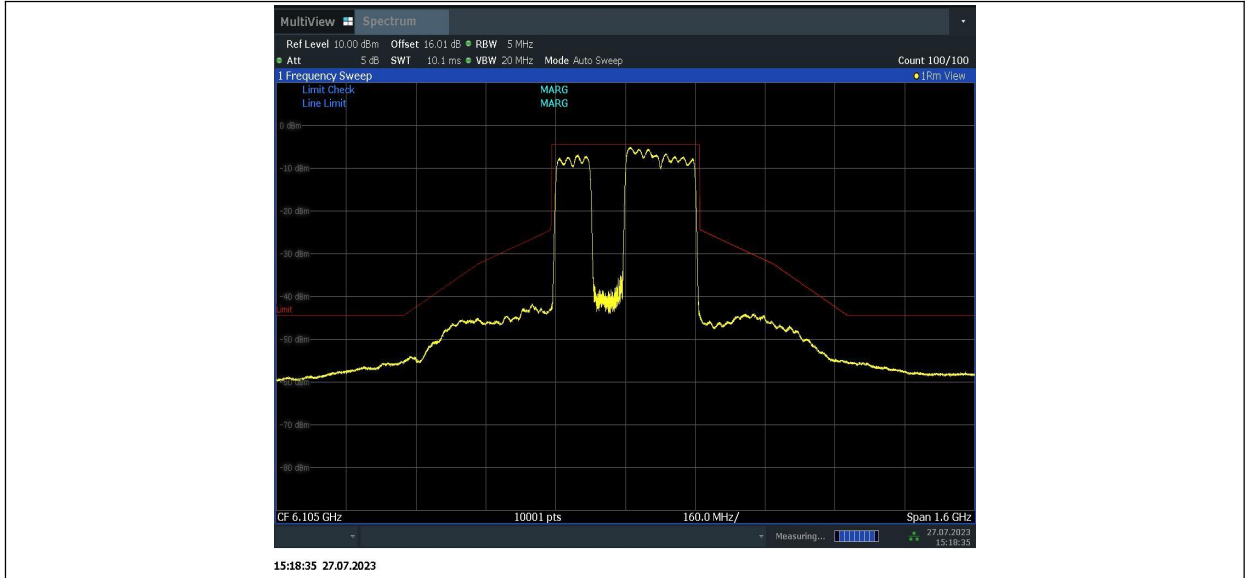
11BE320MIMO_Ant1_6105_996+996+996_3
