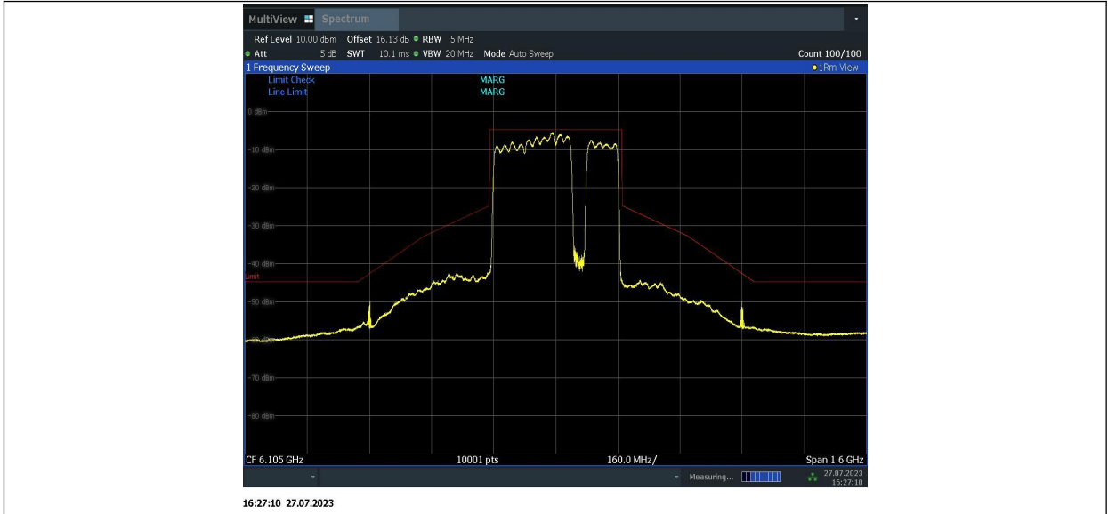
11BE320MIMO_Ant2_6105_996+996+996+484_7
