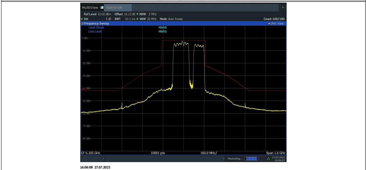
11BE320MIMO_Ant2_6105_996+996+484_10
