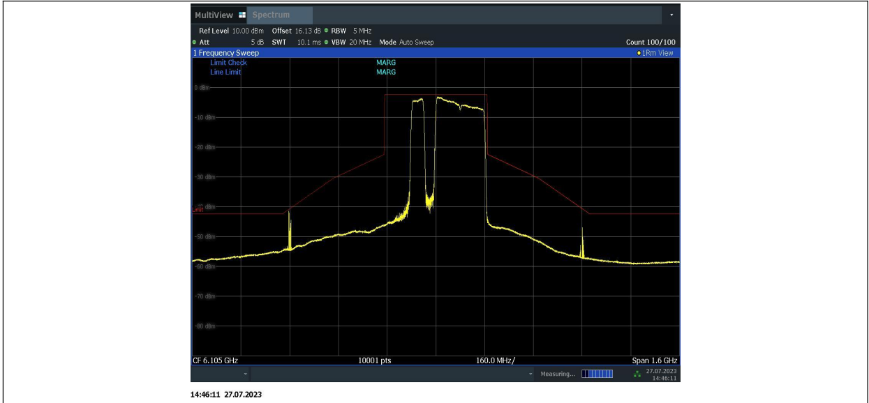
11BE320MIMO_Ant2_6105_996+996+484_9
