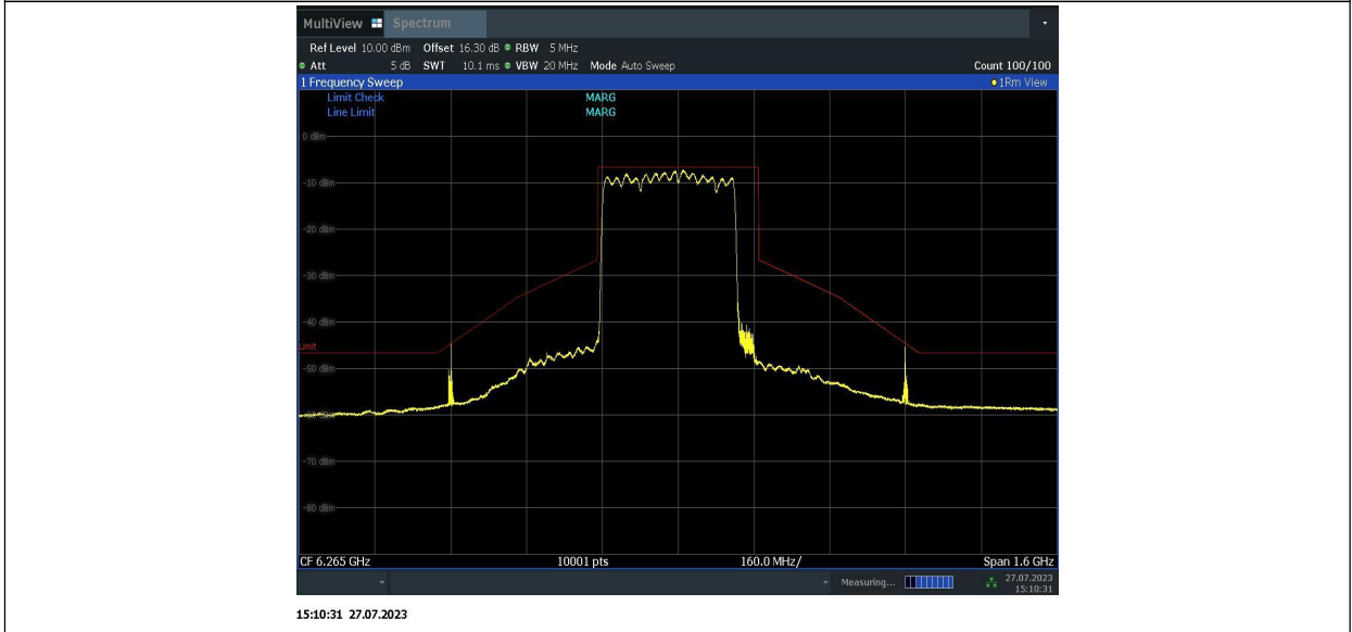
11BE320MIMO_Ant1_6265_996+996+996_1
