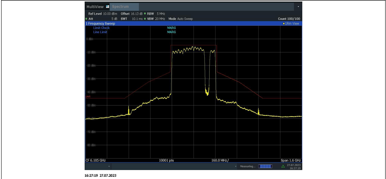
11BE320MIMO_Ant2_6105_996+996+996+484_8
