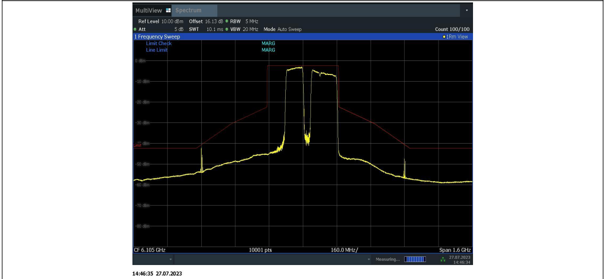
11BE320MIMO_Ant2_6105_996+996+484_10
