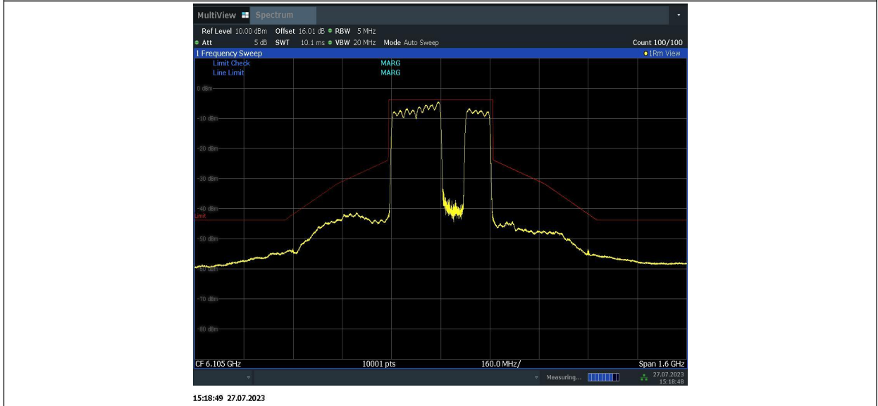
11BE320MIMO_Ant1_6105_996+996+996_4
