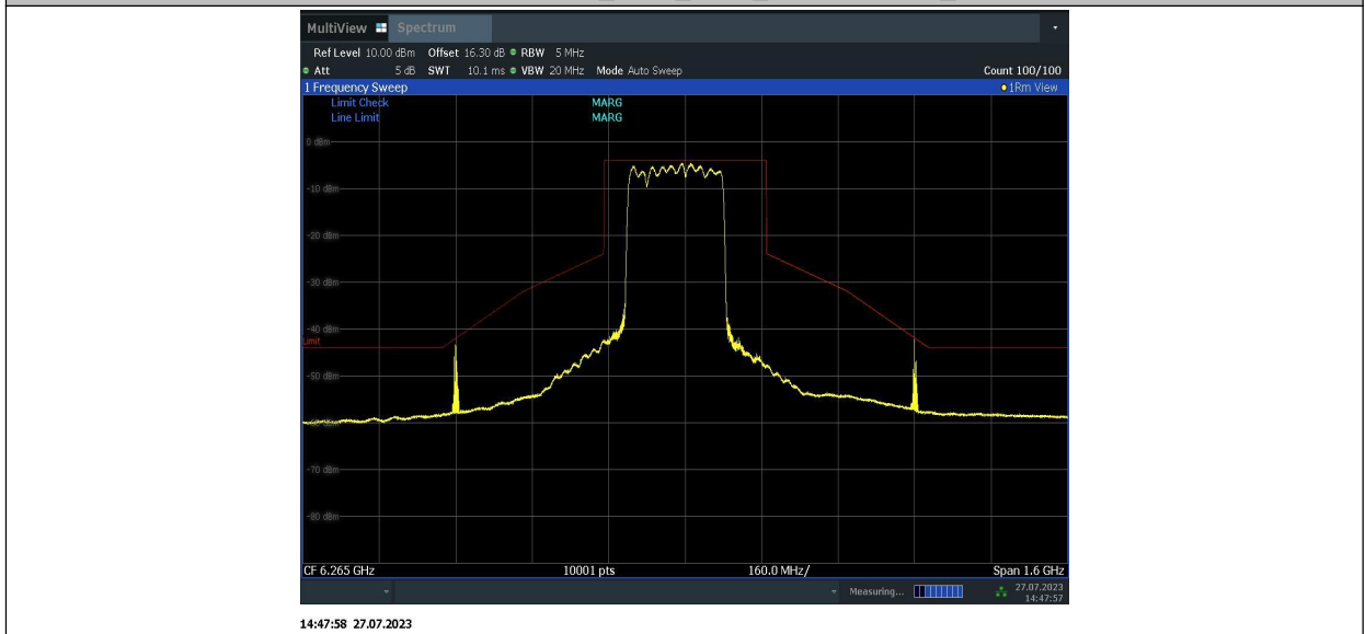
11BE320MIMO_Ant1_6265_996+996+484_1
