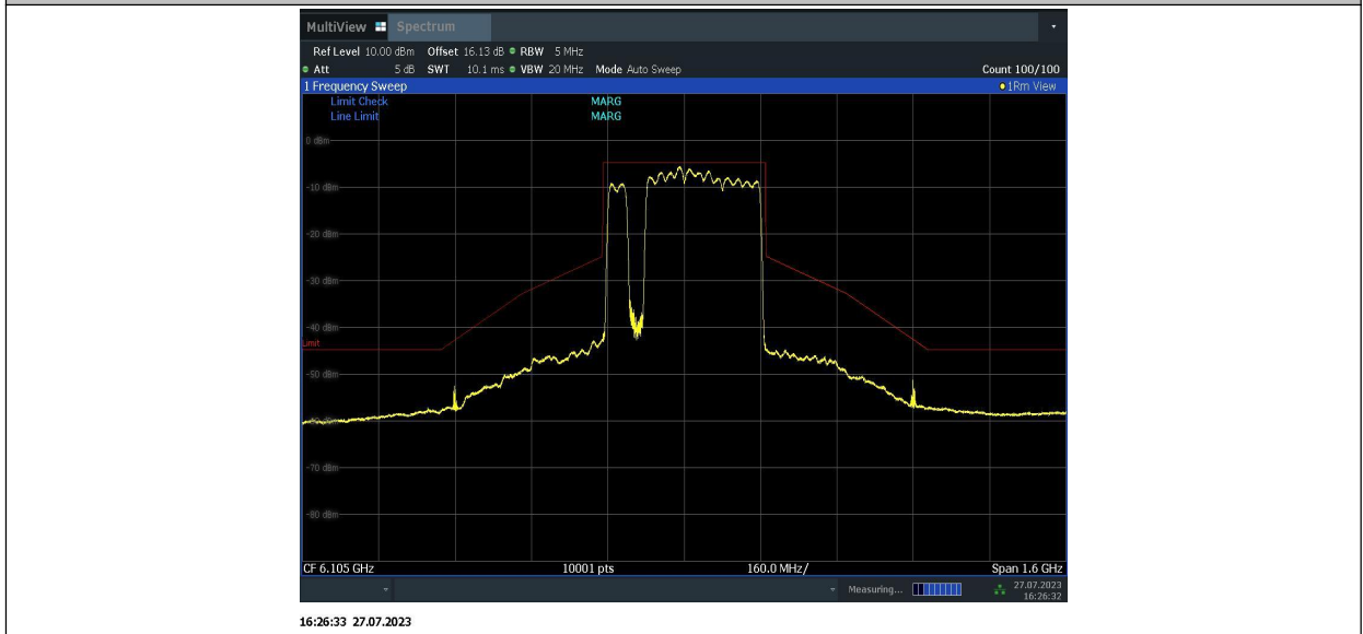
11BE320MIMO_Ant2_6105_996+996+996+484_3
