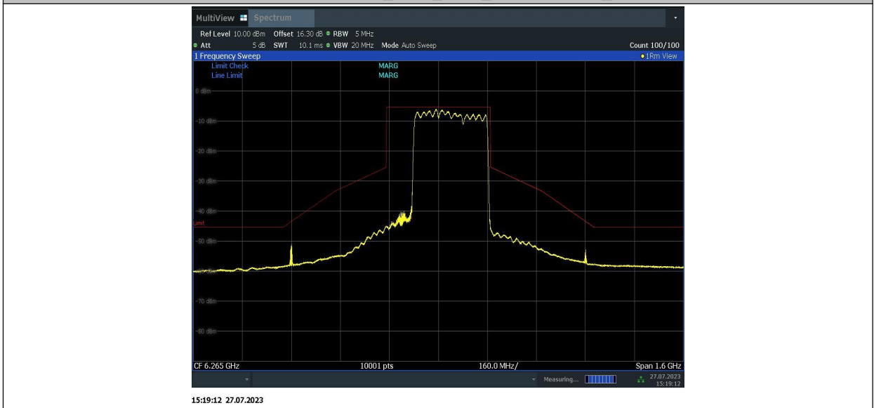
11BE320MIMO_Ant1_6265_996+996+996_1
