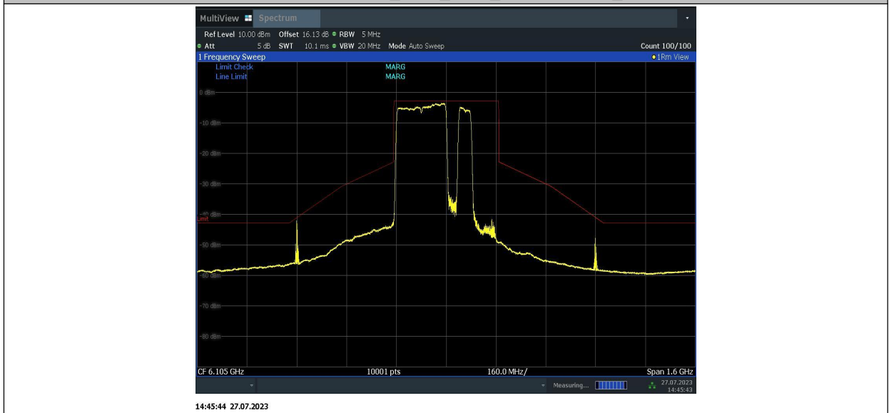
11BE320MIMO_Ant2_6105_996+996+484_5
