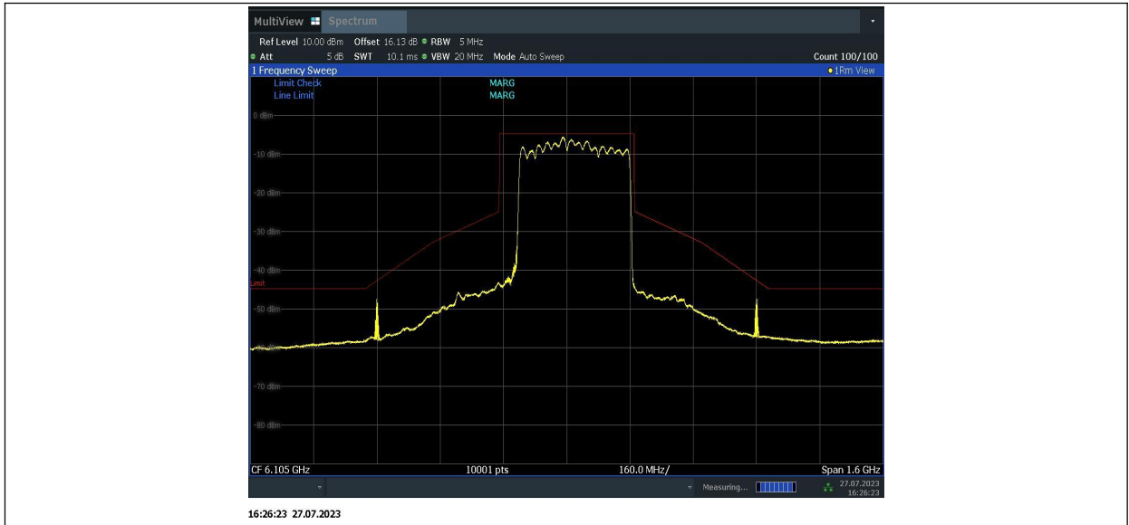
11BE320MIMO_Ant2_6105_996+996+996+484_2
