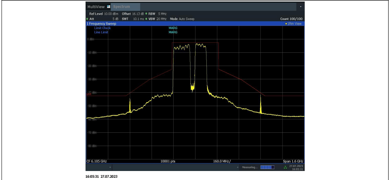
11BE320MIMO_Ant2_6105_996+996+484_5
