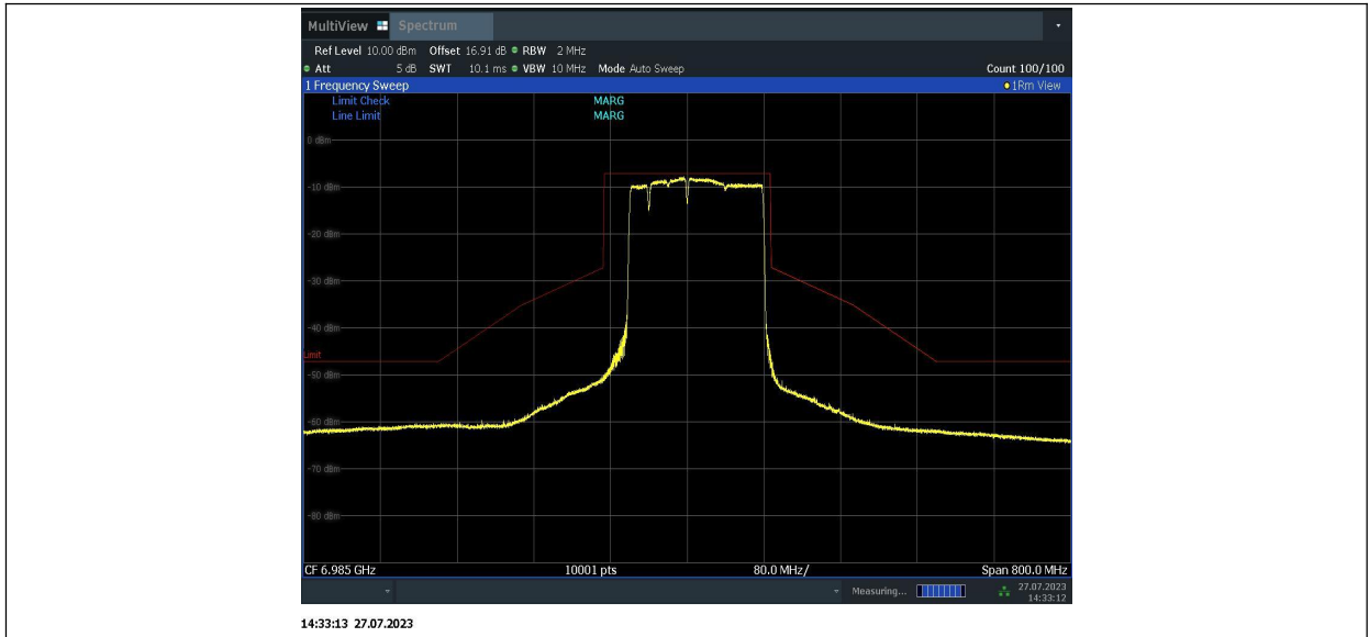
11BE160MIMO_Ant2_6985_996+484+242_2
