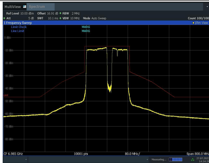
11BE160MIMO_Ant2_6985_996+484+242_5
