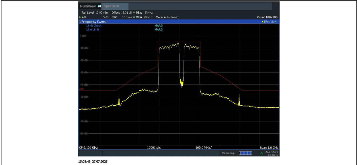
11BE320MIMO_Ant1_6105_996+996+996+484_6
