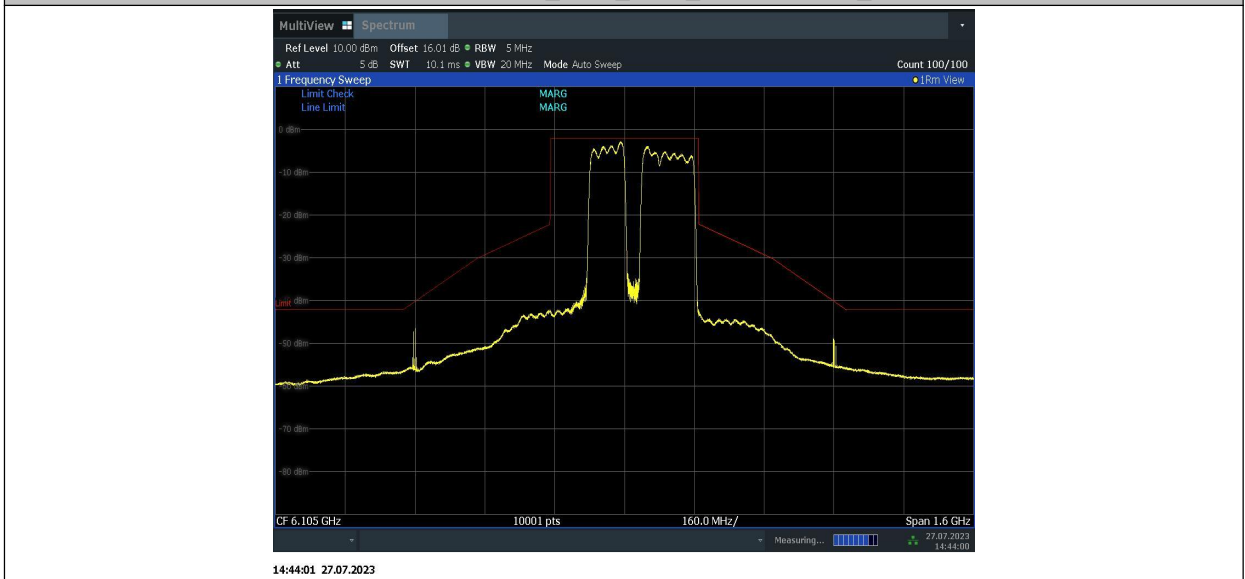
11BE320MIMO_Ant1_6105_996+996+484_9
