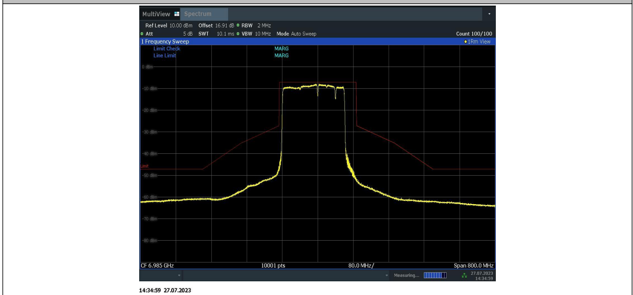
11BE160MIMO_Ant2_6985_996+484+242_8
