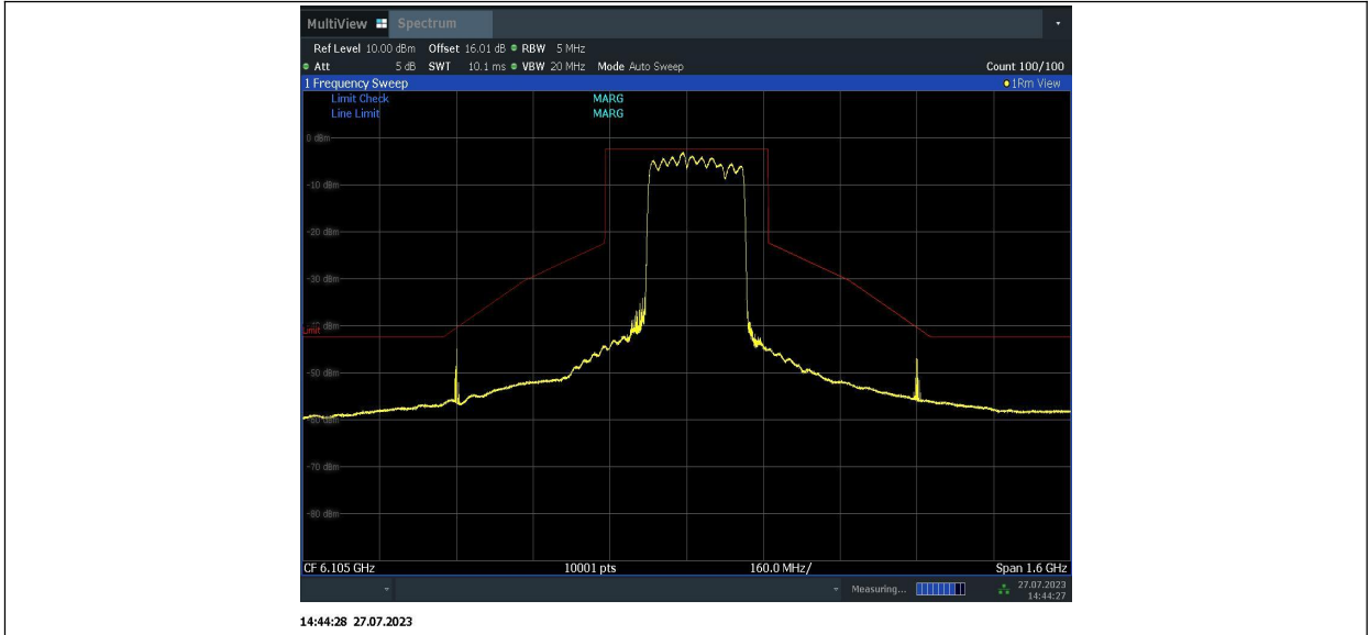
11BE320MIMO_Ant1_6105_996+996+996+484_1
