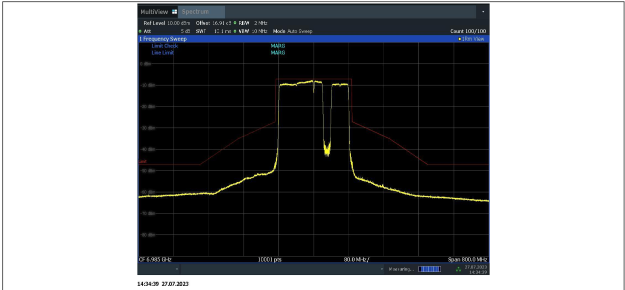
11BE160MIMO_Ant2_6985_996+484+242_7
