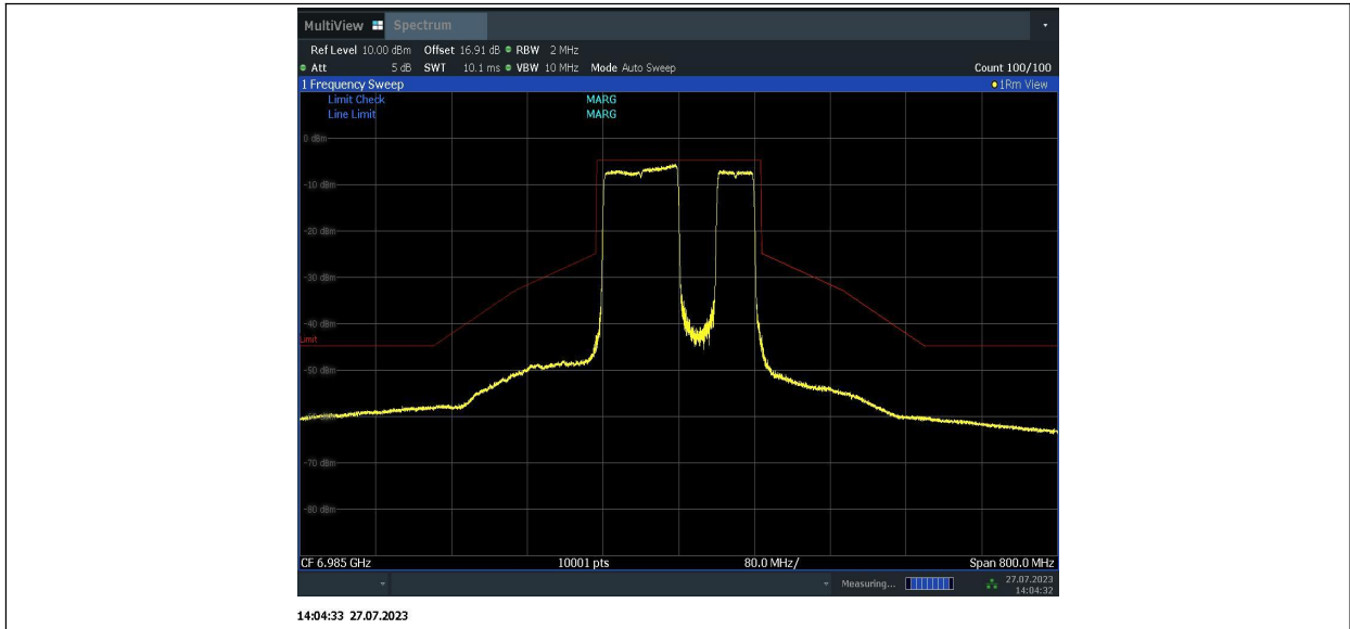
11BE160MIMO_Ant2_6985_996+484_4
