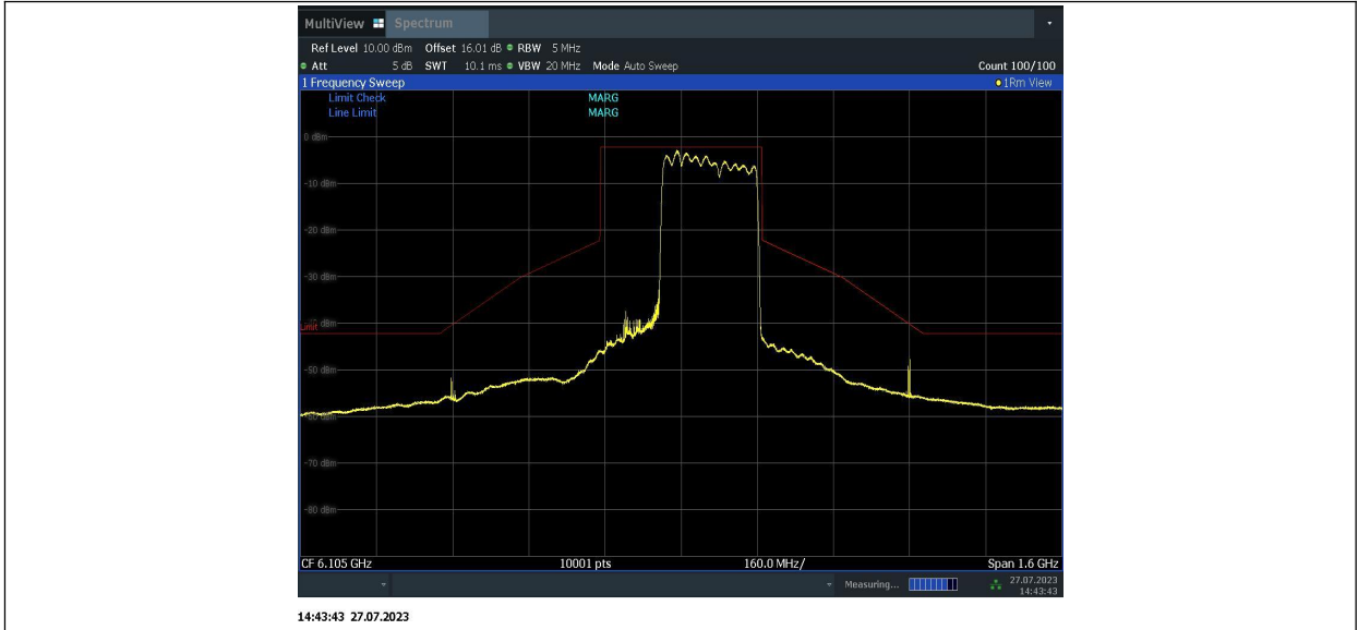
11BE320MIMO_Ant1_6105_996+996+484_8
