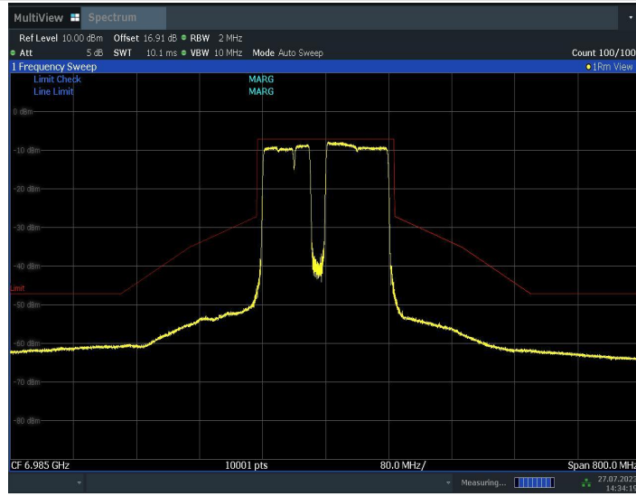
11BE160MIMO_Ant2_6985_996+484+242_4
