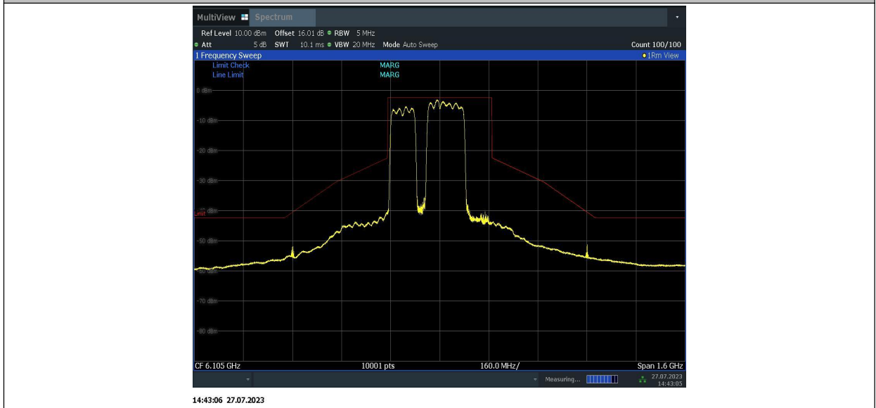
11BE320MIMO_Ant1_6105_996+996+484_4
