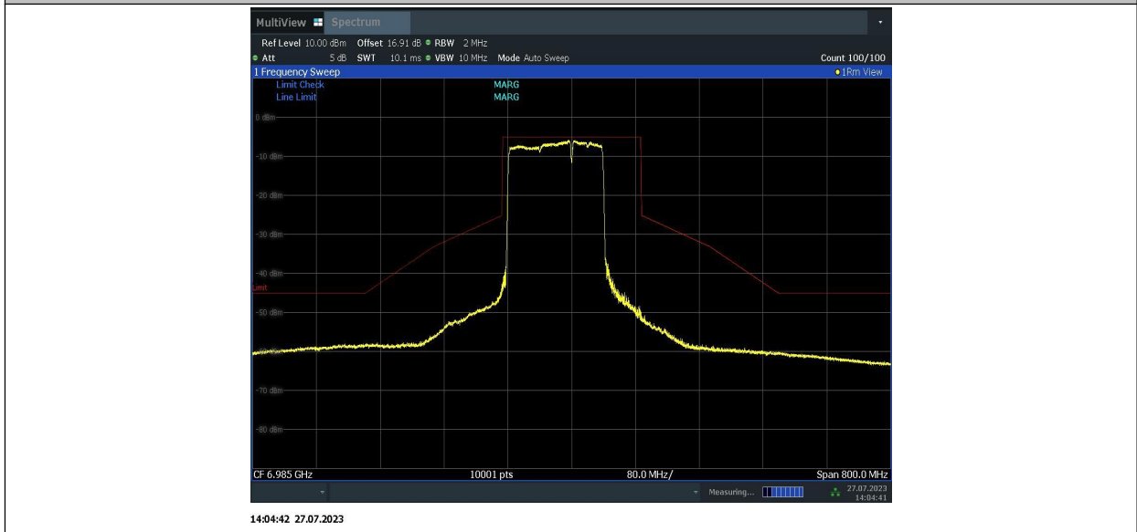
11BE160MIMO_Ant2_6985_996+484_4
