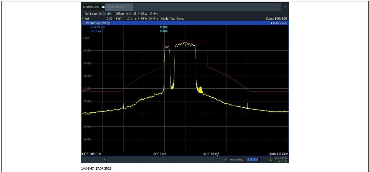
11BE320MIMO_Ant1_6105_996+996+484_3
