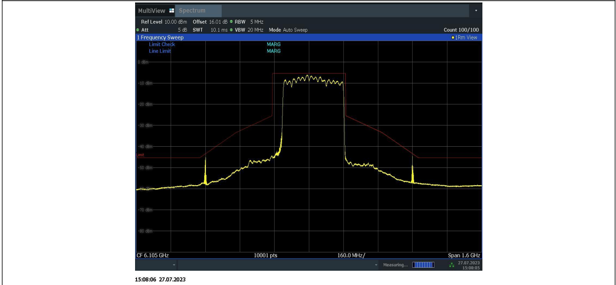
11BE320MIMO_Ant1_6105_996+996+996+484_2
