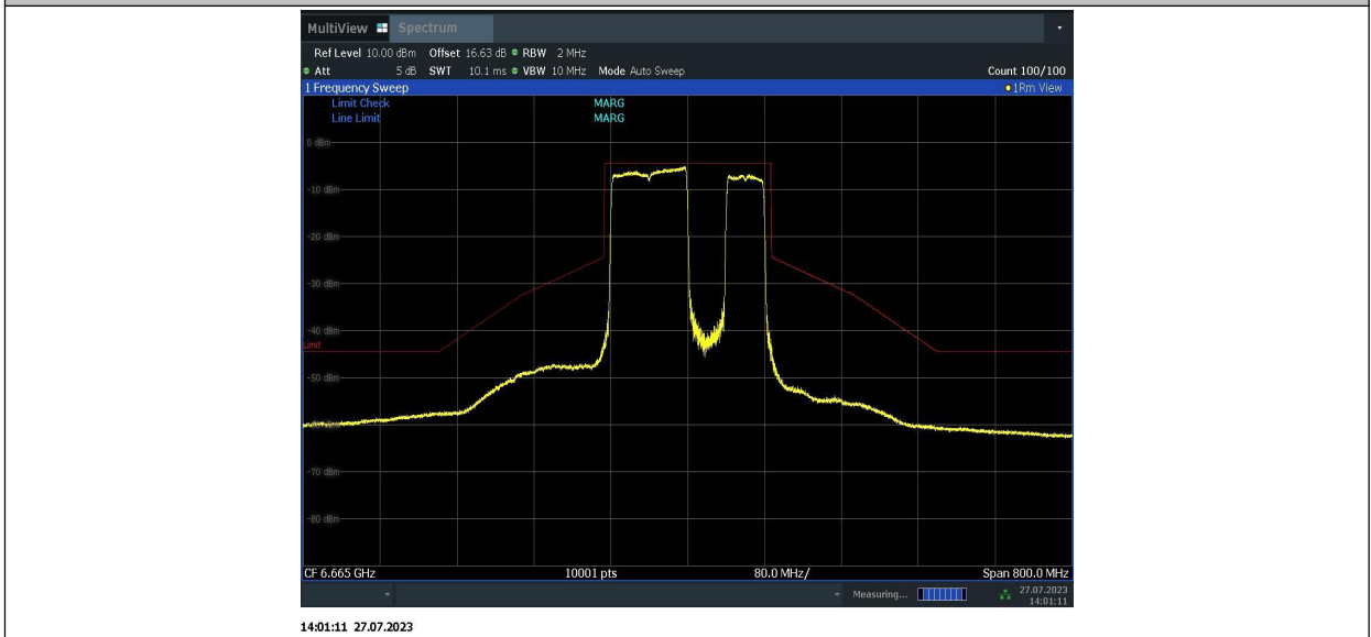
11BE160MIMO_Ant2_6665_996+484_3
