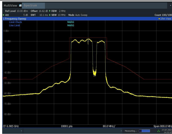
11BE160MIMO_Ant1_6985_996+484+242_6
