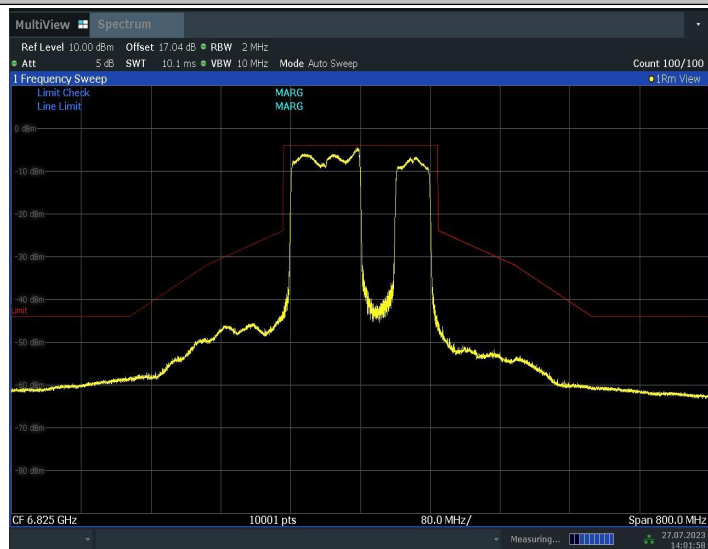
11BE160MIMO_Ant1_6825_996+484_3
