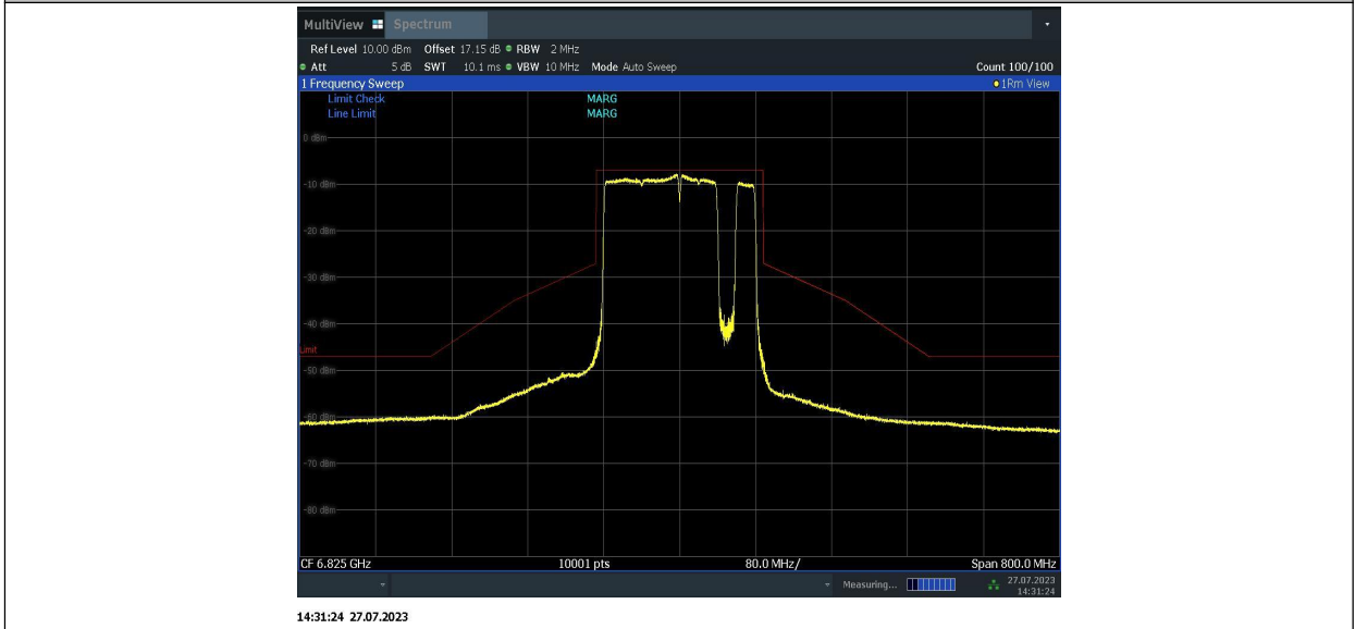
11BE160MIMO_Ant2_6825_996+484+242_7
