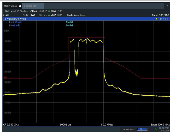
11BE160MIMO_Ant1_6985_996+484+242_2
