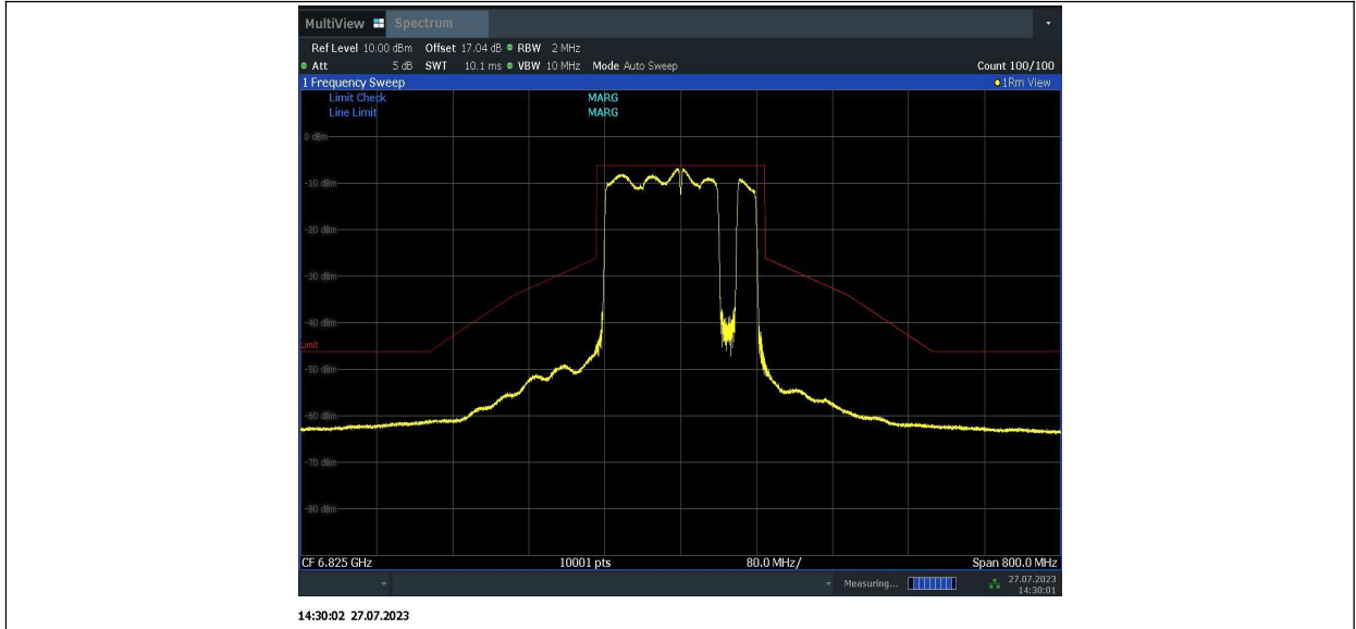
11BE160MIMO_Ant1_6825_996+484+242_8
