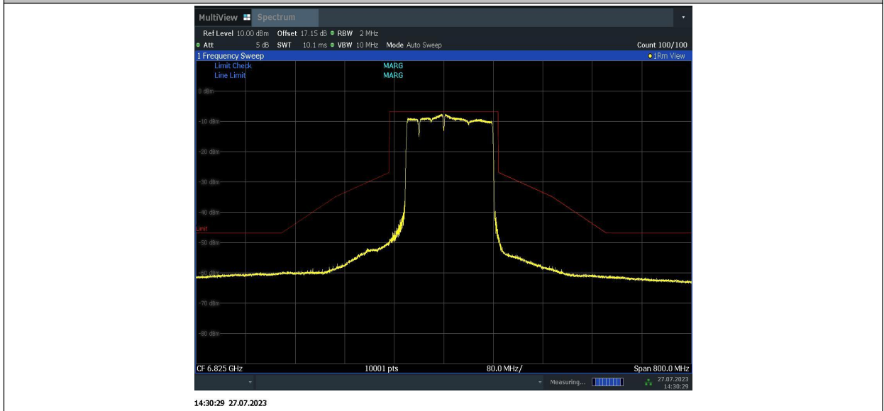
11BE160MIMO_Ant2_6825_996+484+242_2
