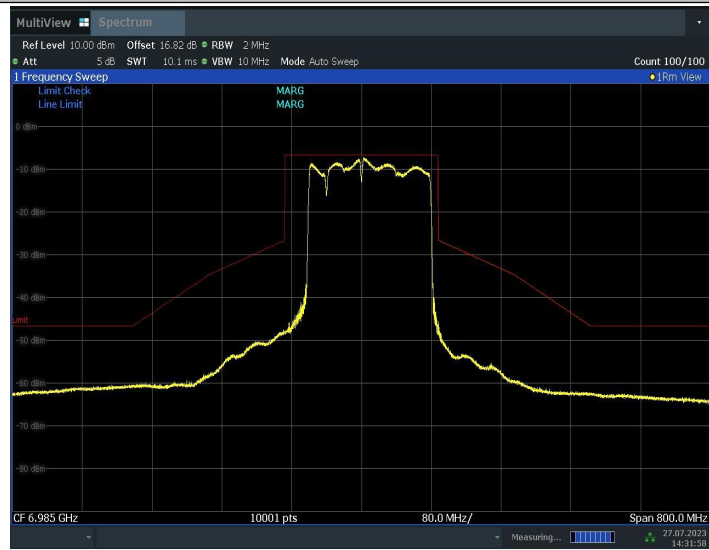
11BE160MIMO_Ant1_6985_996+484+242_1
