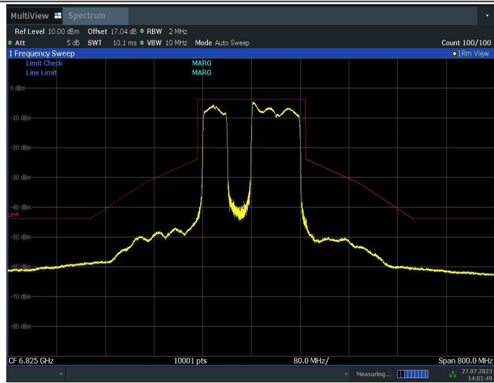
11BE160MIMO_Ant1_6825_996+484_2
