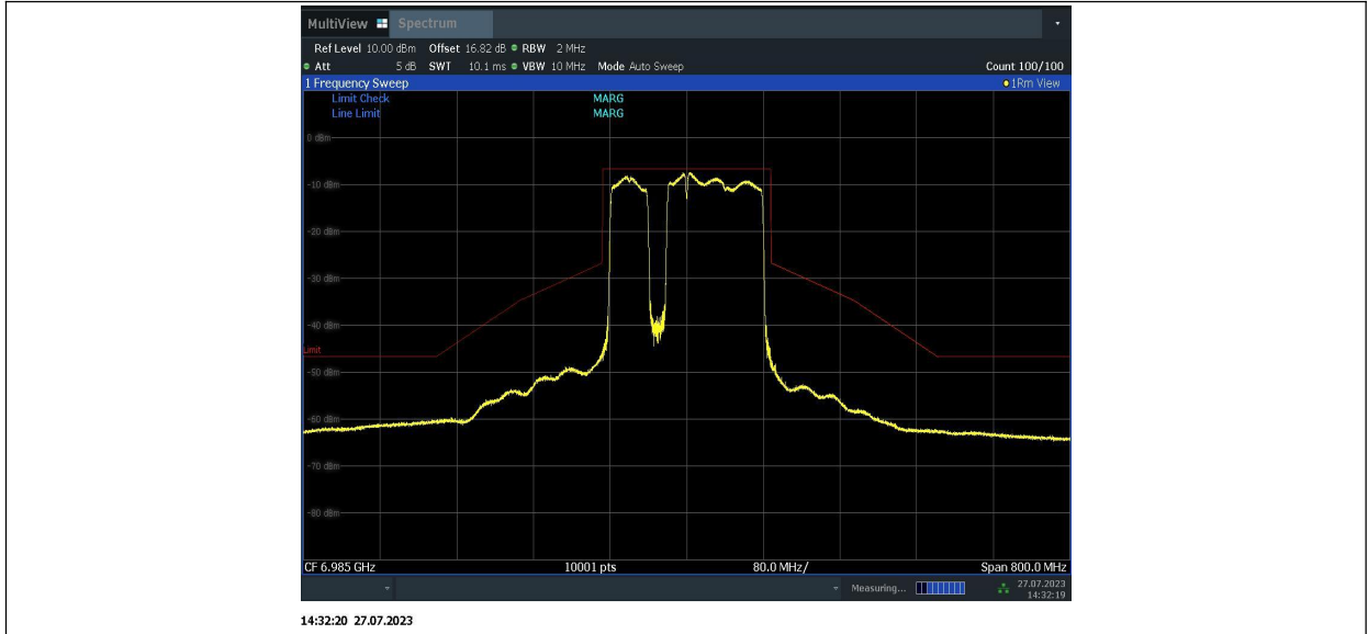
11BE160MIMO_Ant1_6985_996+484+242_4
