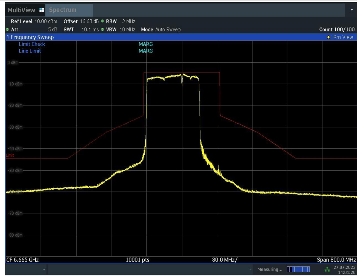
11BE160MIMO_Ant2_6665_996+484_4
