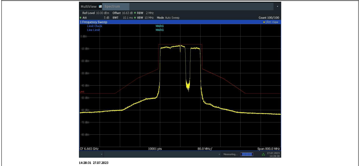
11BE160MIMO_Ant2_6665_996+484+242_6
