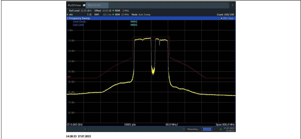
11BE160MIMO_Ant2_6665_996+484+242_6
