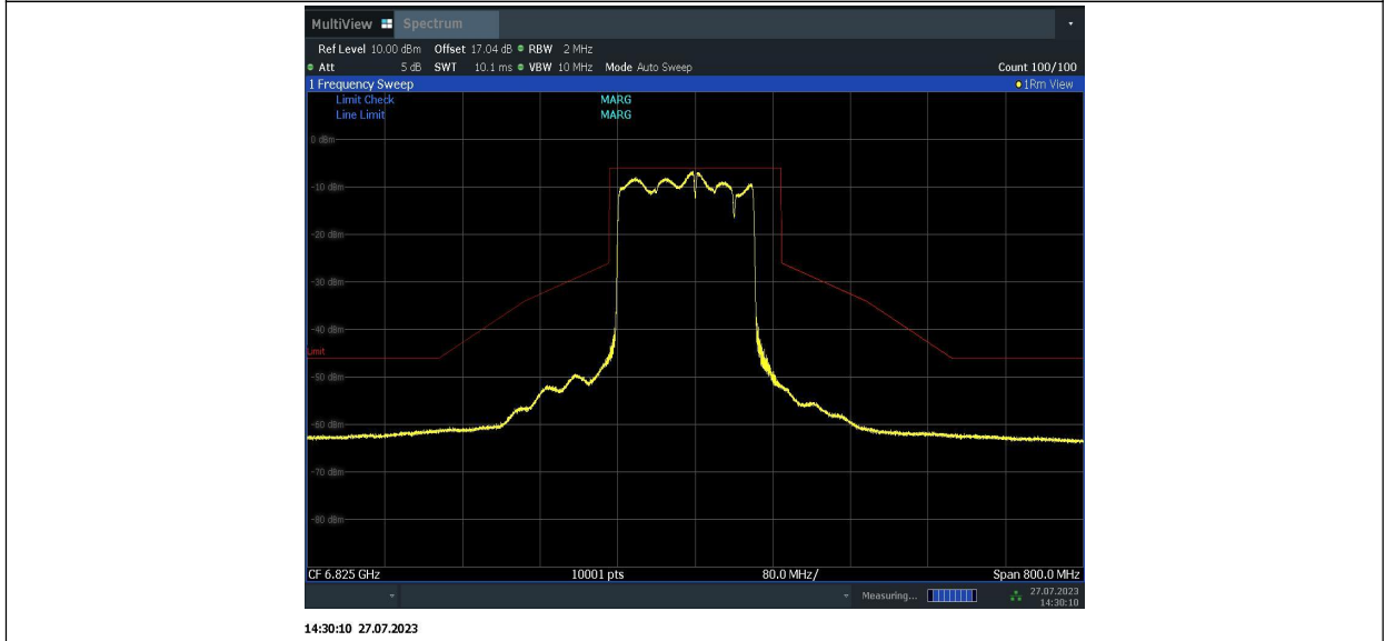
11BE160MIMO_Ant1_6825_996+484_1
