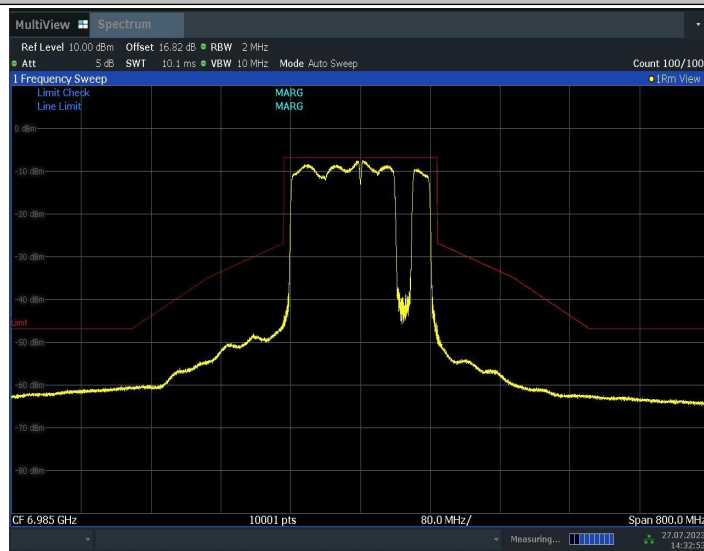
11BE160MIMO_Ant1_6985_996+484+242_7
