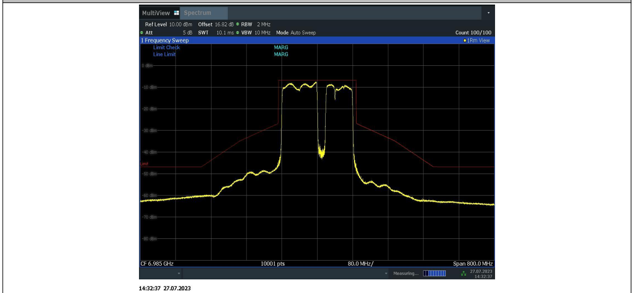
11BE160MIMO_Ant1_6985_996+484+242_5
