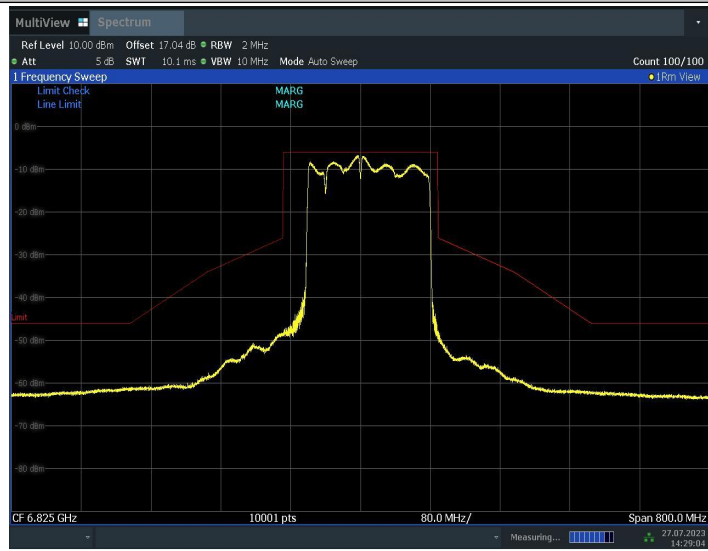
11BE160MIMO_Ant1_6825_996+484+242_1
