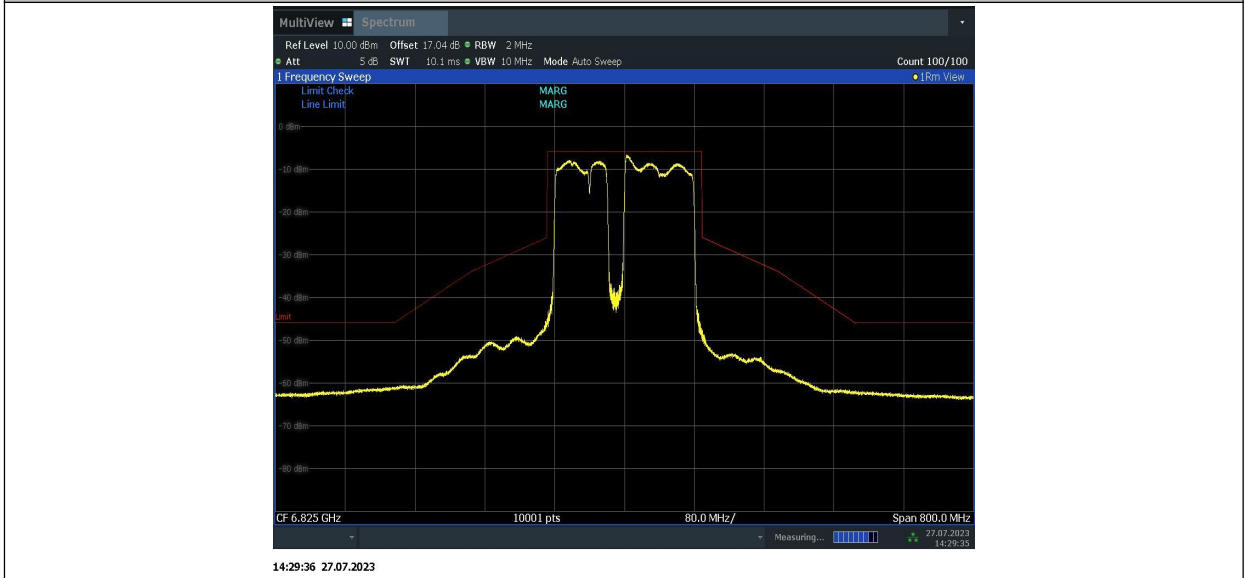
11BE160MIMO_Ant1_6825_996+484+242_4
