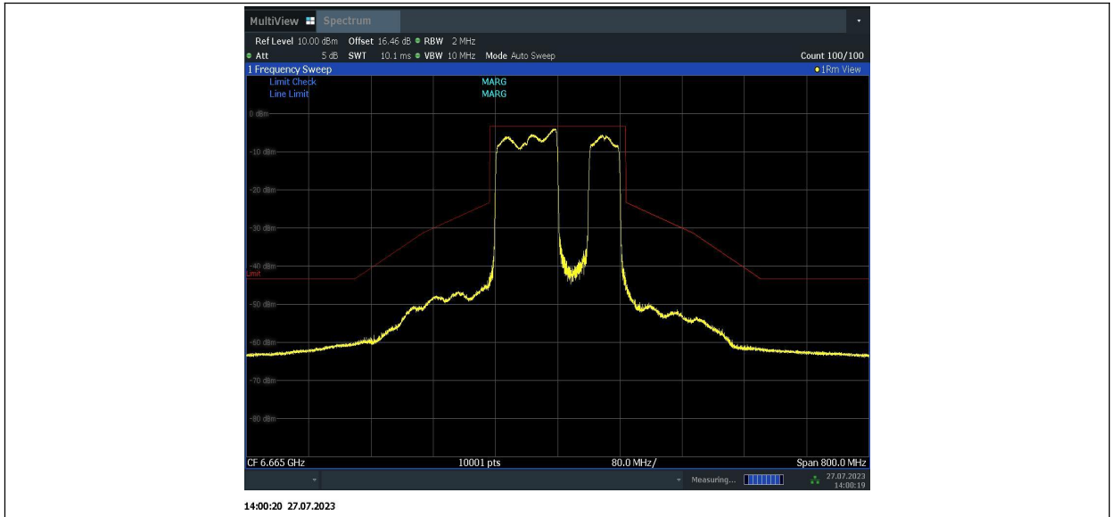
11BE160MIMO_Ant1_6665_996+484_4
