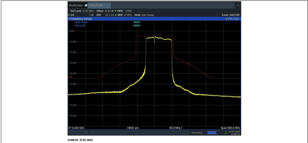
11BE160MIMO_Ant2_6665_996+484_2
