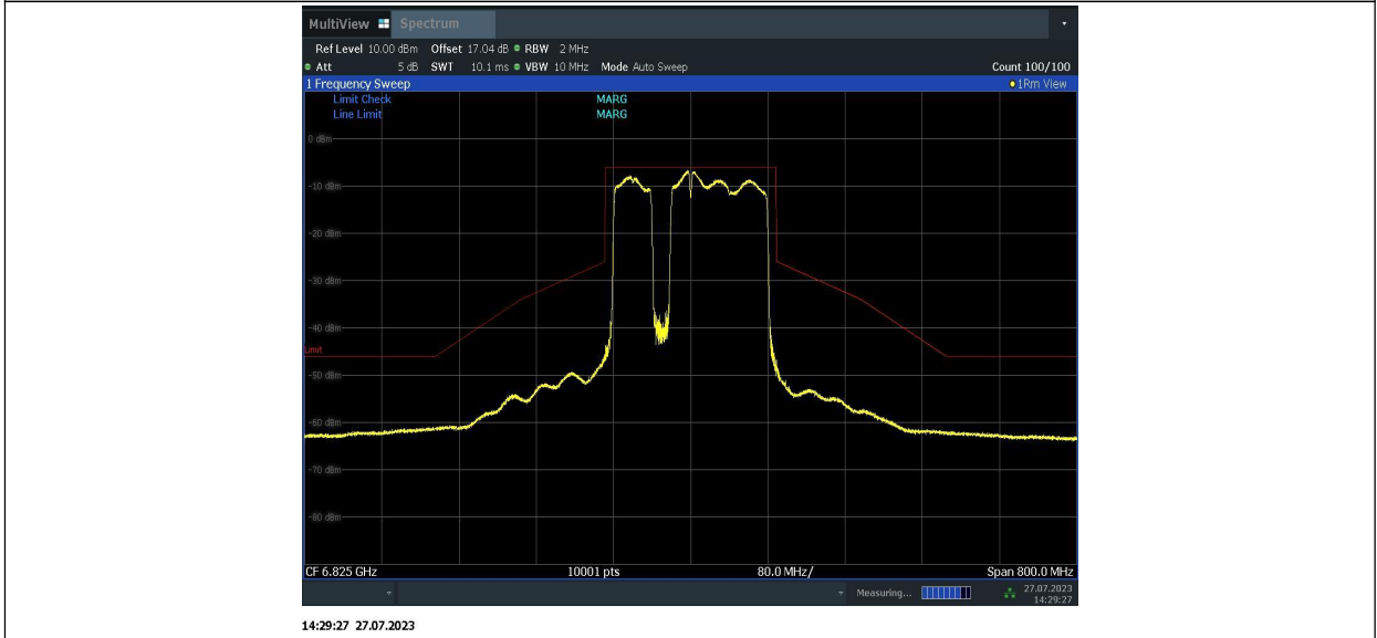
11BE160MIMO_Ant1_6825_996+484+242_4
