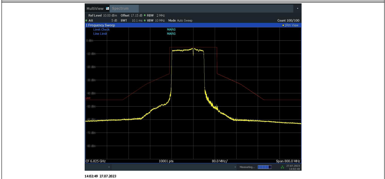
11BE160MIMO_Ant2_6825_996+484_4
