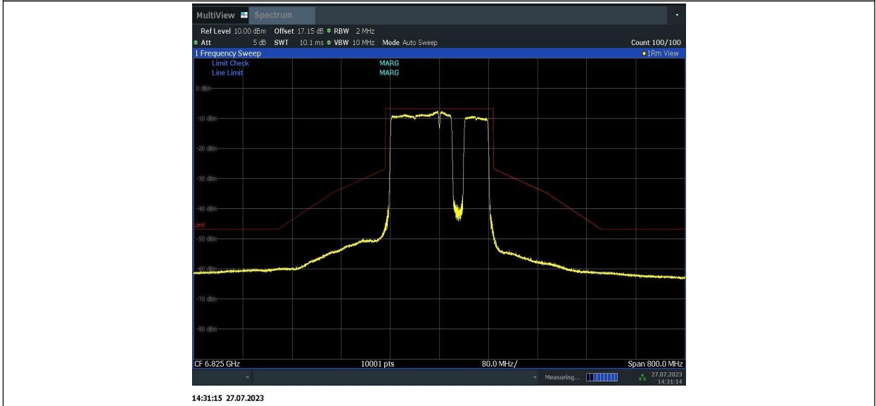
11BE160MIMO_Ant2_6825_996+484+242_7
