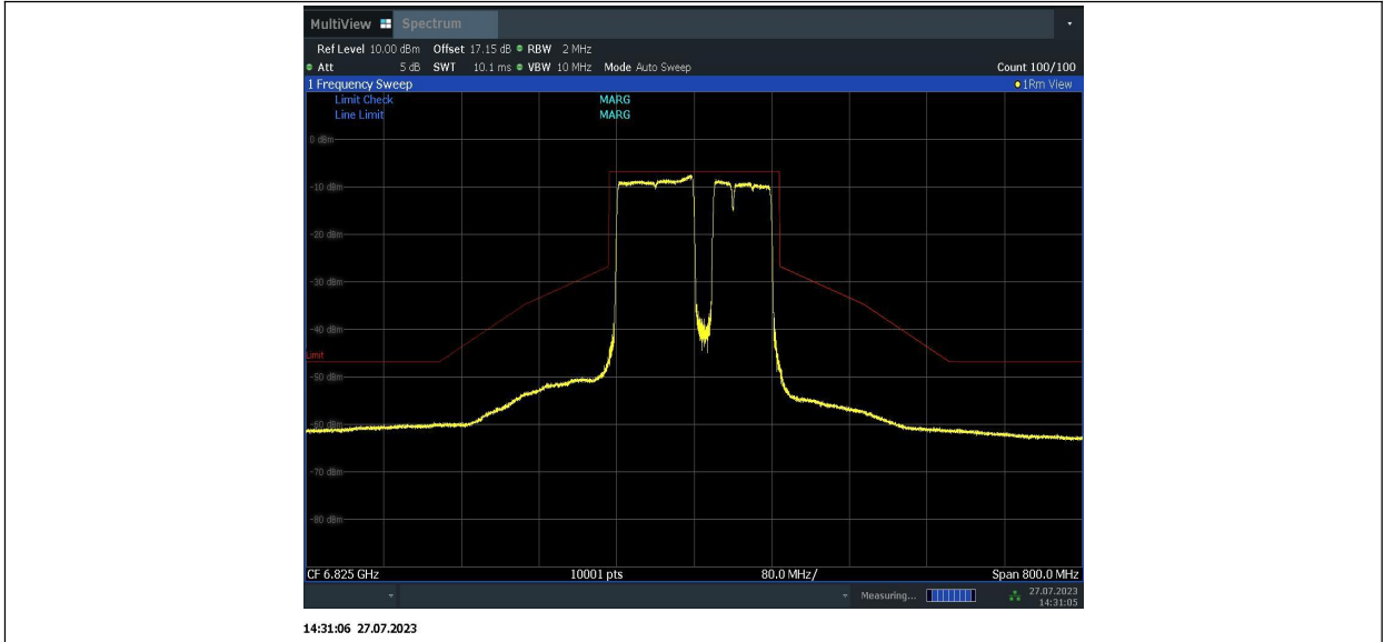
11BE160MIMO_Ant2_6825_996+484+242_6
