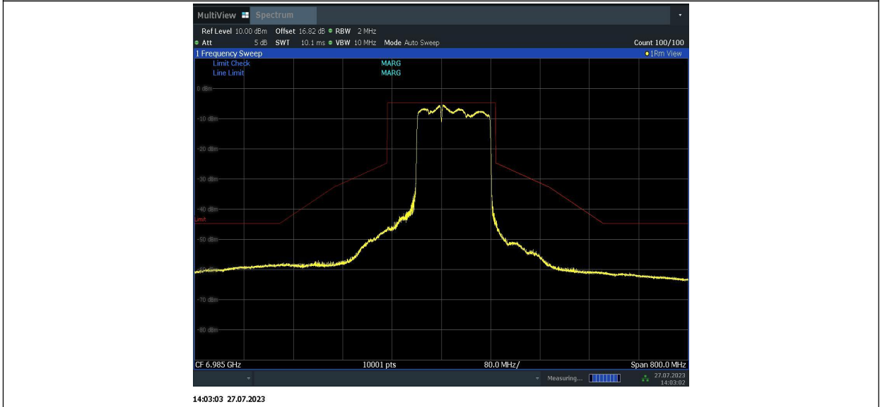
11BE160MIMO_Ant1_6985_996+484_2
