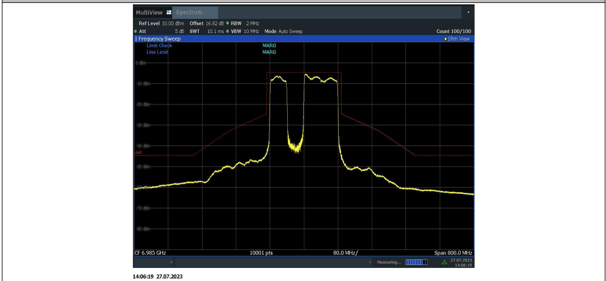
11BE160MIMO_Ant1_6985_996+484_2
