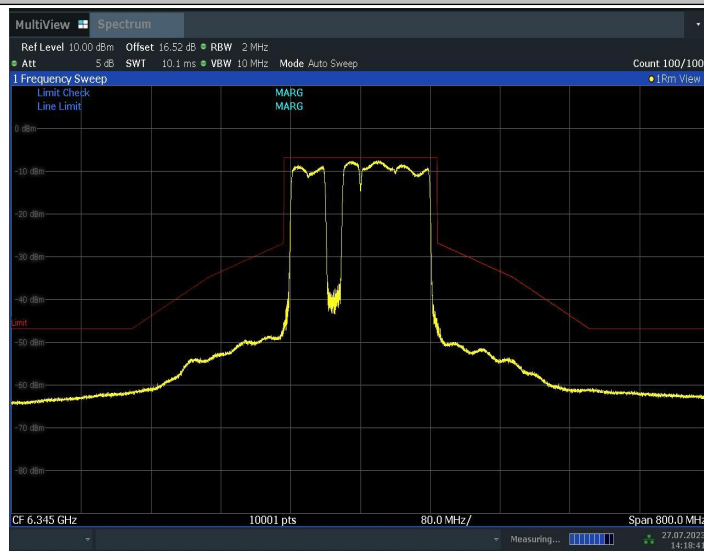
11BE160MIMO_Ant1_6345_996+484+242_3
