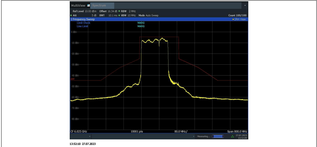
11BE160MIMO_Ant2_6025_996+484+242_1
