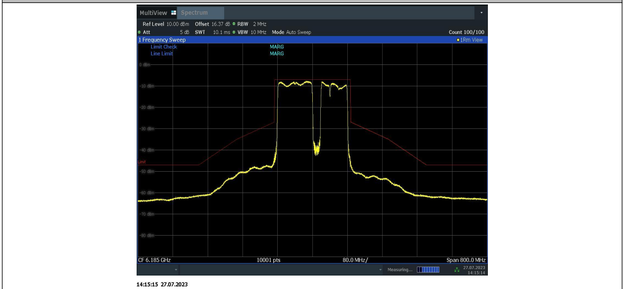
11BE160MIMO_Ant1_6185_996+484+242_5
