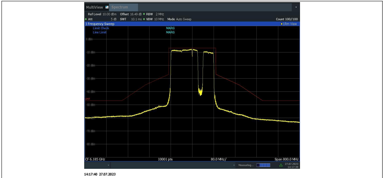
11BE160MIMO_Ant2_6185_996+484+242_7
