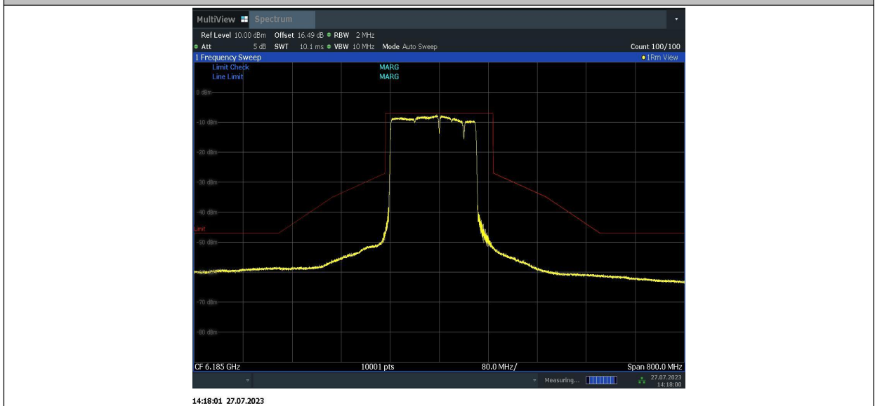
11BE160MIMO_Ant2_6185_996+484+242_8
