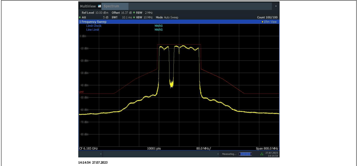
11BE160MIMO_Ant1_6185_996+484+242_4
