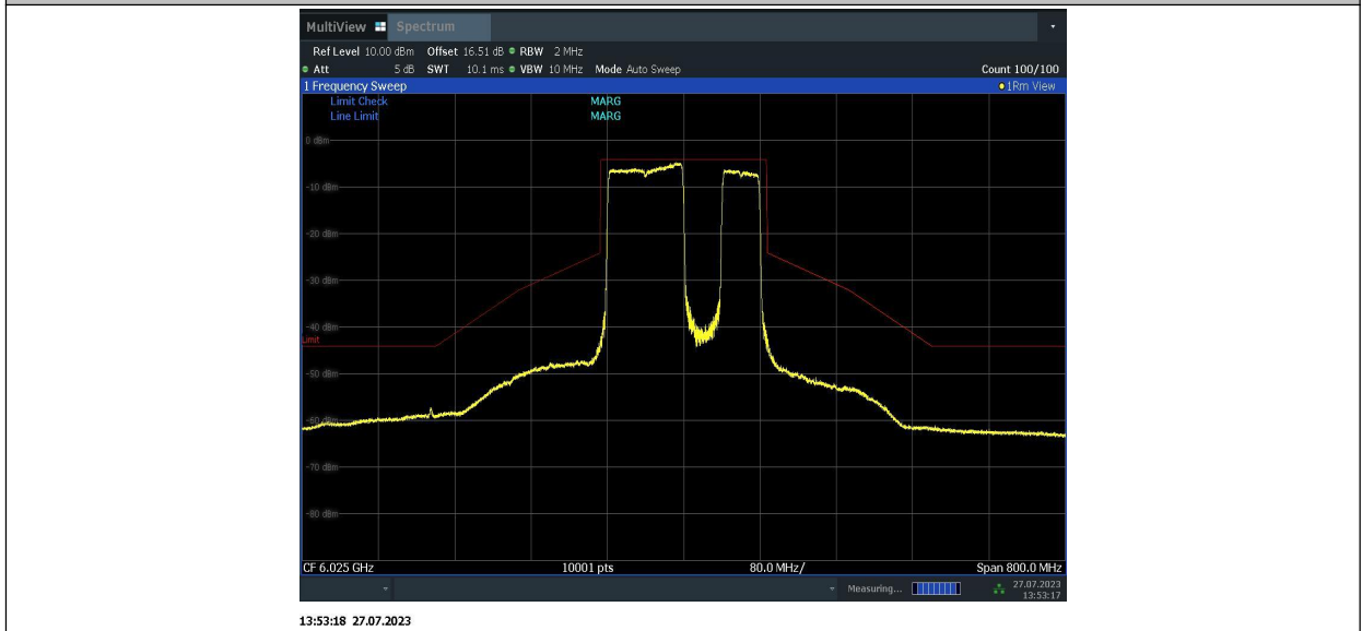
11BE160MIMO_Ant2_6025_996+484_4
