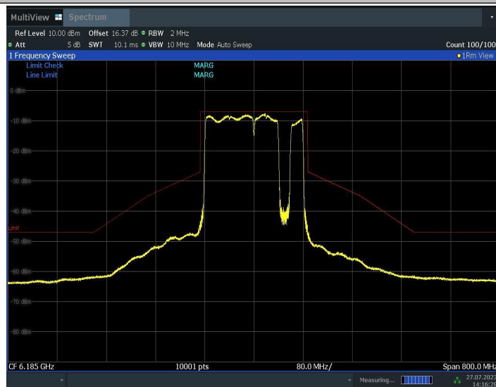
11BE160MIMO_Ant1_6185_996+484+242_7
