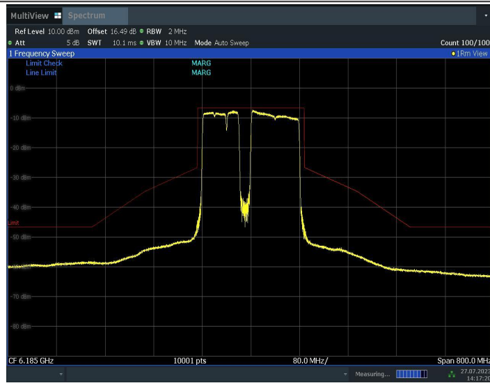
11BE160MIMO_Ant2_6185_996+484+242_4
