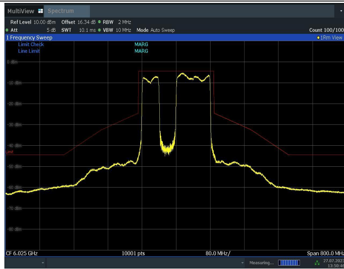
11BE160MIMO_Ant1_6025_996+484_2
