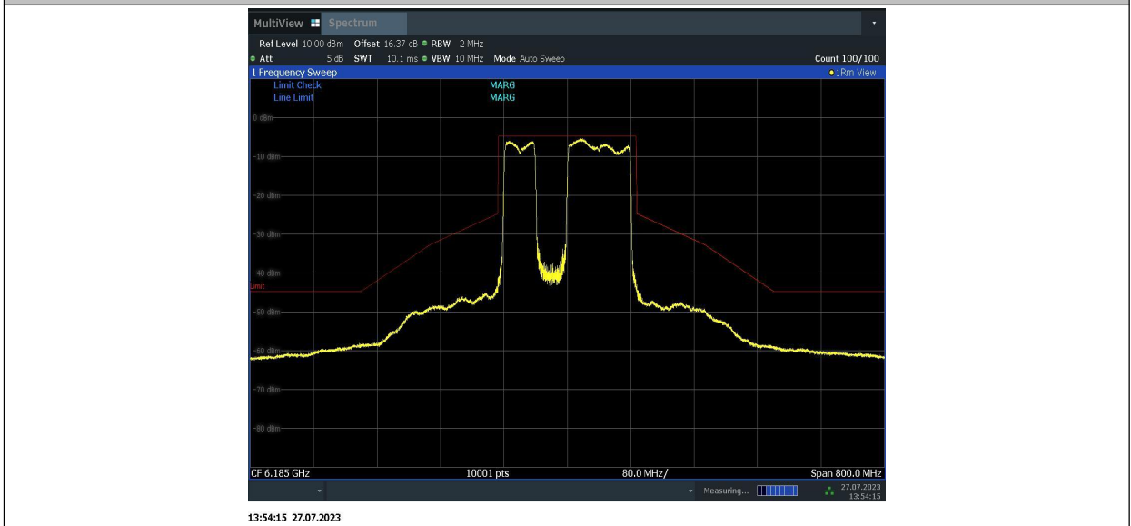
11BE160MIMO_Ant1_6185_996+484_2
