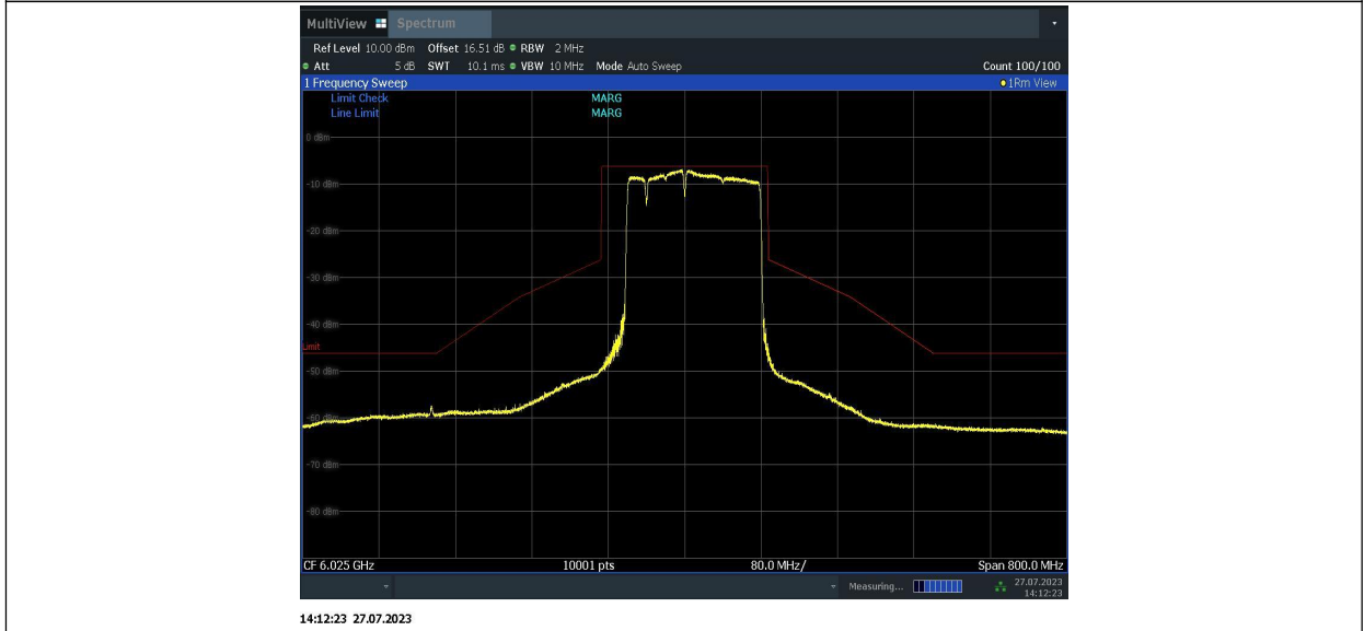
11BE160MIMO_Ant2_6025_996+484+242_2
