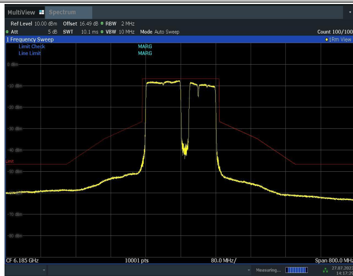
11BE160MIMO_Ant2_6185_996+484+242_5
