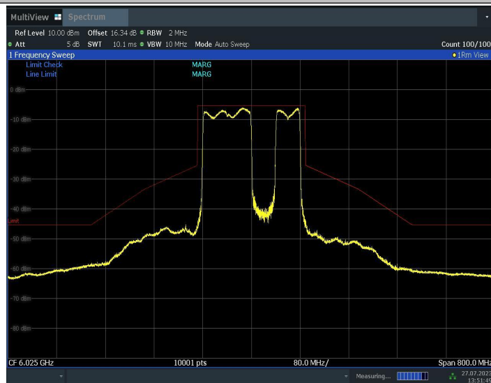
11BE160MIMO_Ant1_6025_996+484_3
