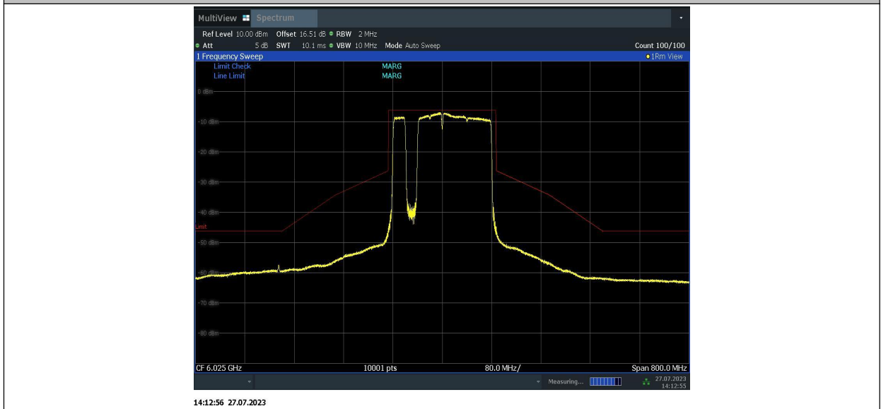
11BE160MIMO_Ant2_6025_996+484+242_2
