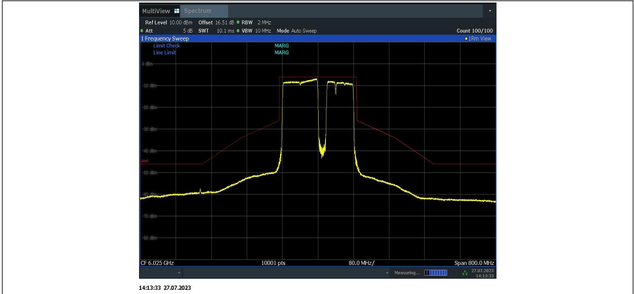
11BE160MIMO_Ant2_6025_996+484+242_6
