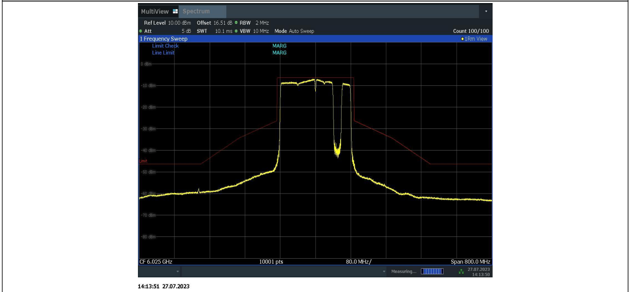
11BE160MIMO_Ant2_6025_996+484+242_7
