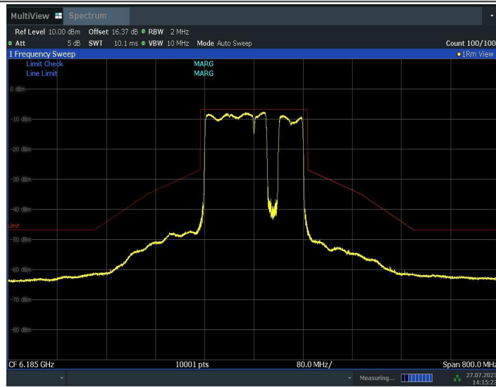
11BE160MIMO_Ant1_6185_996+484+242_6
