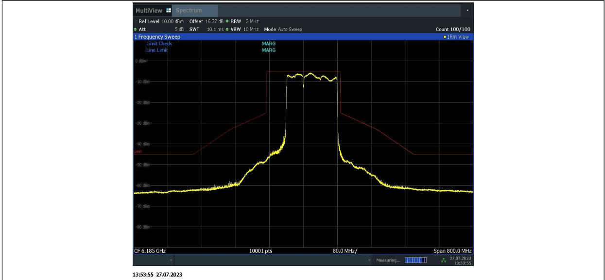
11BE160MIMO_Ant1_6185_996+484_2
