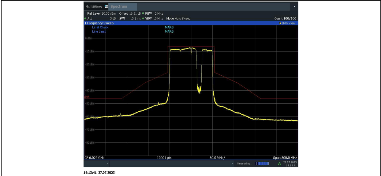
11BE160MIMO_Ant2_6025_996+484+242_7
