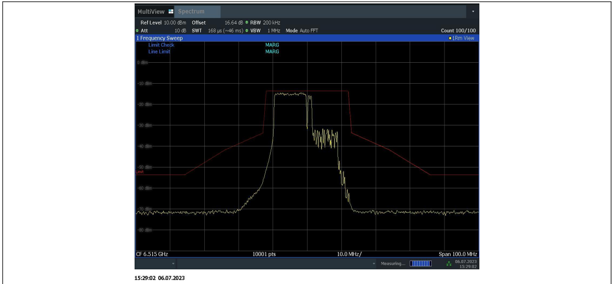
11BE20MIMO_Ant2_6515_52 Tone,index38 + 26Tone,index1
