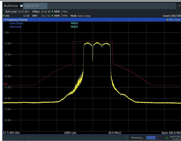
11BE80MIMO_Ant1_5985_484+242_1
