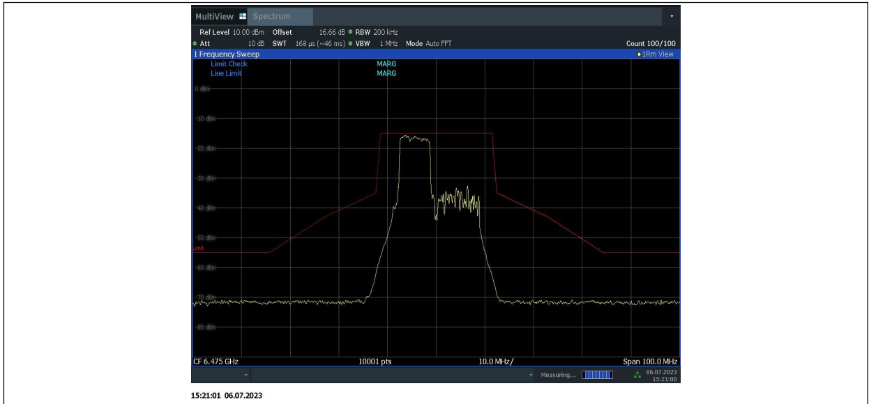
11BE20MIMO_Ant2_6475_106 Tone,index53 + 26Tone,index4
