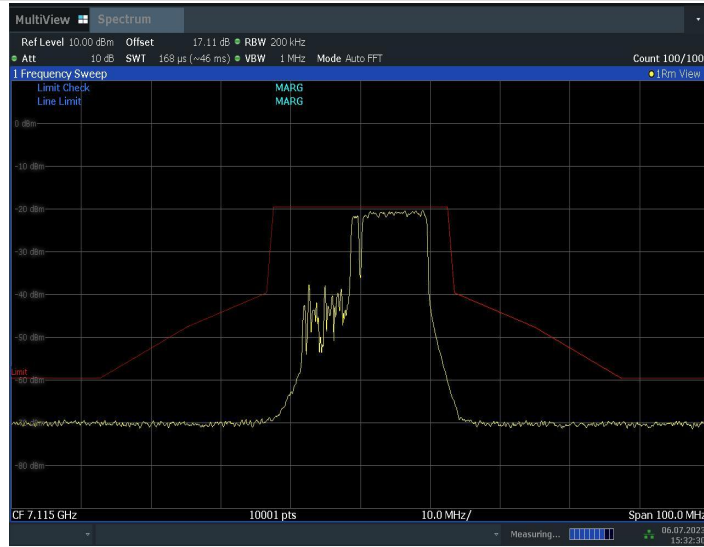
11BE20MIMO_Ant2_7115_106 Tone,index54 + 26Tone,index4
