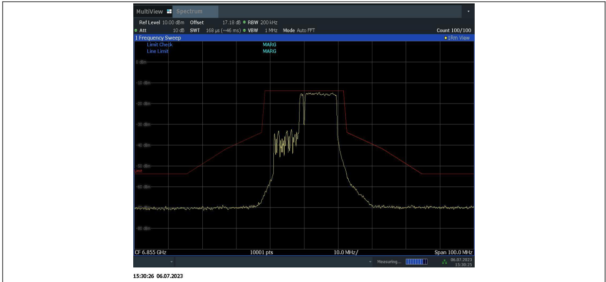
11BE20MIMO_Ant1_6855_52 Tone,index39 + 26Tone,index7
