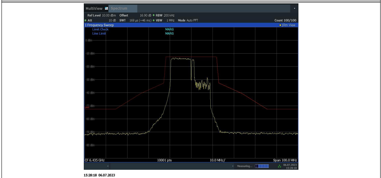
11BE20MIMO_Ant2_6435_106 Tone,index53 + 26Tone,index4
