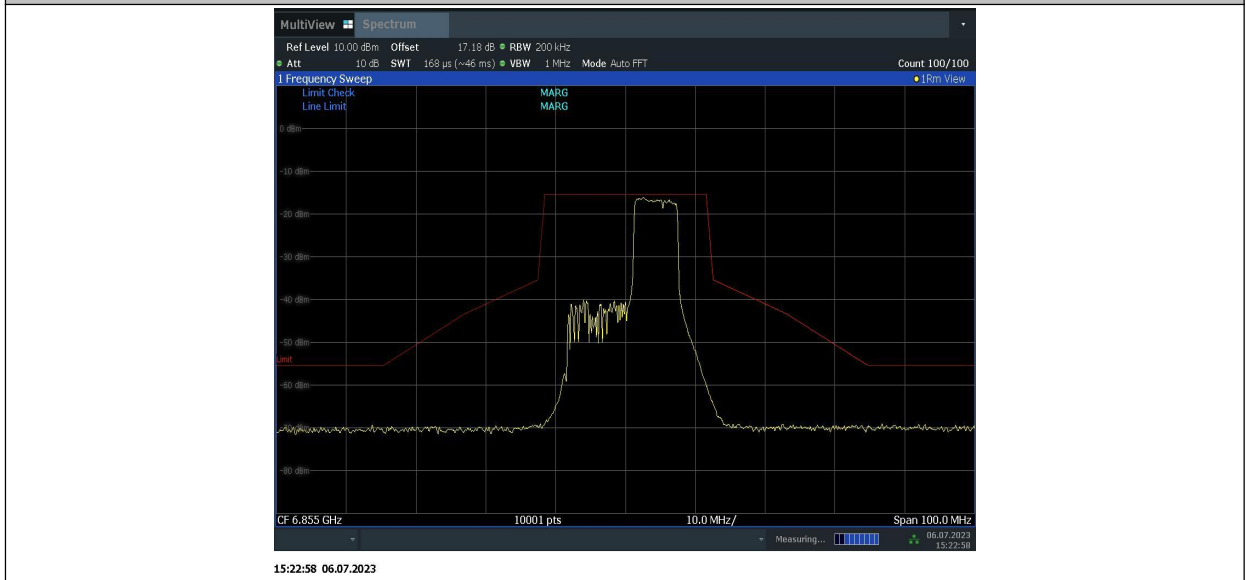
11BE20MIMO_Ant2_6855_106 Tone,index54 + 26Tone,index4
