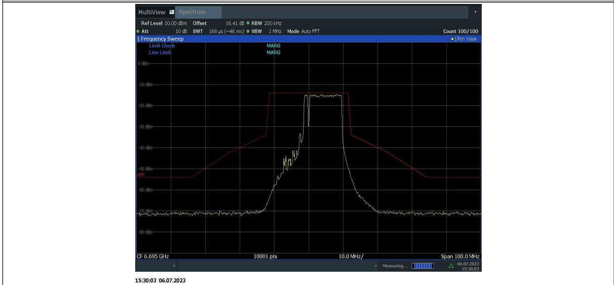
11BE20MIMO_Ant1_6695_52 Tone,index39 + 26Tone,index7
