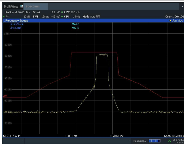
11BE20MIMO_Ant2_7115_52 Tone,index39 + 26Tone,index7
