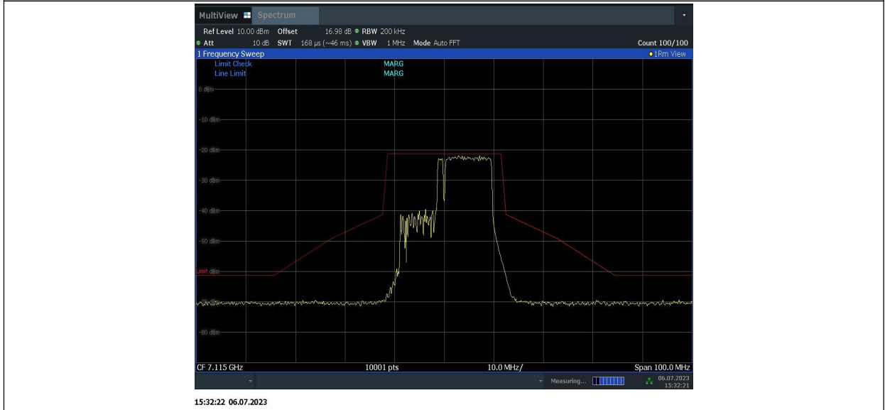
11BE20MIMO_Ant1_7115_52 Tone,index39 + 26Tone,index7
