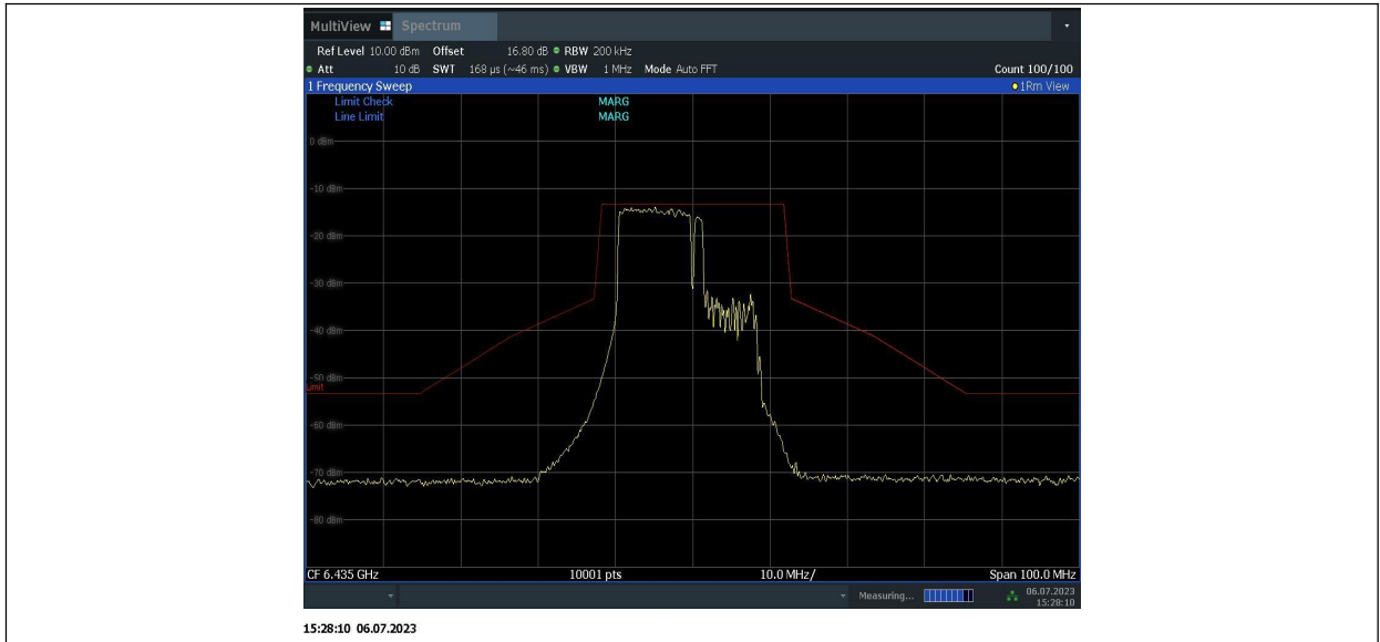
11BE20MIMO_Ant1_6435_52 Tone,index38 + 26Tone,index1
