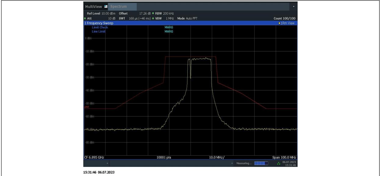
11BE20MIMO_Ant2_6895_52 Tone,index39 + 26Tone,index7
