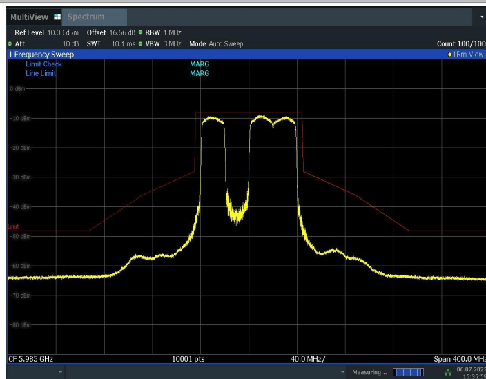
11BE80MIMO_Ant1_5985_484+242_2
