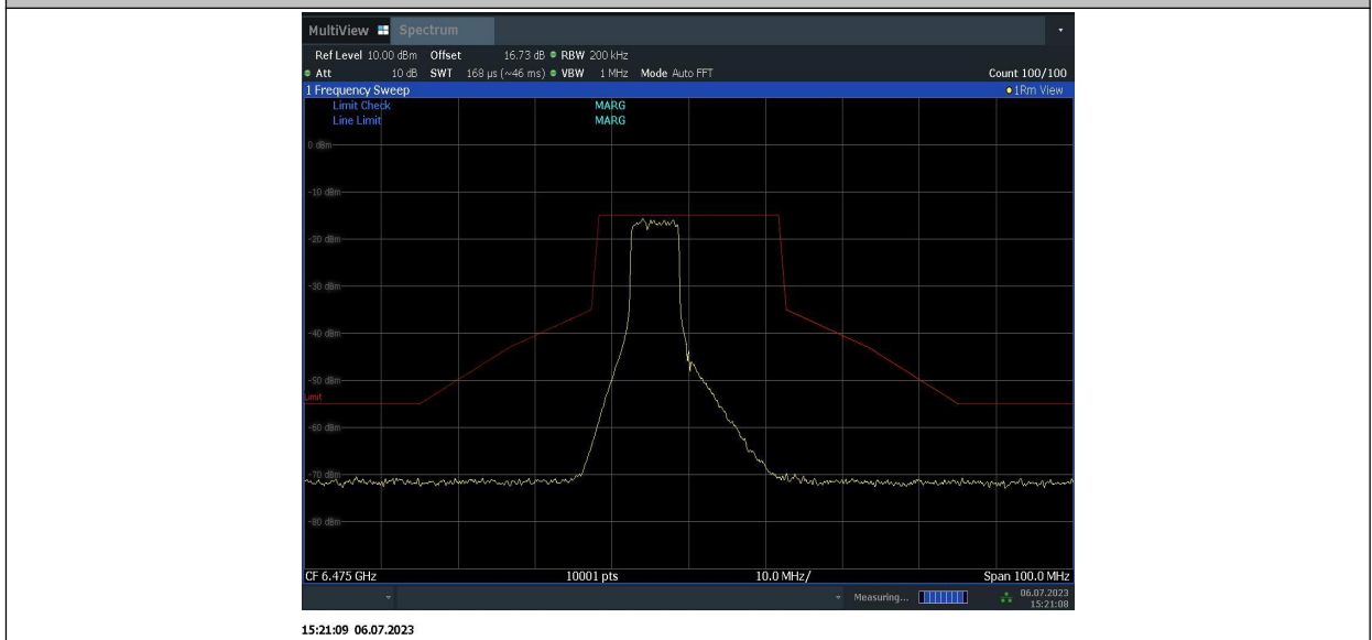
11BE20MIMO_Ant2_6475_52 Tone,index38 + 26Tone,index1
