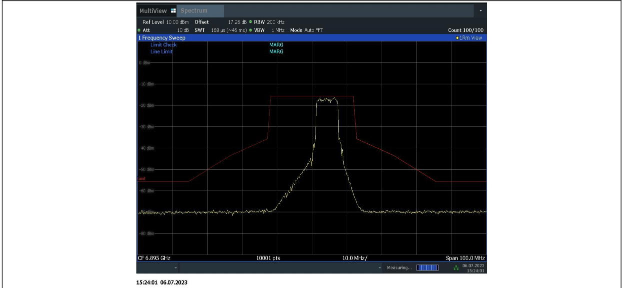
11BE20MIMO_Ant1_6995_106 Tone,index54 + 26Tone,index4
