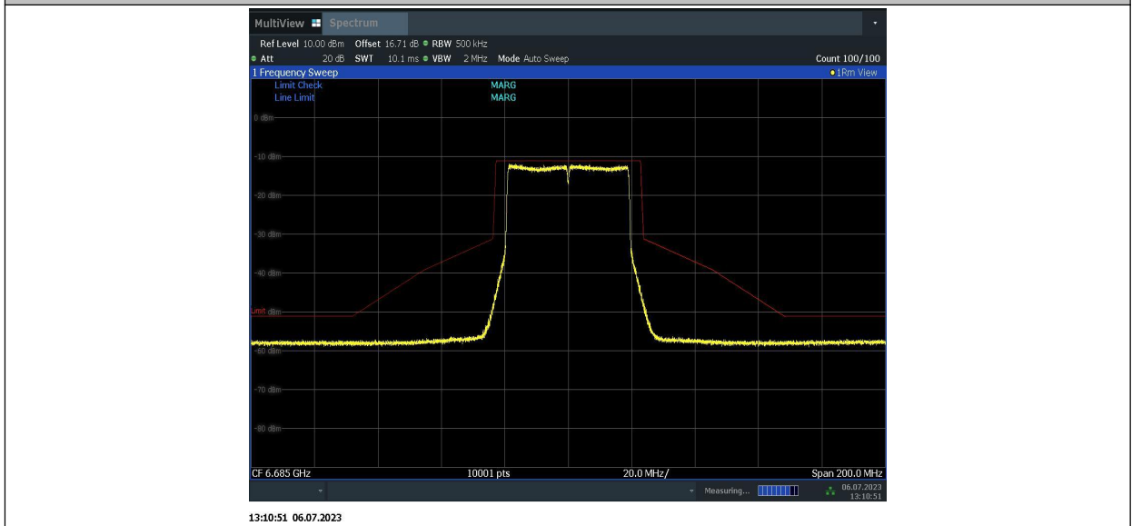
11BE40MIMO_Ant2_6685
