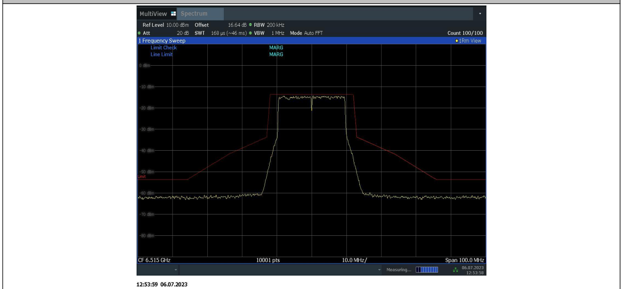
11BE20MIMO_Ant2_6515
