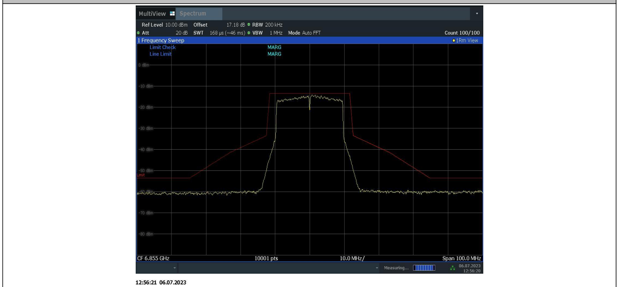
11BE20MIMO_Ant1_6855
