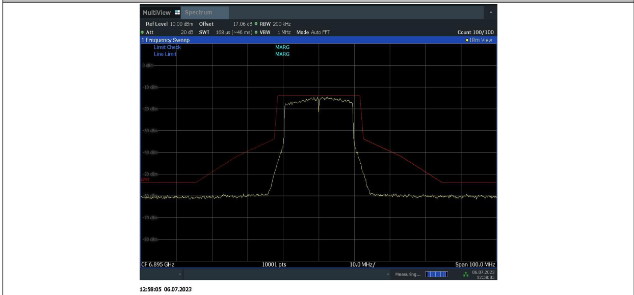
11BE20MIMO_Ant2_6895
