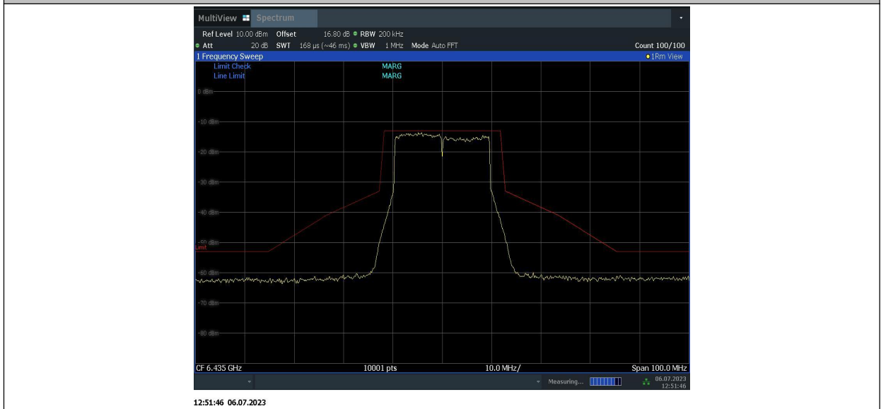
11BE20MIMO_Ant1_6435
