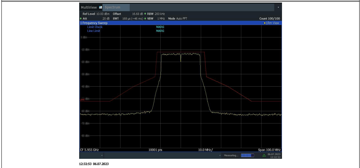
11BE20MIMO_Ant2_5955
