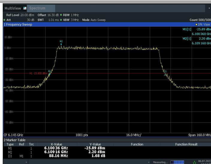
11BE80MIMO_Ant2_6145
