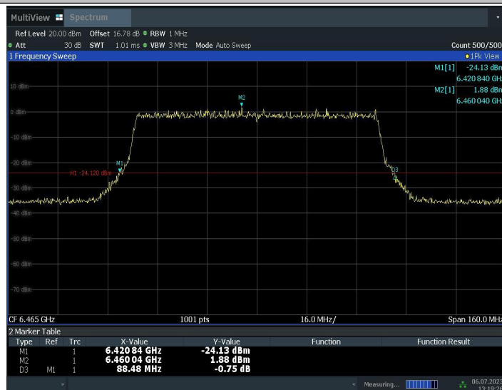
11BE80MIMO_Ant2_6465
