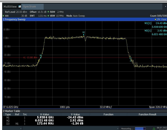
11BE160MIMO_Ant2_6025
