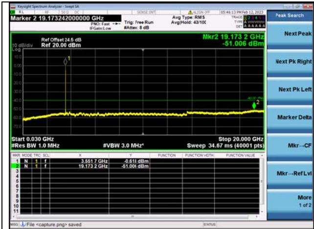
Band48C-30M-20G / 20MHz+10MHz /1RB+1RB/ QPSK / Low CH
