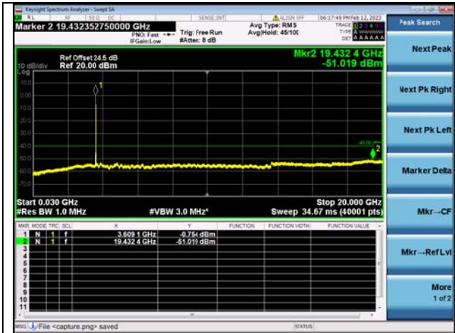
Band48C-30M-20G / 20MHz+15MHz /1RB+1RB/ QPSK / Mid CH
