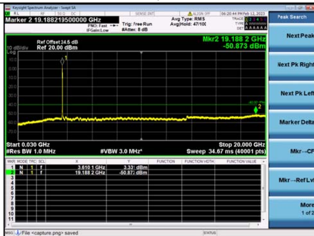
Band48C-30M-20G / 20MHz+15MHz /100RB+75RB/ QPSK / Mid CH
