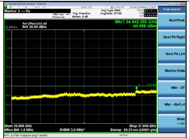
Band48C-20G-37G / 20MHz+15MHz /1RB+1RB/ QPSK / Low CH
