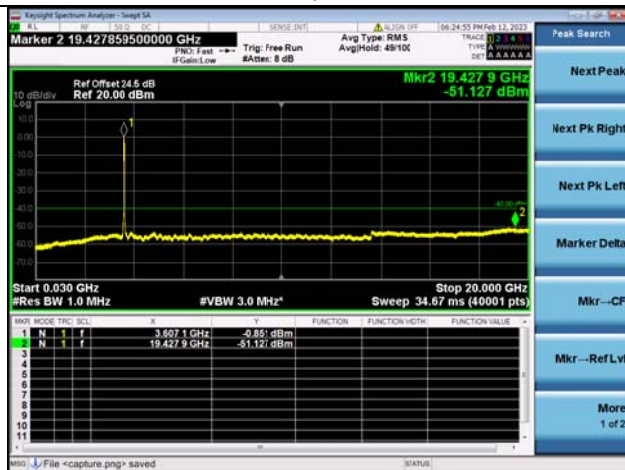
Band48C-30M-20G / 20MHz+20MHz /100RB+100RB/ QPSK / Mid CH
