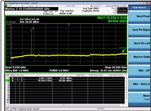
Band48C-30M-20G / 10MHz+20MHz /1RB+1RB/ QPSK / Low CH
