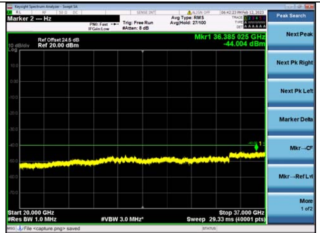
Band48C-20G-37G / 20MHz+15MHz /1RB+1RB/ QPSK / High CH
