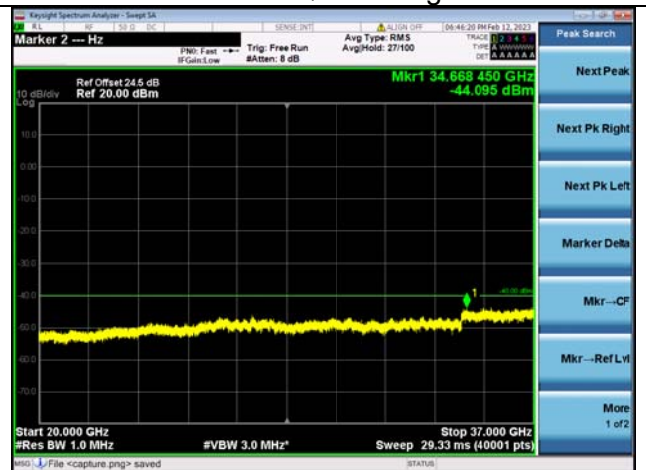
Band48C-20G-37G / 20MHz+20MHz /100RB+100RB/ QPSK / High CH
