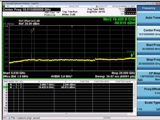
Band48C-30M-20G / 20MHz+20MHz / 1RB+1RB/ QPSK / Low CH
