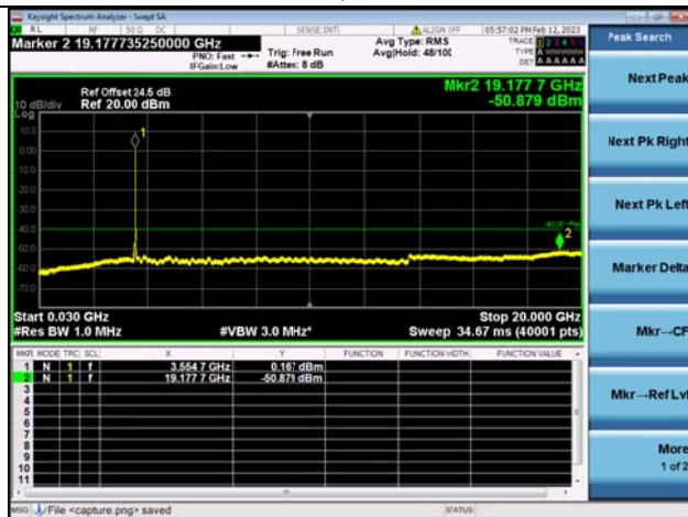
Band48C-30M-20G / 20MHz+15MHz /100RB+75RB/ QPSK / Low CH
