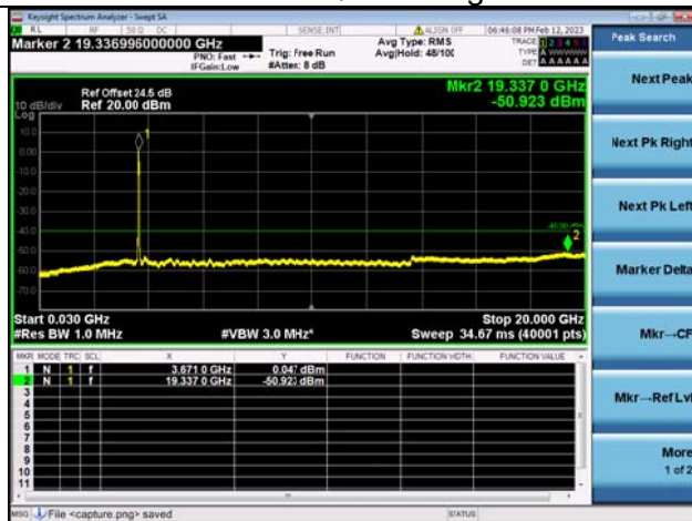
Band48C-30M-20G / 20MHz+20MHz /100RB+100RB/ QPSK / High CH
