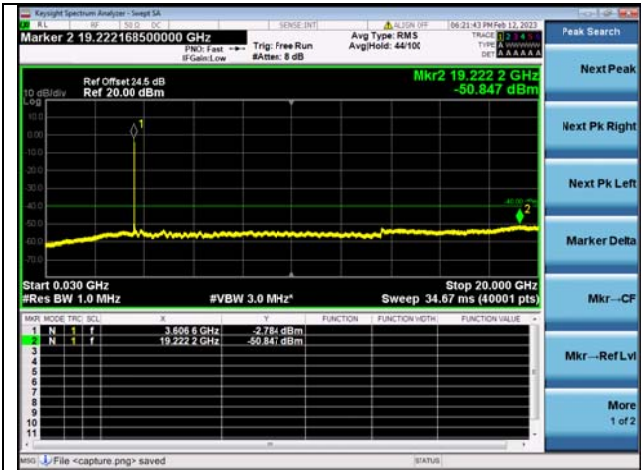
Band48C-30M-20G / 20MHz+20MHz /1RB+1RB/ QPSK / Mid CH
