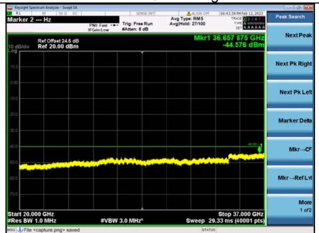
Band48C-20G-37G / 20MHz+15MHz /100RB+75RB/ QPSK / High CH
