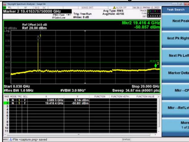
Band48C-30M-20G / 20MHz+10MHz /1RB+1RB/ QPSK / High CH
