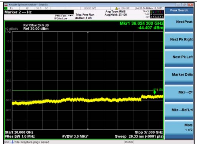
Band48C-20G-37G / 20MHz+15MHz /100RB+75RB/ QPSK / Mid CH
