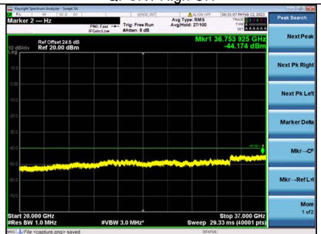
Band48C-20G-37G / 20MHz+5MHz / 100RB+25RB / QPSK / High CH
