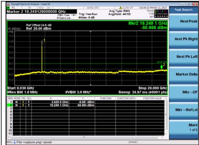
Band48C-30M-20G / 20MHz+10MHz /1RB+1RB/ QPSK / Mid CH
