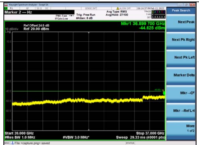
Band48C-20G-37G / 15MHz+20MHz / 1RB+1RB/ QPSK / Mid CH
