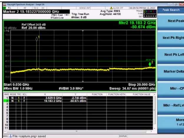
Band48C-30M-20G / 20MHz+10MHz /1RB+1RB/ QPSK / Mid CH
