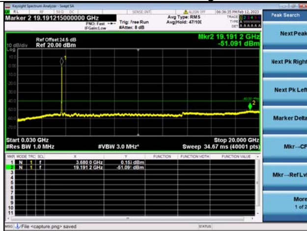
Band48C-30M-20G / 20MHz+10MHz /100RB+50RB/ QPSK / High CH
