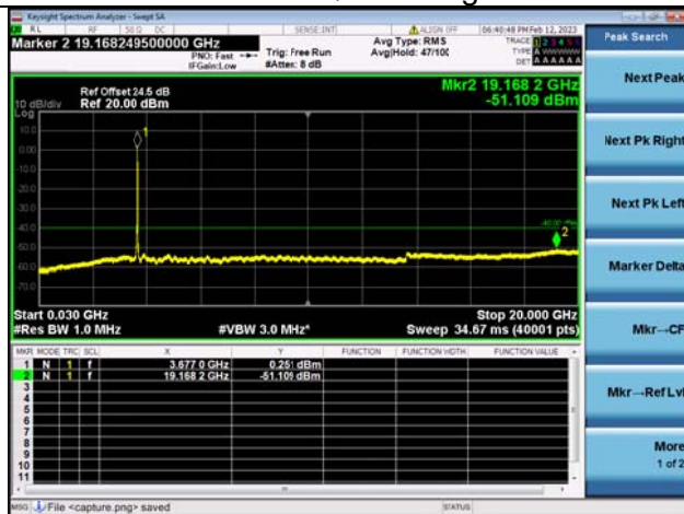
Band48C-30M-20G / 15MHz+20MHz /75RB+100RB/ QPSK / High CH
