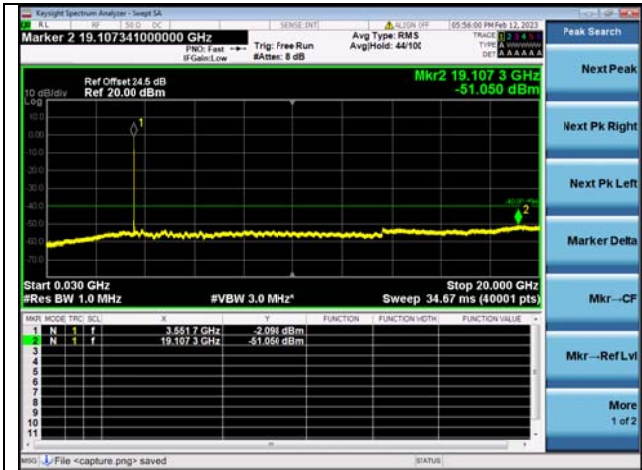
Band48C-30M-20G / 20MHz+15MHz /1RB+1RB/ QPSK / Low CH
