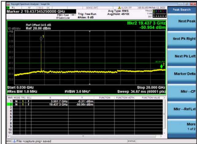
Band48C-30M-20G / 15MHz+20MHz /1RB+1RB/ QPSK / Low CH
