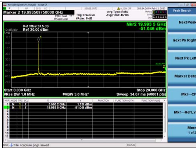
Band48C-30M-20G / 15MHz+20MHz /75RB+100RB/ QPSK / Low CH
