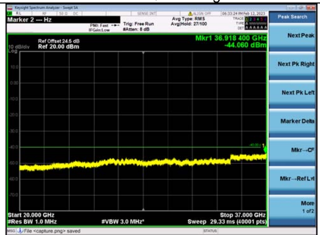
Band48C-20G-37G / 10MHz+20MHz /1RB+1RB/ QPSK / High CH
