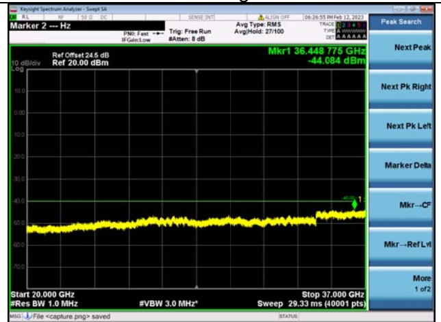
Band48C-20G-37G / 5MHz+20MHz / 1RB+1RB / QPSK / High CH
