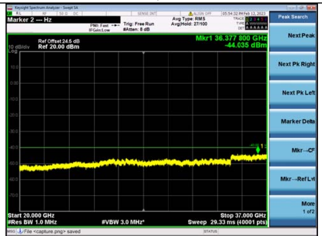
Band48C-20G-37G / 15MHz+20MHz /75RB+100RB/ QPSK / Low CH
