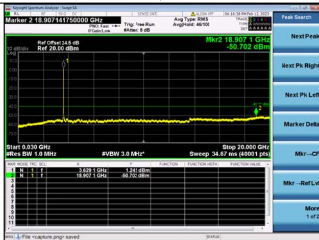
Band48C-30M-20G / 20MHz+10MHz /100RB+50RB/ QPSK / Mid CH
