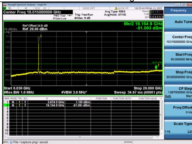
Band48C-30M-20G / 20MHz+15MHz /100RB+75RB/ QPSK / High CH
