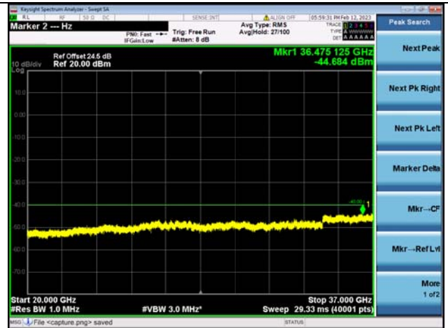
Band48C-20G-37G / 20MHz+20MHz / 1RB+1RB/ QPSK / Low CH
