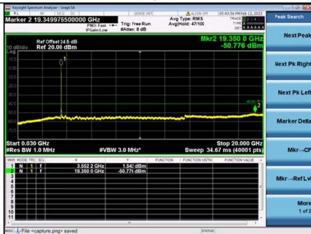
Band48C-30M-20G / 10MHz+20MHz /50RB+100RB/ QPSK / Low CH
