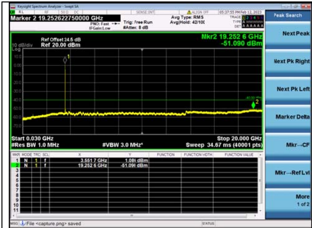
Band48C-30M-20G / 20MHz+5MHz / 1RB+1RB / QPSK / Low CH
