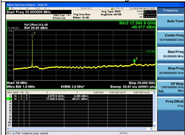
Band41C-30M-20G / 15MHz+10MHz /75RB+50RB/ QPSK / High CH
