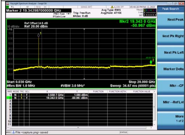
Band48C-30M-20G / 20MHz+5MHz / 100RB+25RB / QPSK / Low CH
