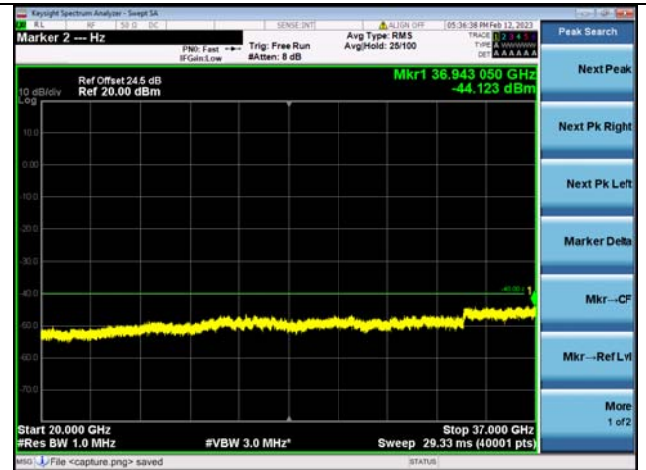
Band48C-20G-37G / 5MHz+20MHz / 1RB+1RB / QPSK / Low CH
