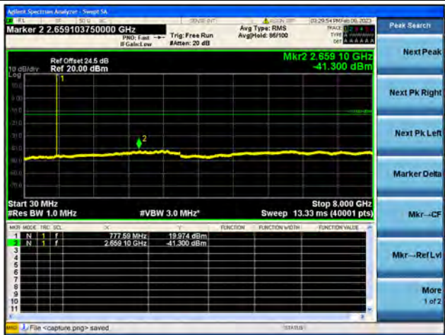
Band13 / 5MHz / Low CH / 64QAM
