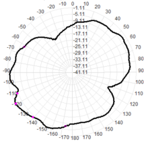
2480.0MHz Total(E1-XZ), Max=-1.23dBi
