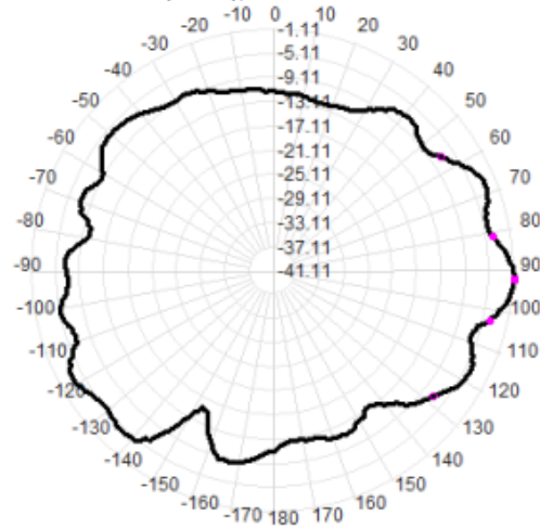
2480.0MHz Total(E2-YZ), Max=-1.23dBi
