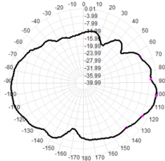
2441.0MHz Total(E2-YZ), Max= 0.01 dBi
