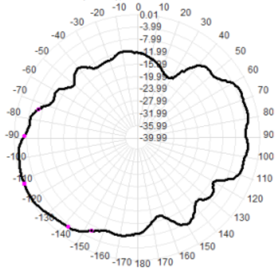
2441.0MHz Total(E1-XZ), Max=-0.34dBi
