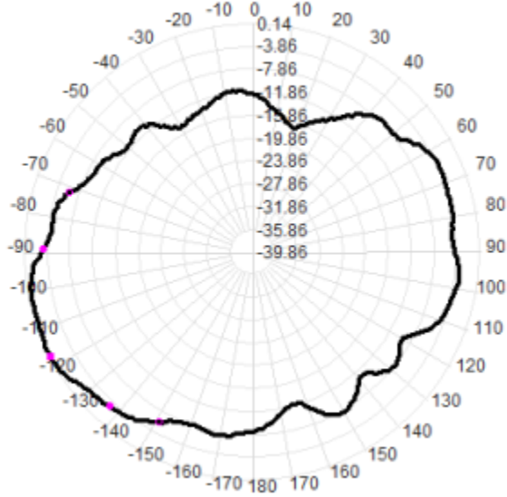
2402.0MHz Total(E1-XZ), Max=-0.05dBi
