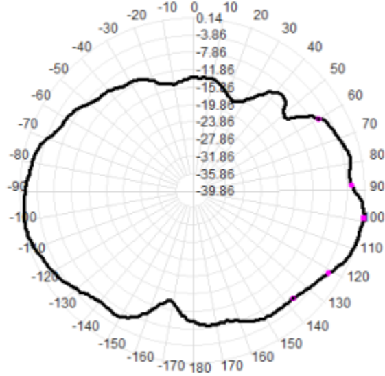
2402.0MHz Total(E2-YZ), Max= 0.14dBi
