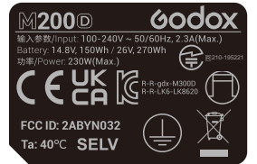
707-M200D0-02右侧贴纸 707-M200D0-02 right side sticker
