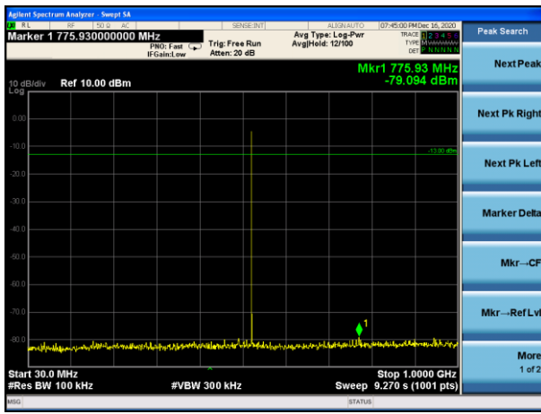
TX CH25(30MHz-1GHz)
