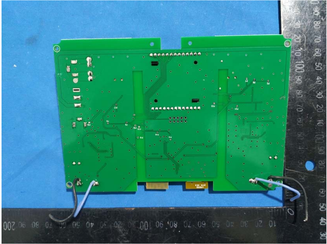
BLE Antenna
